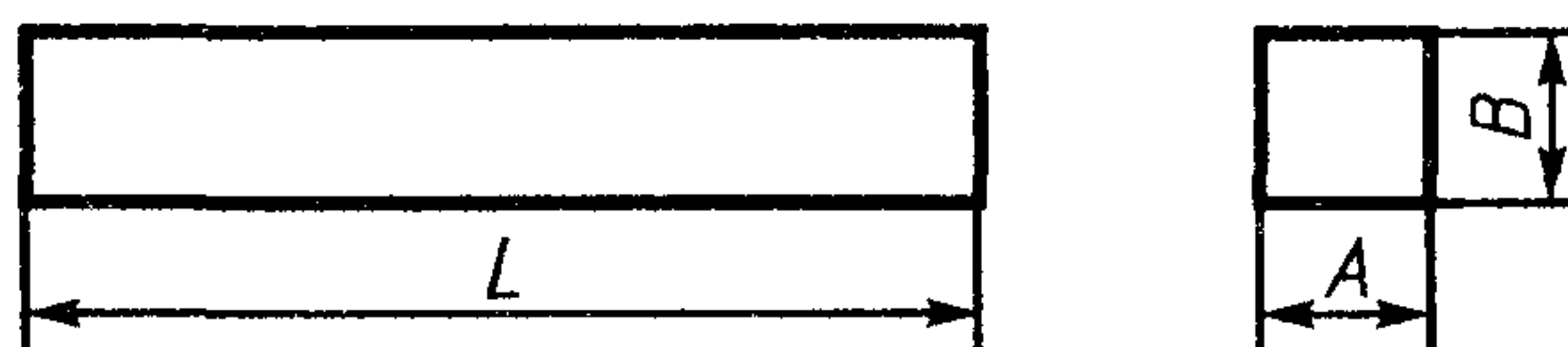
Рисунок А.1 — Размеры образца для испытания на ударный изгиб
