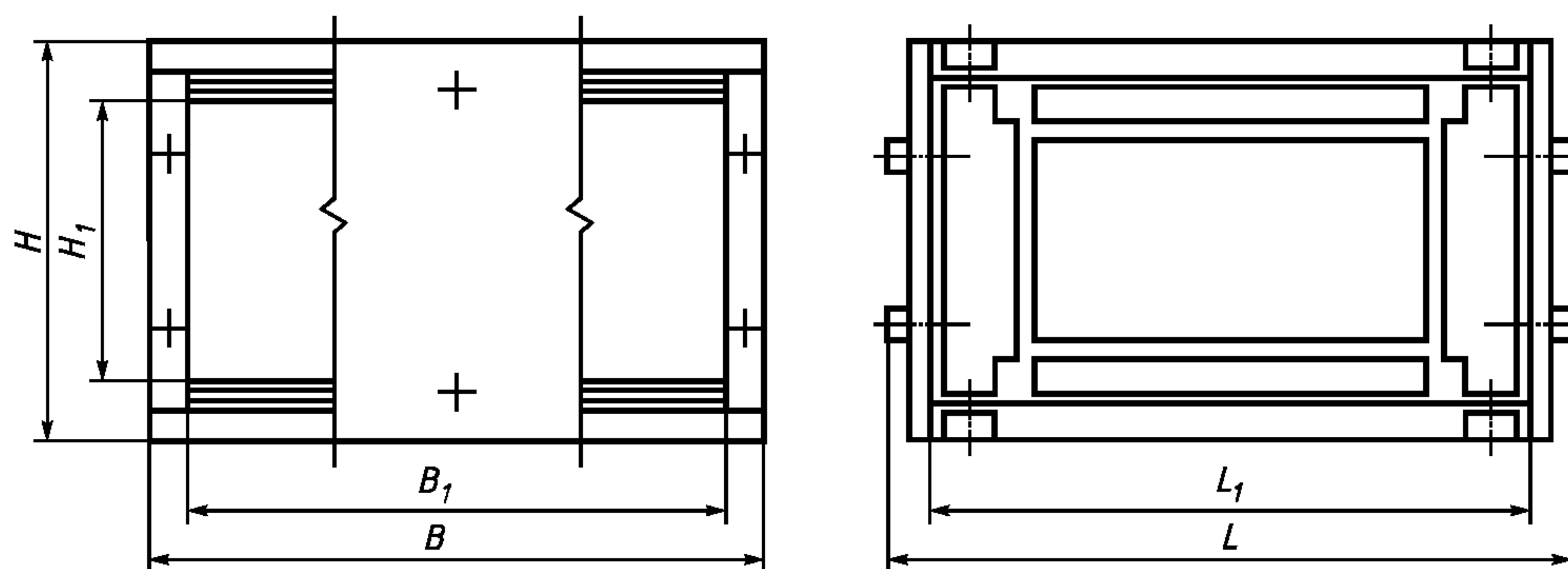
Рисунок 6 — Координационные размеры БНК3 (корпус моноблока)
