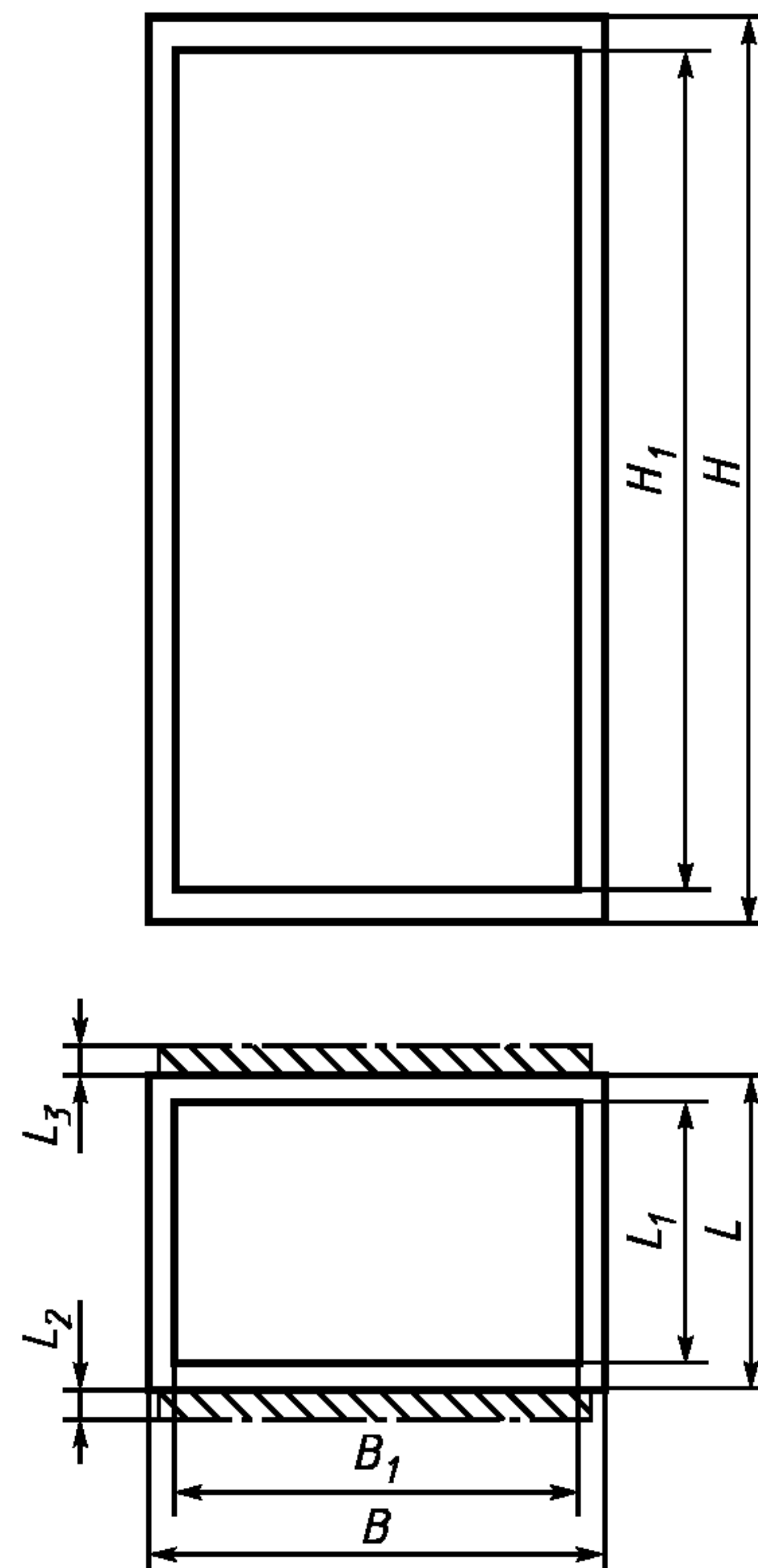
Рисунок 5 — Координационные размеры БНКЗ (корпус шкафа)
