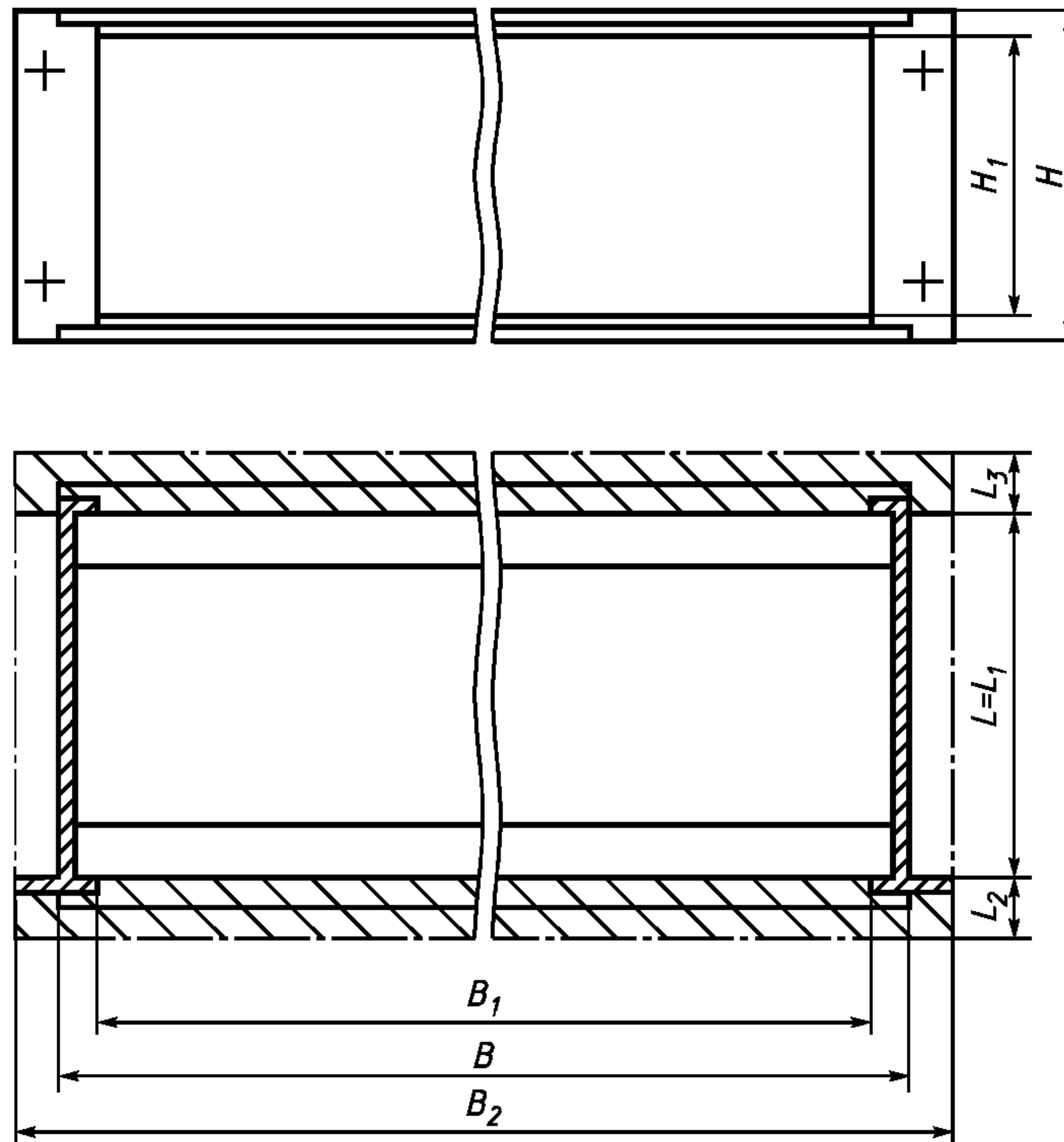
Рисунок 3 — Координационные размеры БНК2 (блочный каркас)
