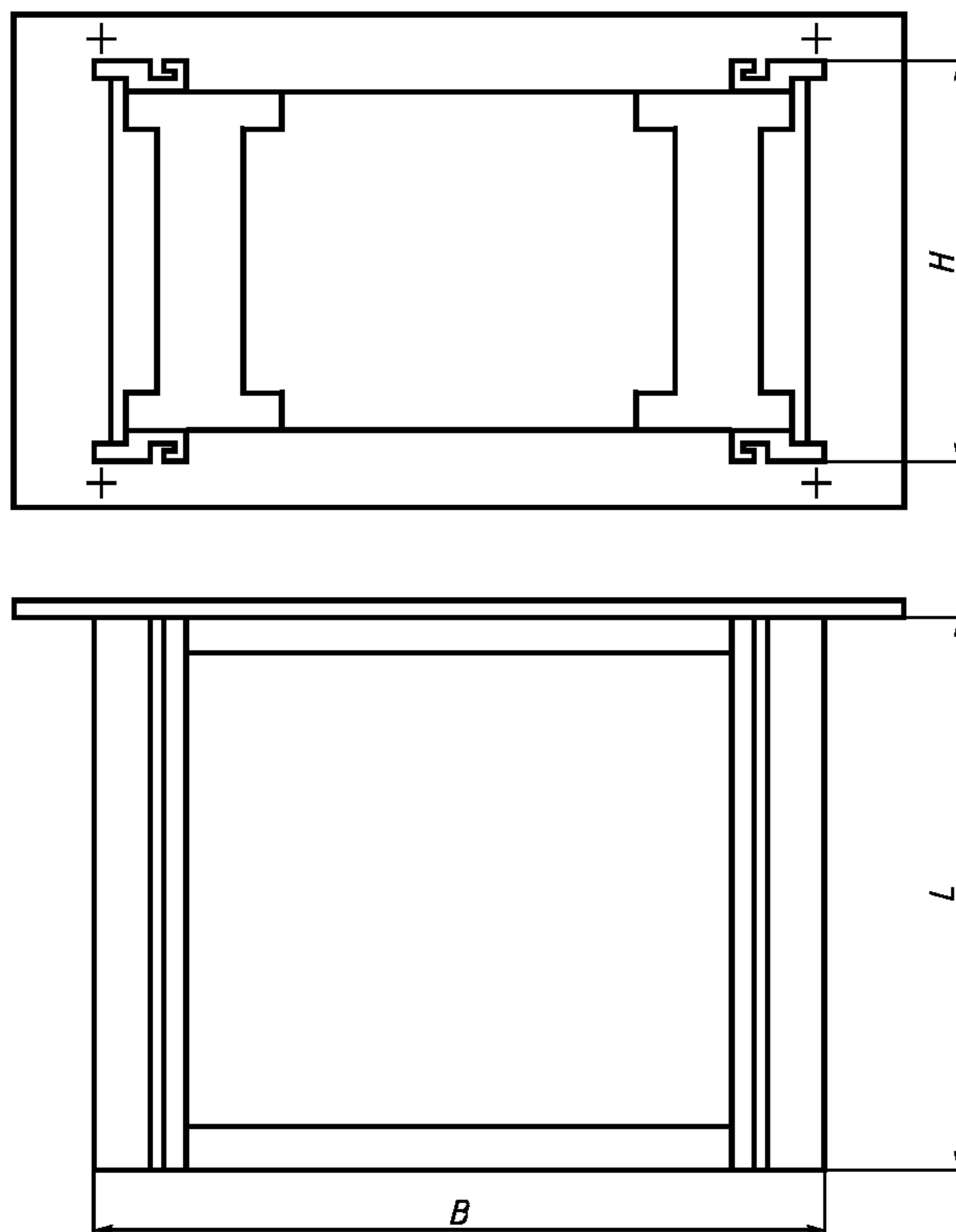
Рисунок 4 — Координационные размеры БНК2 (корпус вставного блока)
