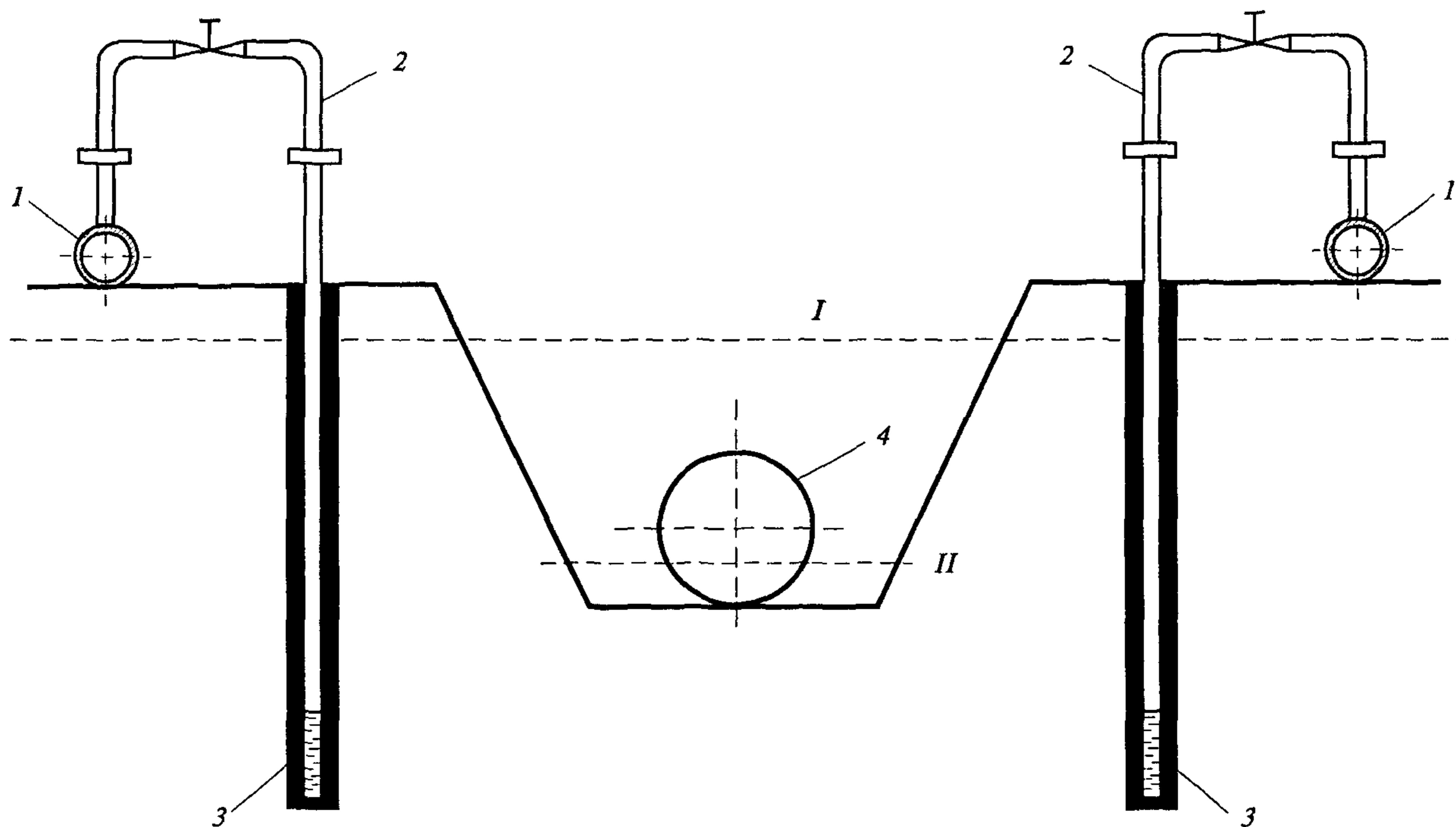
Рис. 5.5. Схема искусственного водопонижения при двух рядах иглофильтров:
