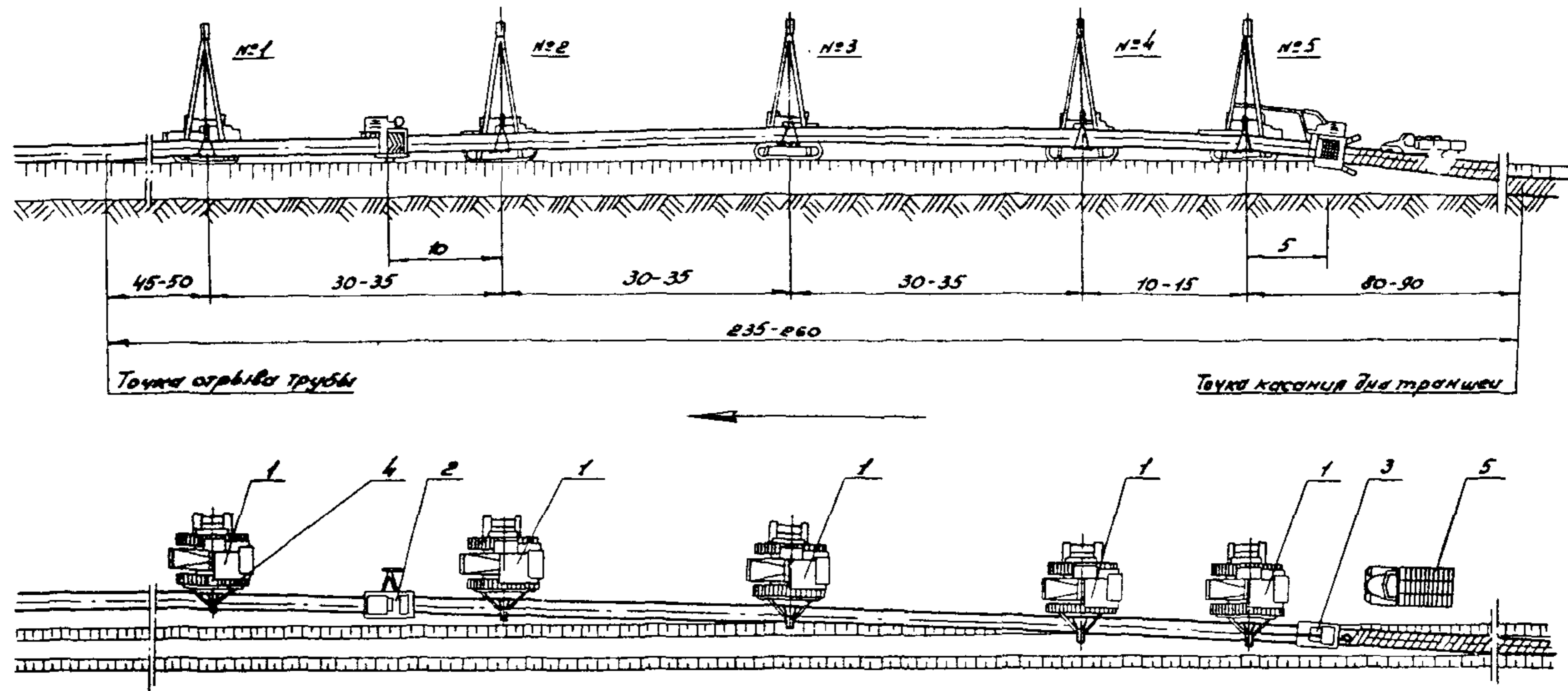
Рис. I. Расстановка машин в колонне при совмещенном способе
