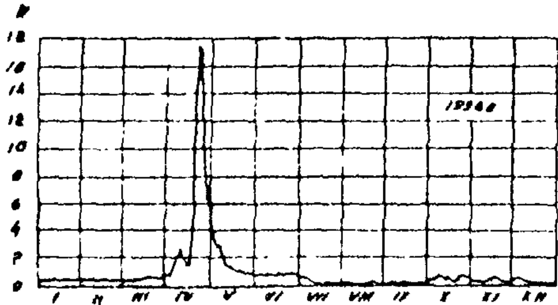
Восточноевропейский подтип режима расходов: р. Вальса - Калинин.
