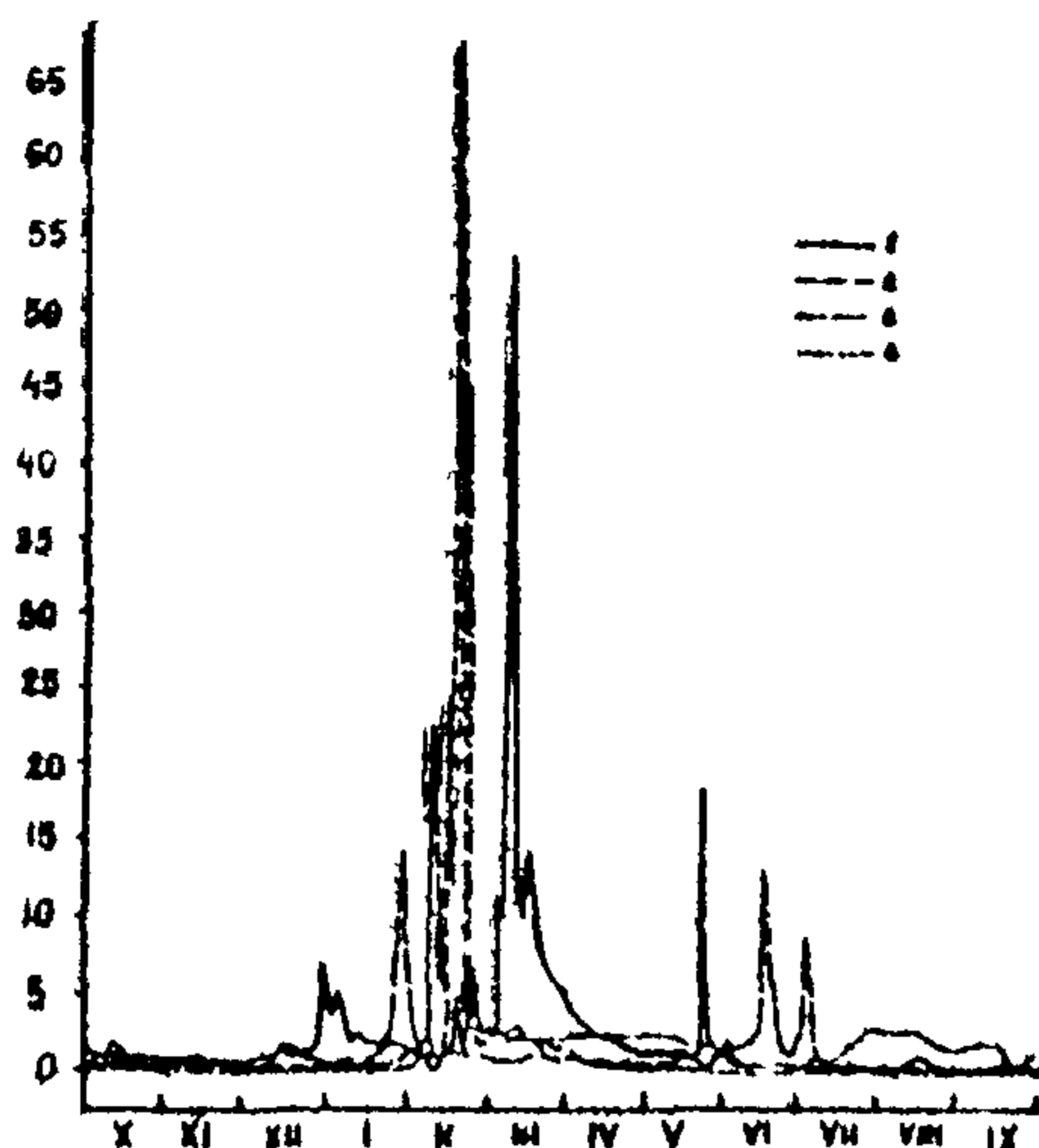
Гидрографы р. Дихая-х. Богурев. 1-гидрограф 1967-68г., 2-средний по водности 1959-60г., 3-близкий к многоводному 1957-58г., 4-близкий к мало- водному 1956-57г.
