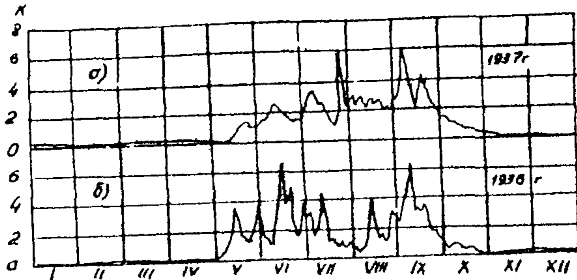
Дальневосточный тип режима расходов а) р. Витим - Бадайтба, б) р. Зея - Зейские врата.
