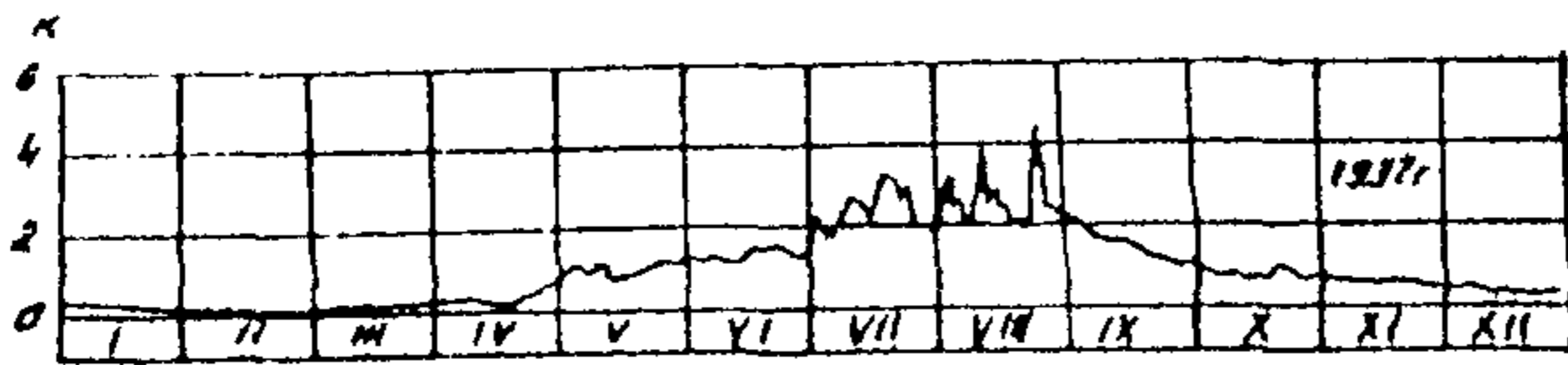
Тяньшанский подтип режима расходов р. Терек - Казбек.
