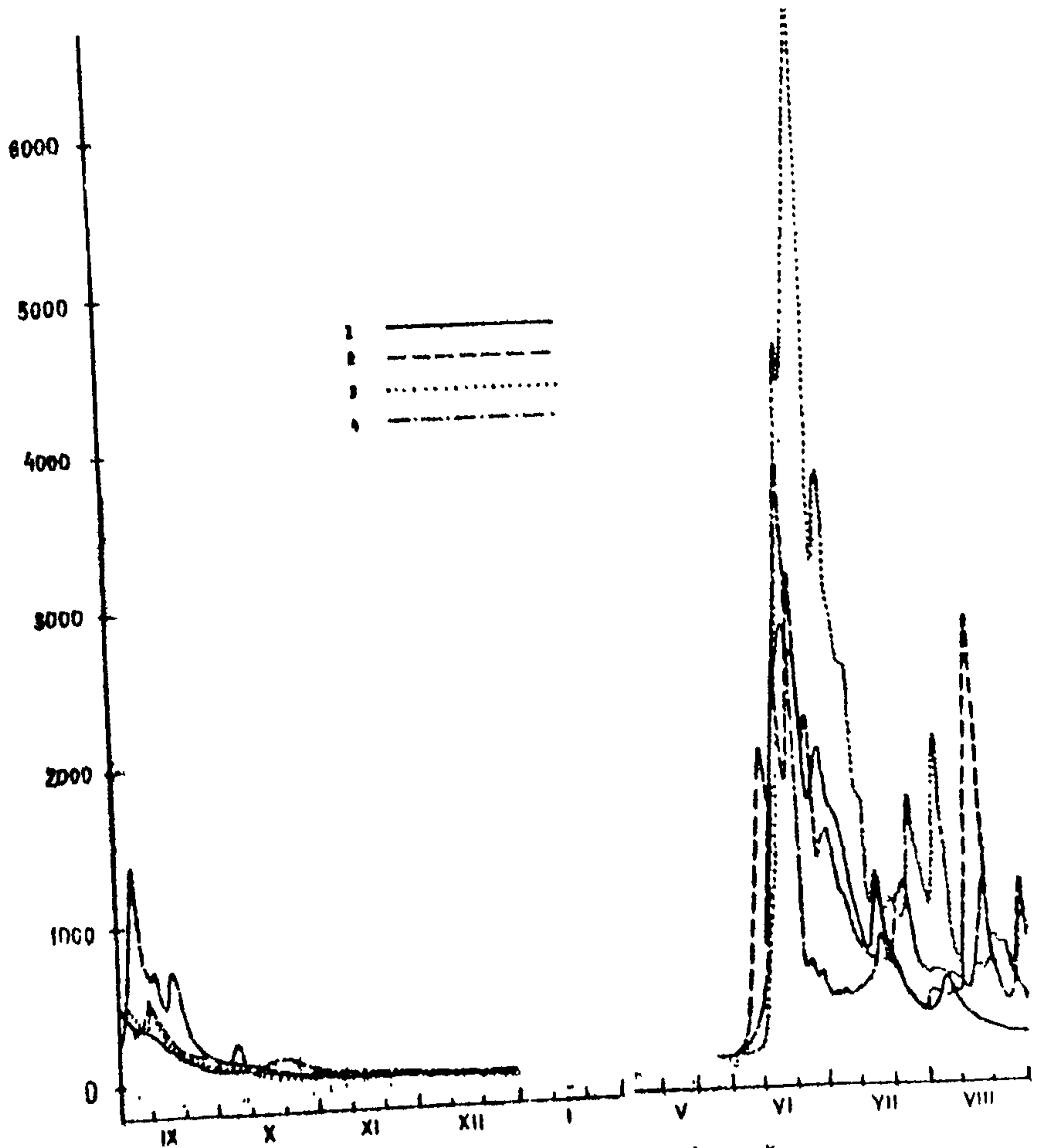
Гидрографы р. Амгузак-устье р. Куждья. 1-гидрограф 1968-69гг., 2-средний по водности 1959-60гг., 3-слизкий к многоводному 1961-62гг., 4-слизкий к маловодному 1954-55гг.
