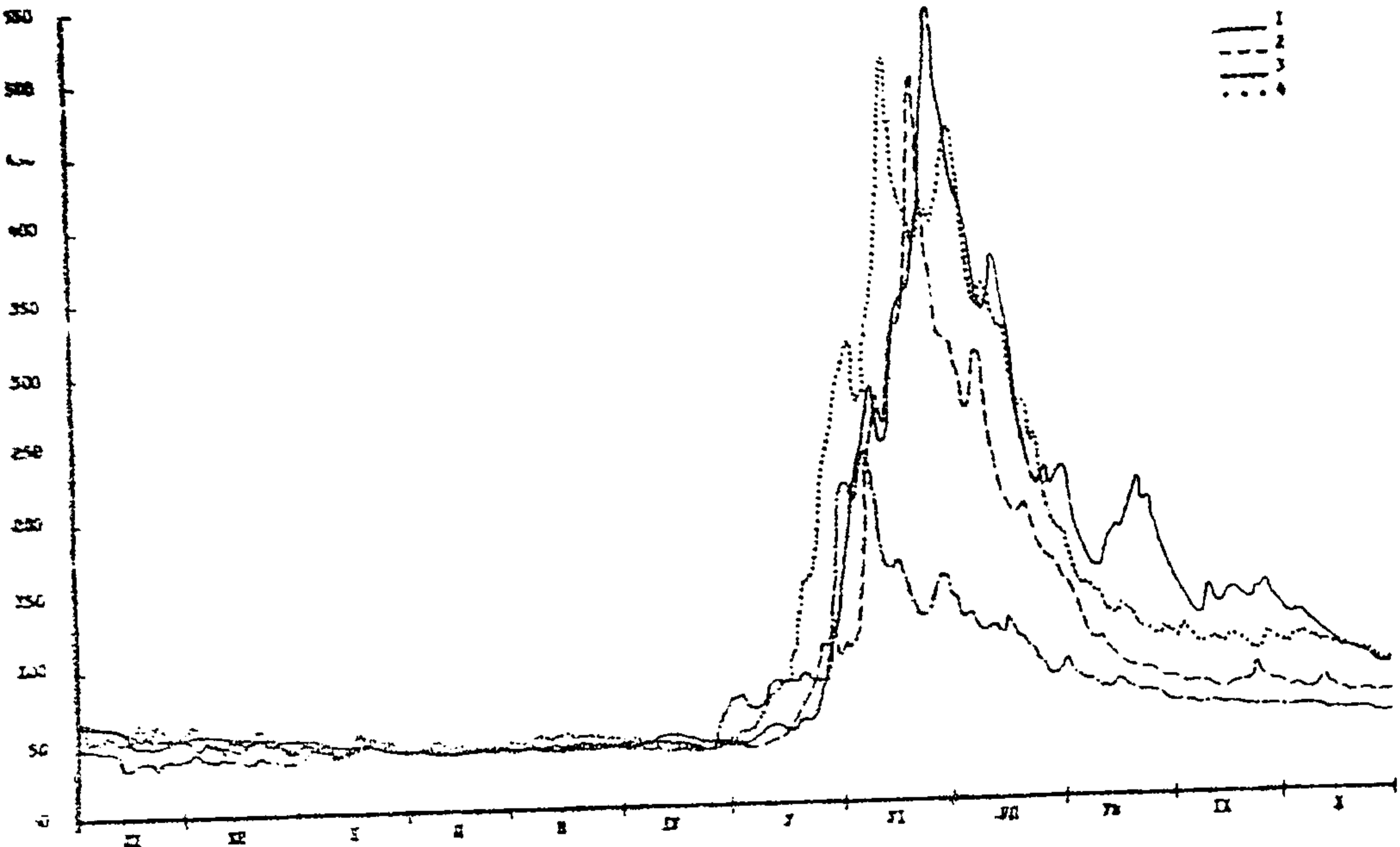
Гидрографы р. Камчатка-с. Верхне-Камчатка. 1-гидрограф 1968-69г., 2-средние по водности 1950-51г., 3-слизкий и каюводному 1956-59г., 4-слизкий и каюводному 1942-43г.
