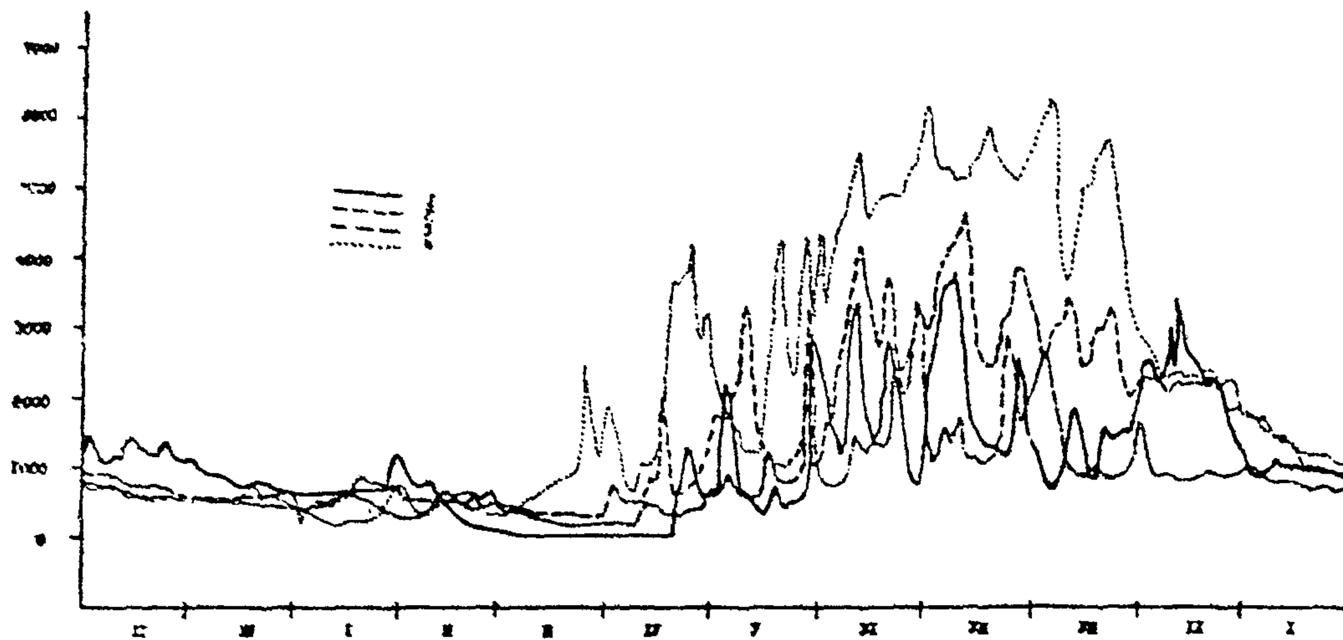
Бассейн р. Аму-Дарья. Гидрографы р. Аму-Дарья-книд. Чэтин. 1-гидрограф 1965-70г., 2-средний по водности 1958-59г., 3-близкий к маловодному 1964-65г., 4-близкий к многоводному 1968-69г.
