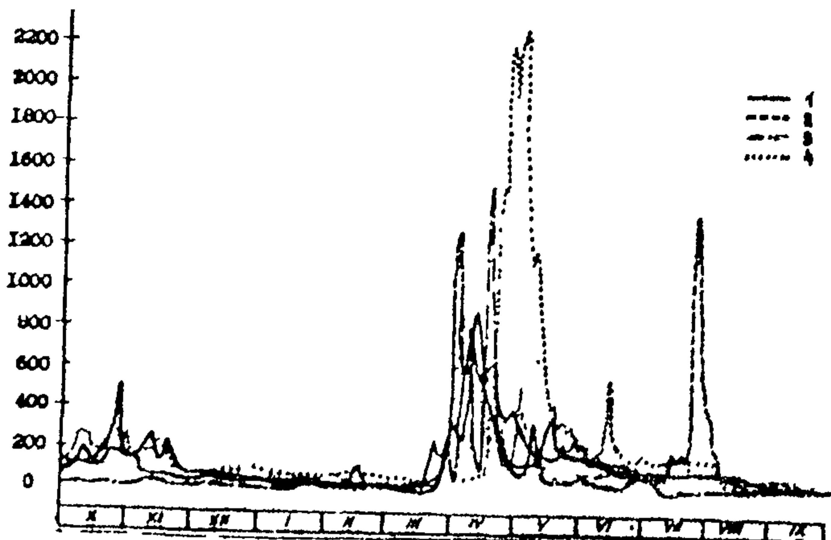
Гидрографы р. Волги-г. Старица. 1-гидрограф 1971-1972г., 2-средний по водности 1942-43гг., 3-близкий к маловодному 1938-1939гг. 4-близкий к многоводному 1954-55гг.
