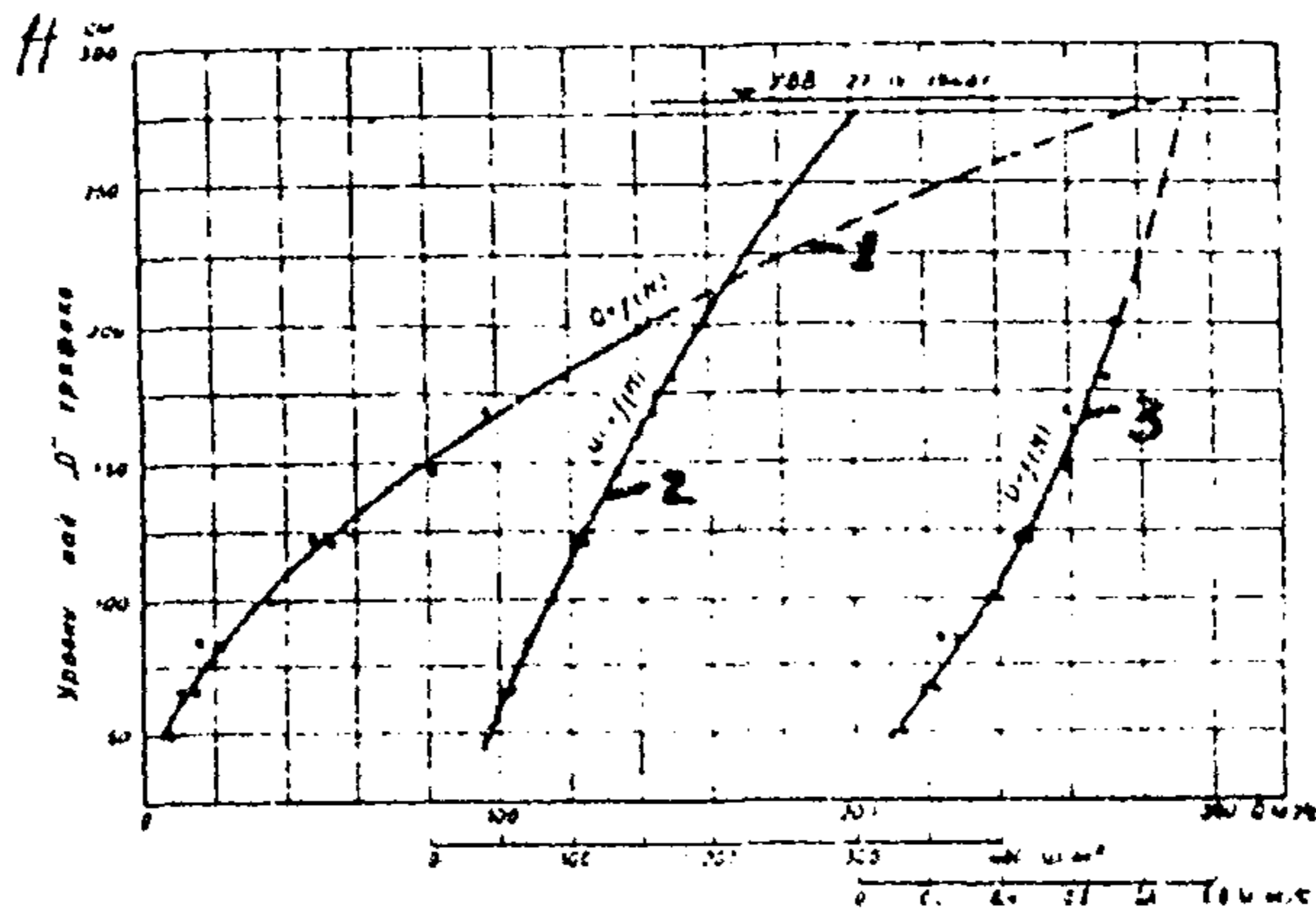
Рис.4. Морфометрические кривые зависимостей расходов /1/, площадей живых сечений /2/ и скоростей течения /3/ от уровня воды в створе моста.
