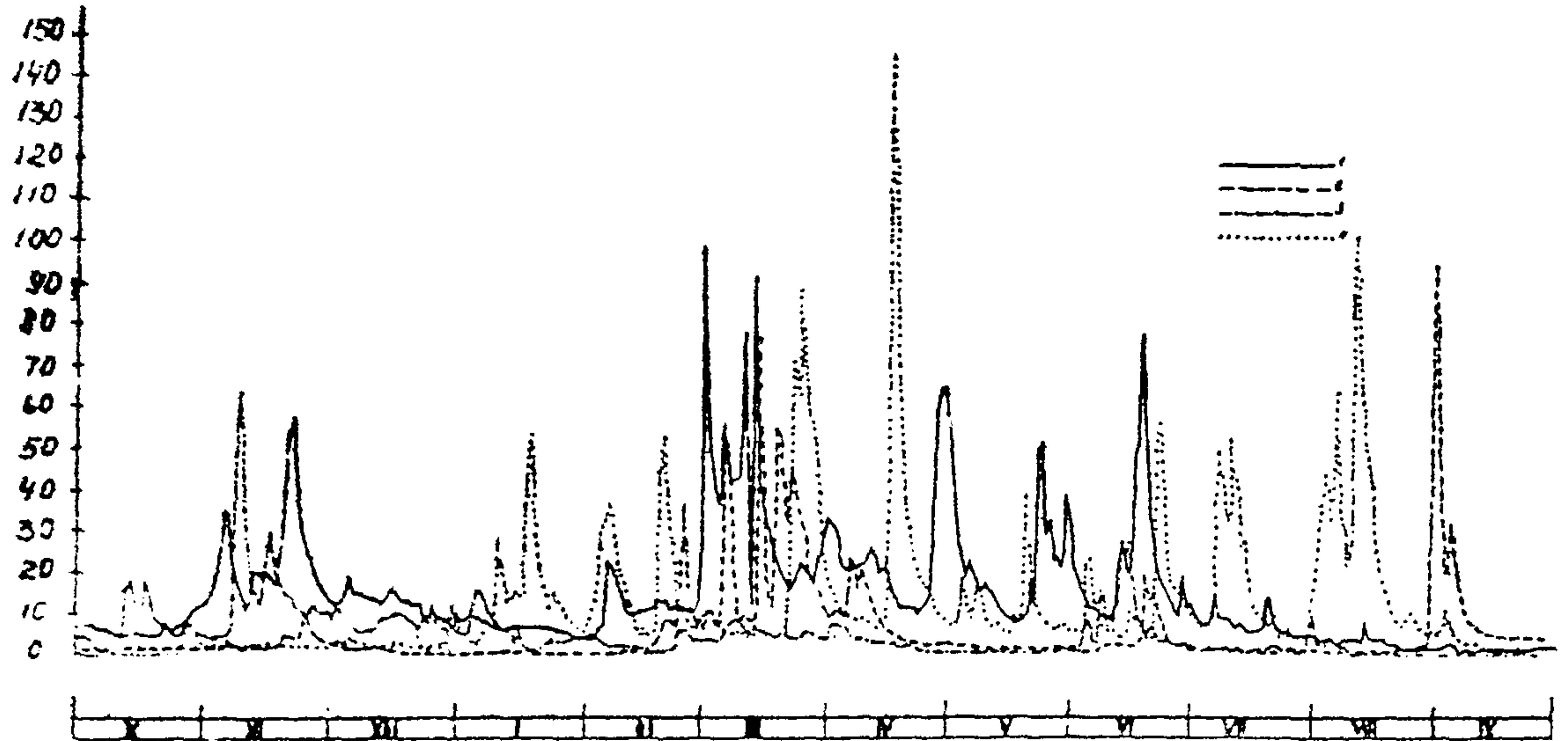
Гидрографы р. Днестр-г. Самбор. 1-гидрограф 1966-67г., 2-средний по водности 1946-47г., 3-близкий к маловодному 1960-61г., 4-близкий к многоводному 1954-55г.
