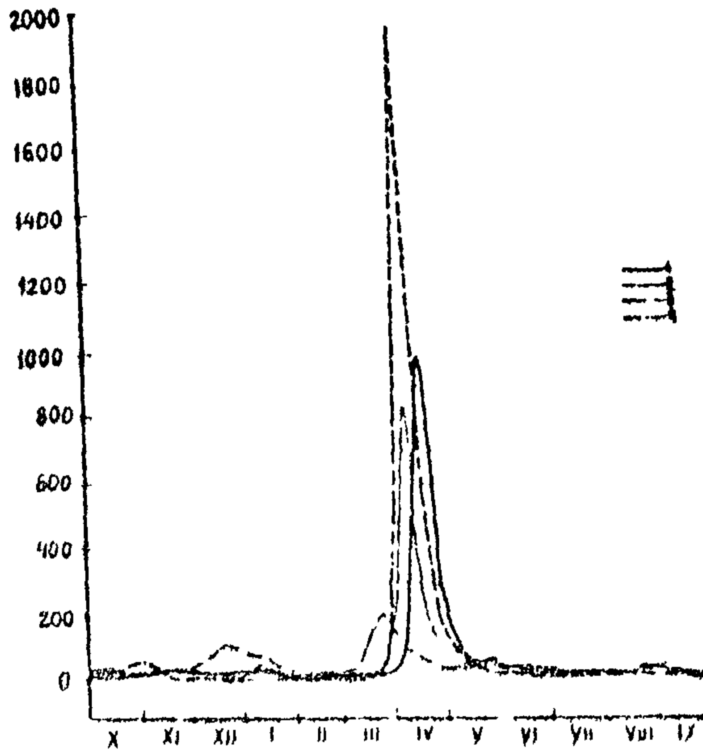
Гидрографы р.Сены-г.Рылов. 1-гидрограф 1958-59гг., 2-средний по водности 1944-45гг., 3-близкий к маловодному 1920-21гг., 4-близкий к многоводному 1969-70гг.
