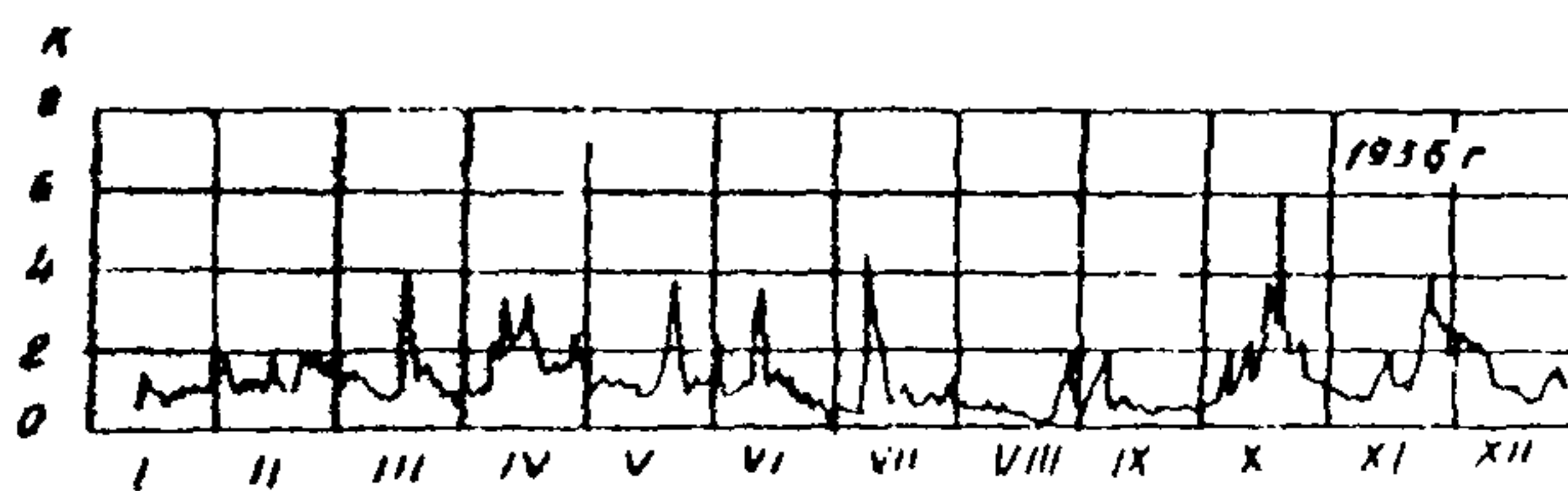
Причерноморский подтип режима расходов р. Сочи - Пластунка
