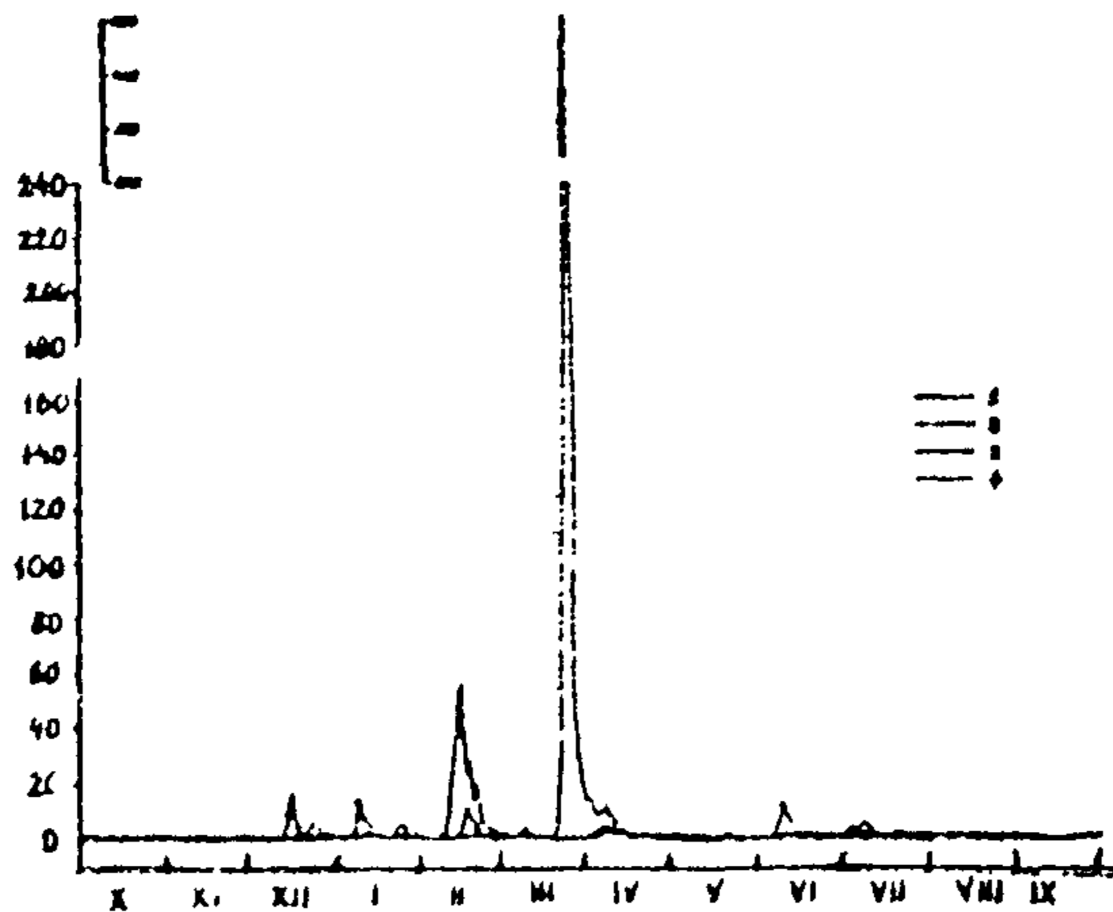
Гидрографы р. Самара-с. Кухановка. 1-гидрограф 1968-69г., 2-средний по водности 1957-58г., 3-близкий к маловодному 1961-62г., 4-близкий к много- водному 1963-64г.
