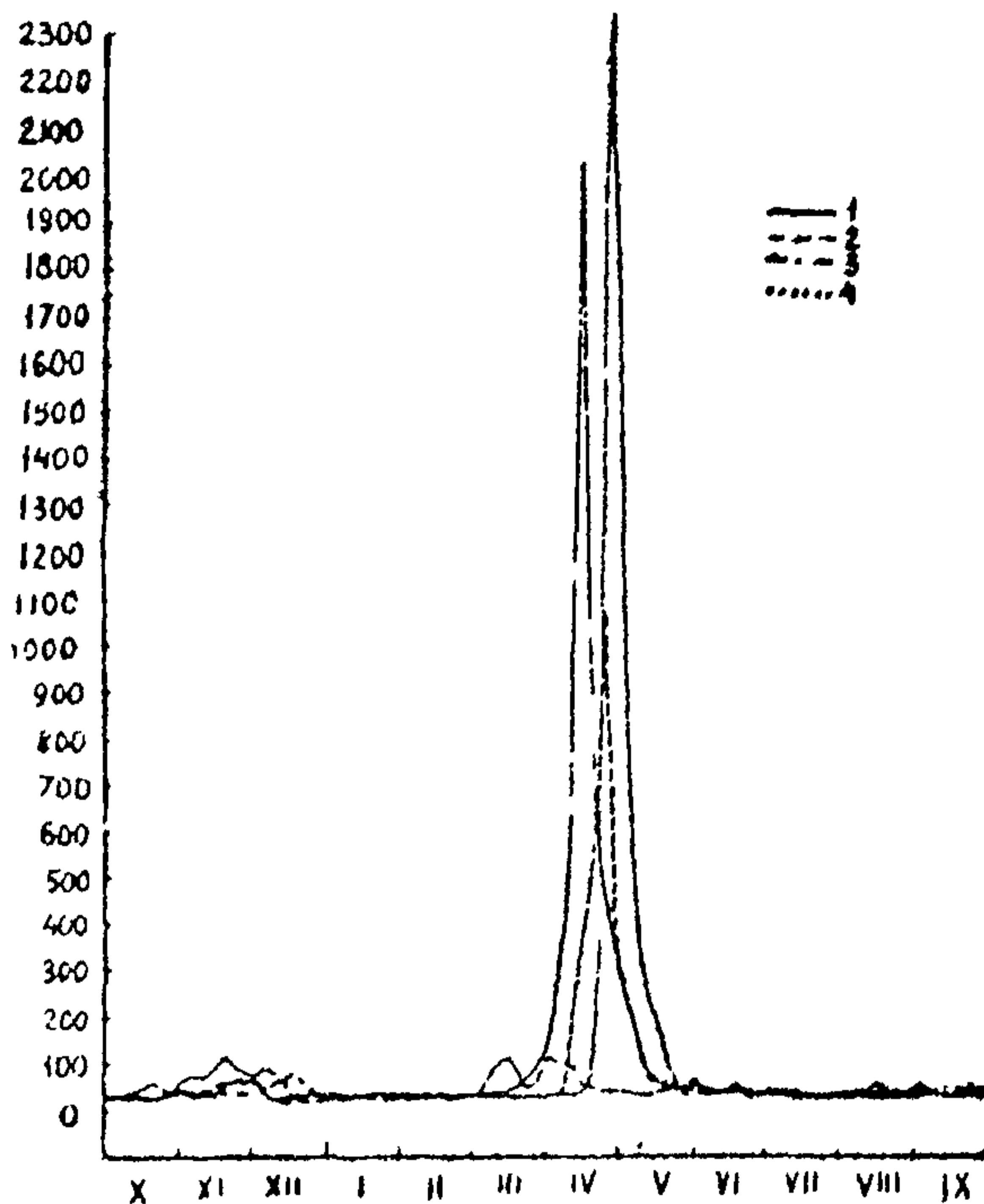
Гидрографы р. Десна-г. Брянск. 1-гидрограф 1966-67гг., 2-средний по водности 1964-1965гг., 3-близкий к маловодному 1924-25гг., 4-близкий к многоводному 1930-31гг.
