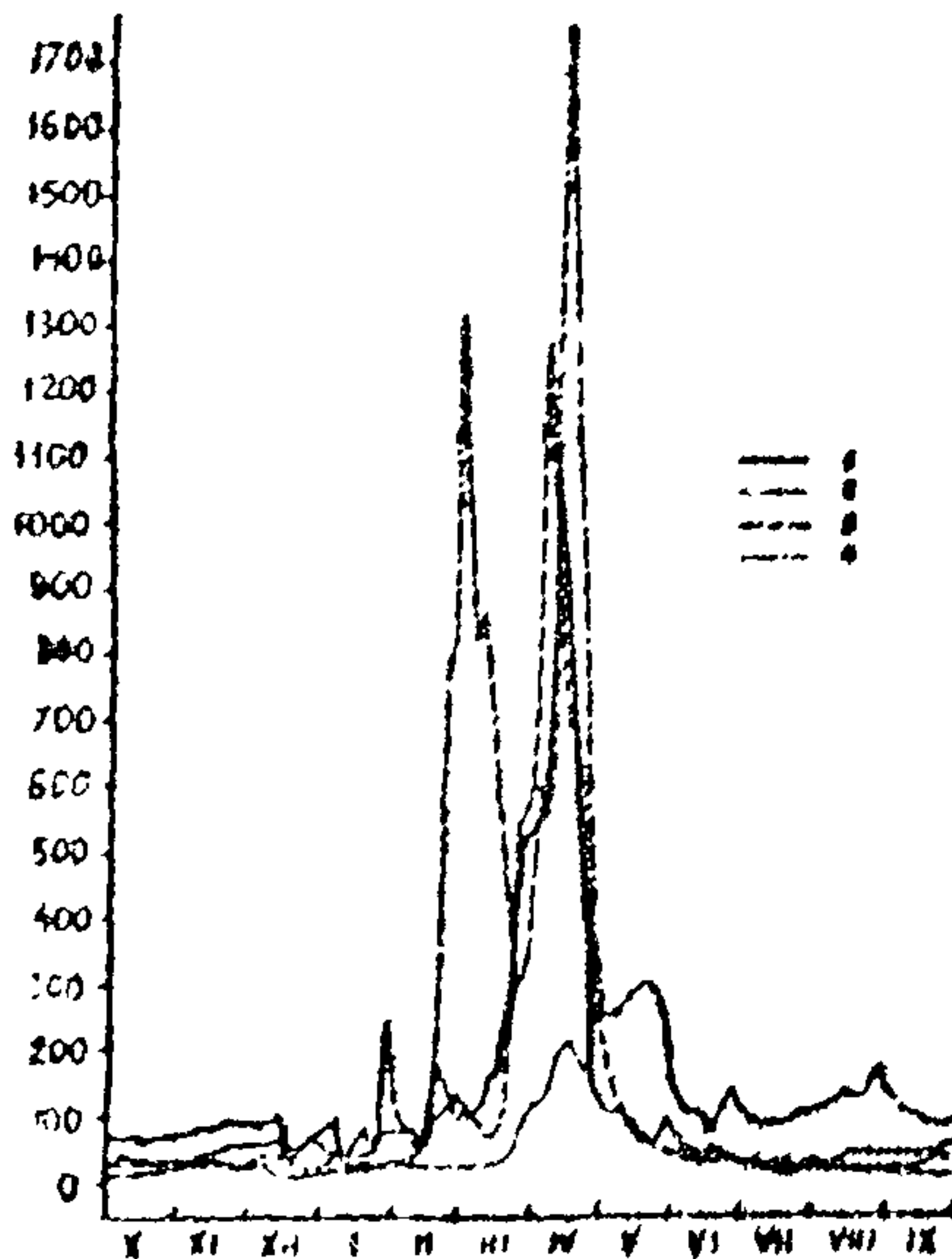
Гидрографы р. Северский Донец-г. Лисичанок. 1-гидрограф 1967-68г., 2-средний по водности 1988-89г., 3-близкий к многоводному 1940-41г., 4-близкий к мало- водному 1953-54г.
