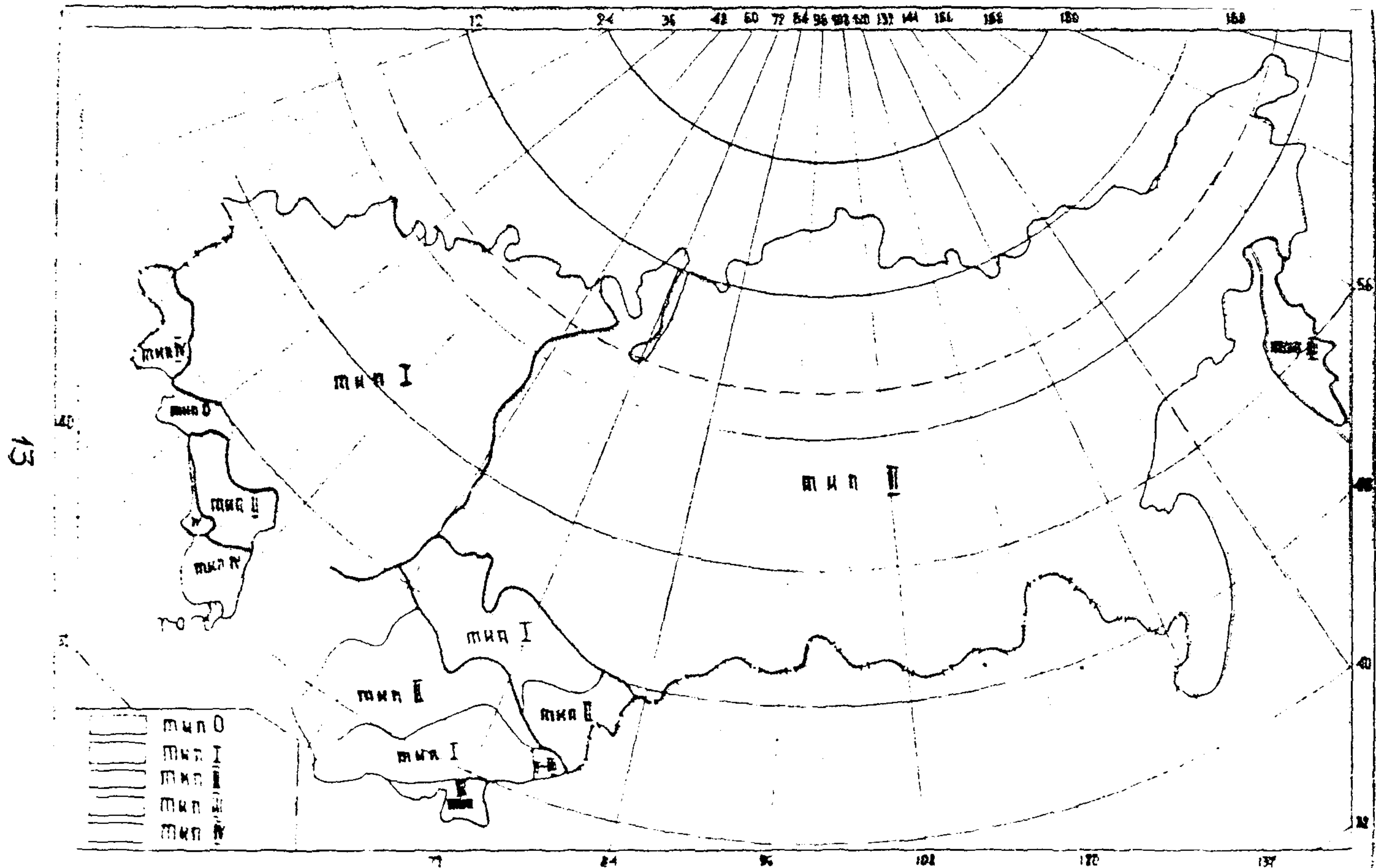
Рис 2 Карта-схема гидрологического районирования типов внутригодового распределения стока СССР (мья I)
