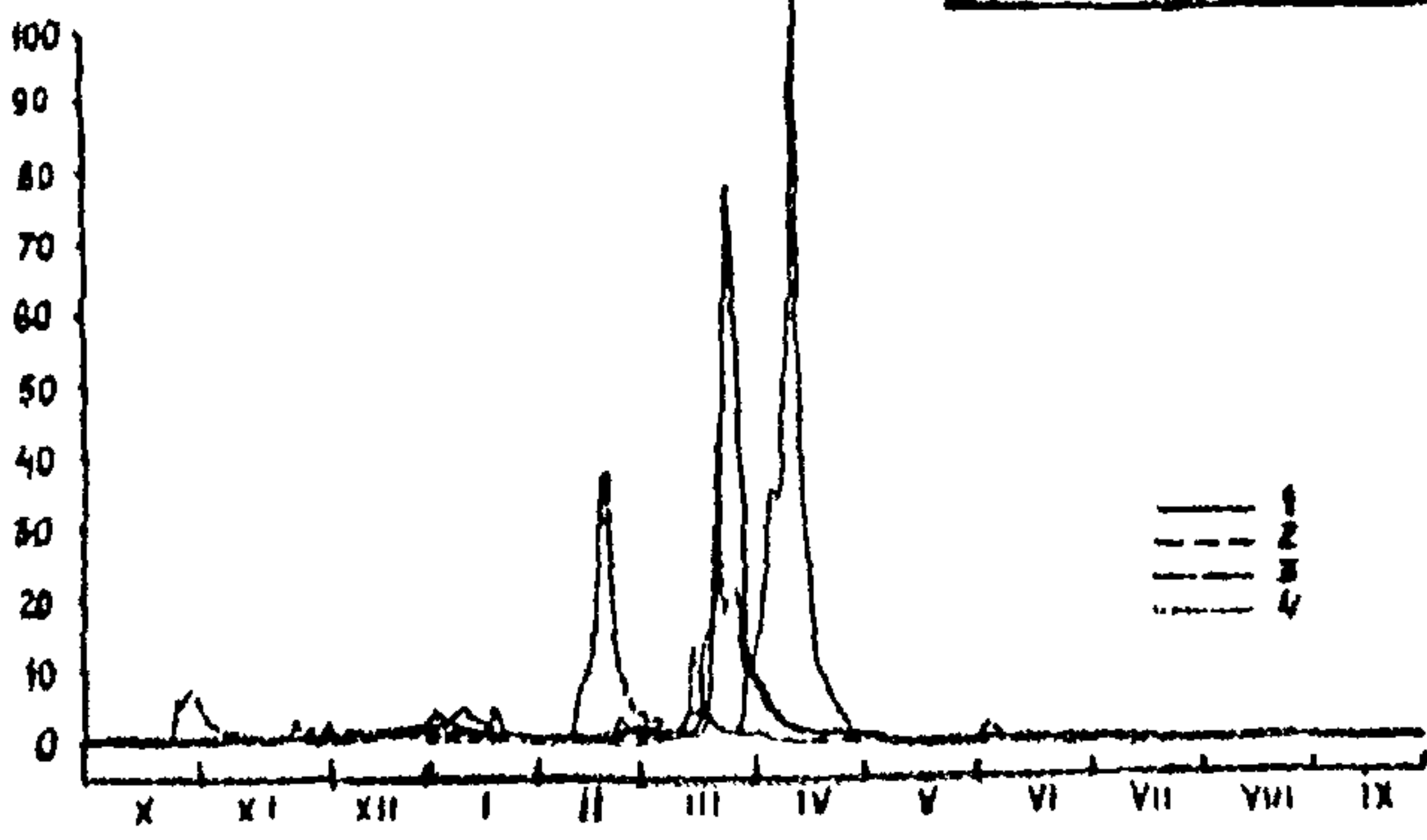
Гидрографы р. Оршик-о. Чернушина. 1-гидрограф 1967-68г., 2-средний по водности 1956-57г., 3-близкий к маловодному 1960-61г., 4-близкий к много- водному 1962-68г.
