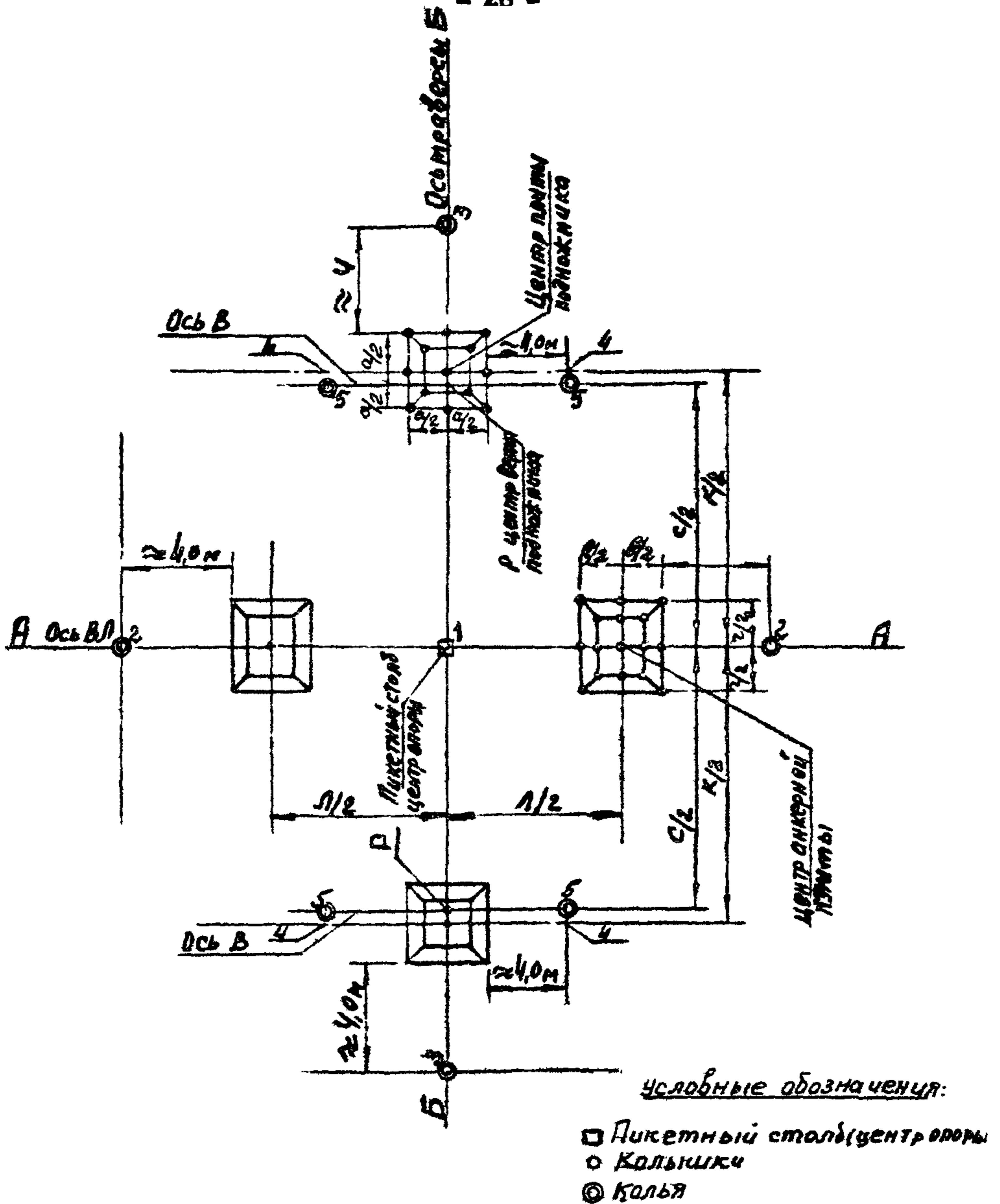
Рис. 7 Разбивка котлованов для фундаментов унифицированных промежуточных стальных опор на оттяжках ВЛ-500кВ (типов ПБ1, ПБ2, ПБ3, ПБ4 и ПБ5)
