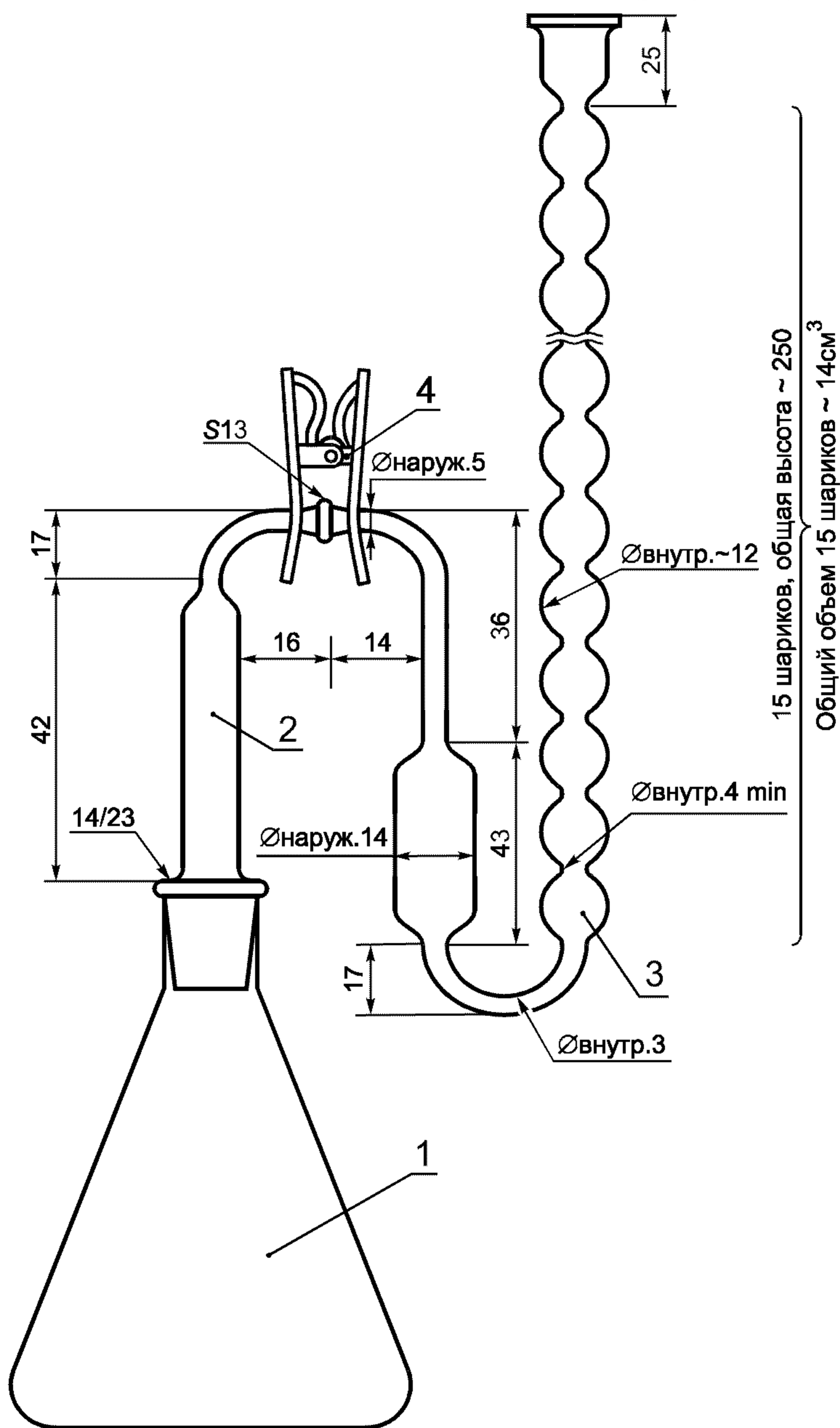
1 — реакционный сосуд; 2 — соединительная трубка; 3 — абсорбционный сосуд; 4 — предохранительные зажимы
