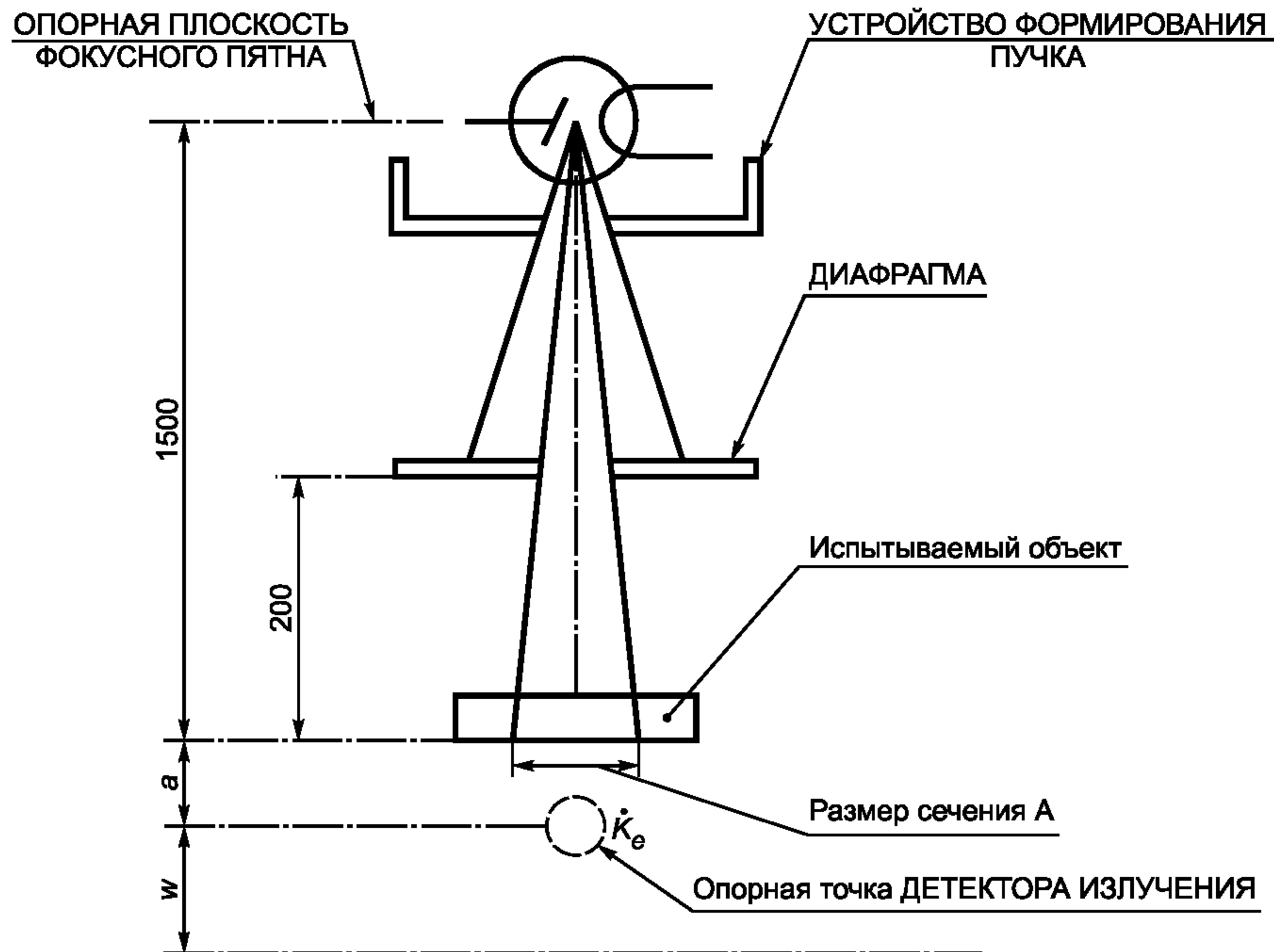
Рисунок 2 — Геометрия УЗКОГО ПУЧКА
