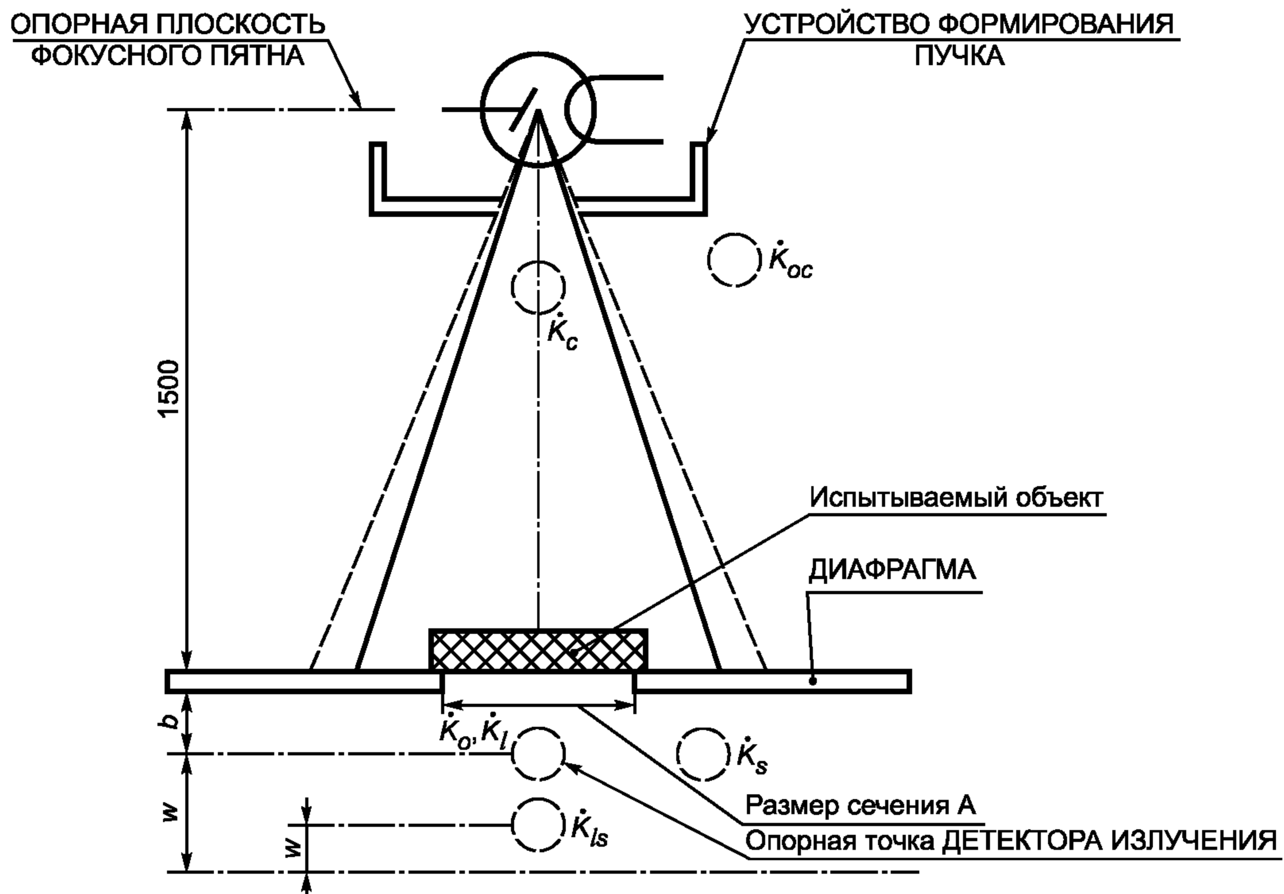
Рисунок 1 — Геометрия ШИРОКОГО ПУЧКА
