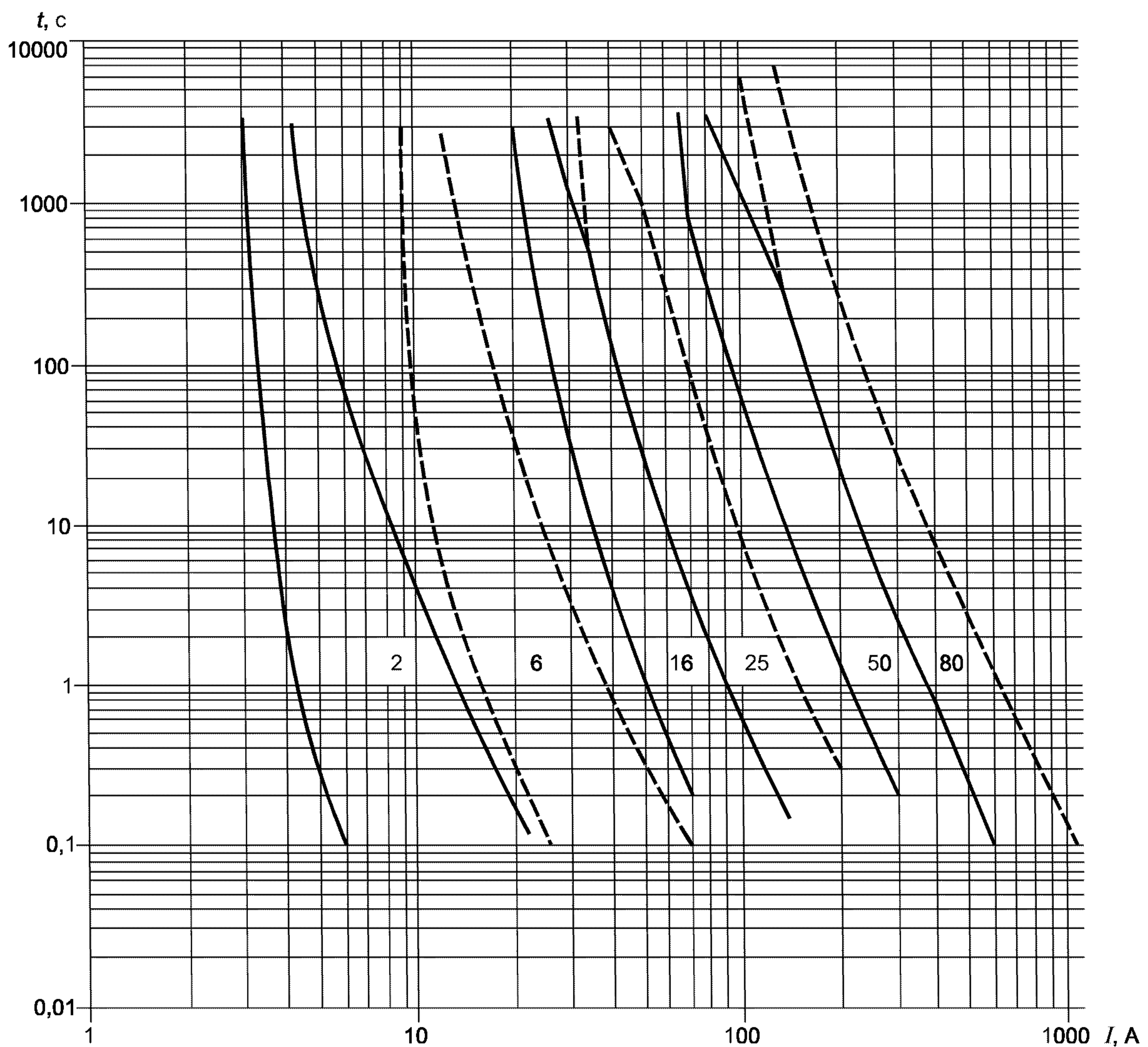
Рисунок А.1 — Время-токовые зоны для плавкого предохранителя
