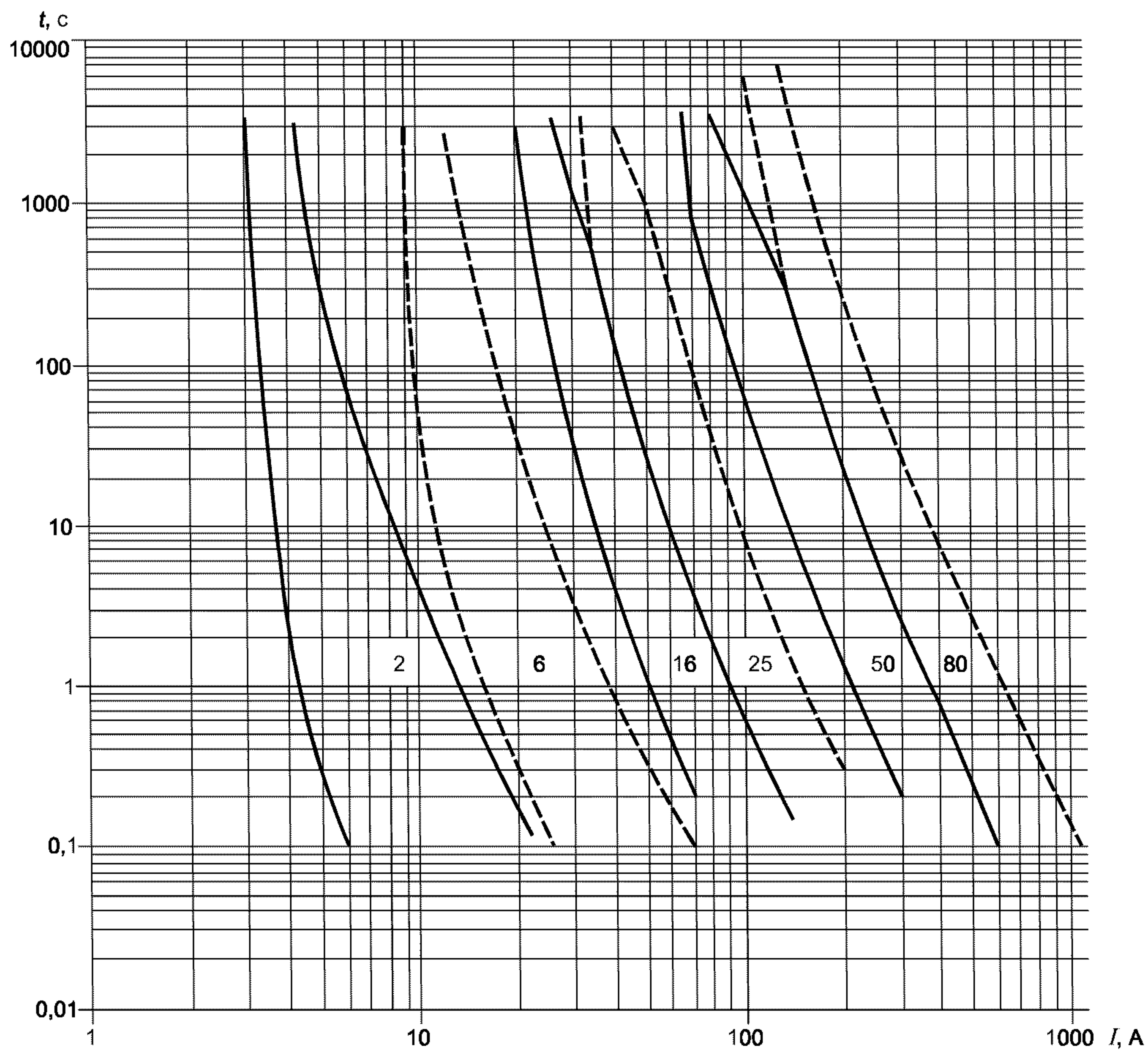
Рисунок А.1 — Время-токовые зоны для плавкого предохранителя
