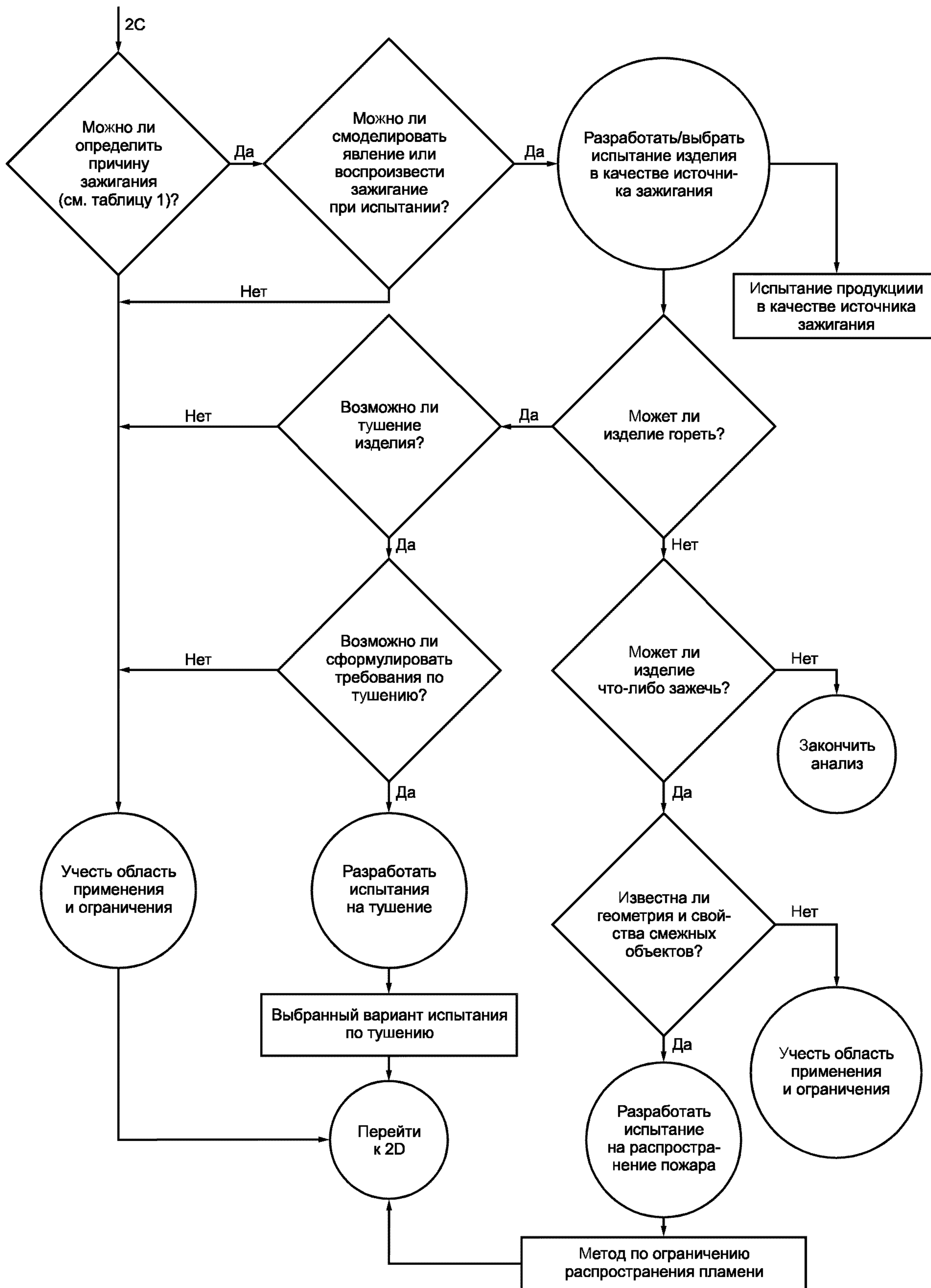
Рисунок А.5 — Блок-схема 2С. Причина пожара
