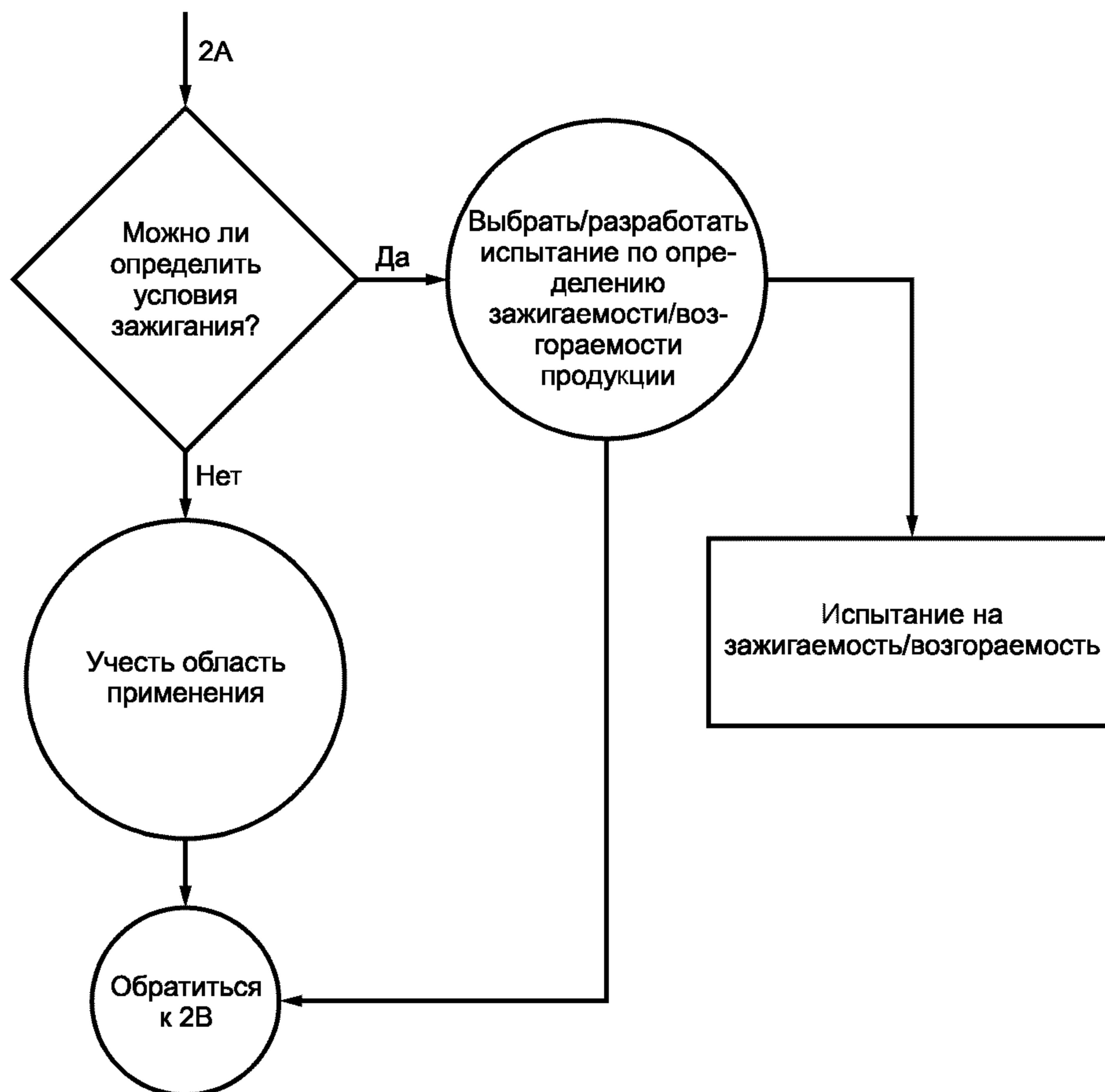
Рисунок А.3 — Блок-схема 2А. Зажигаемость/возгораемость
