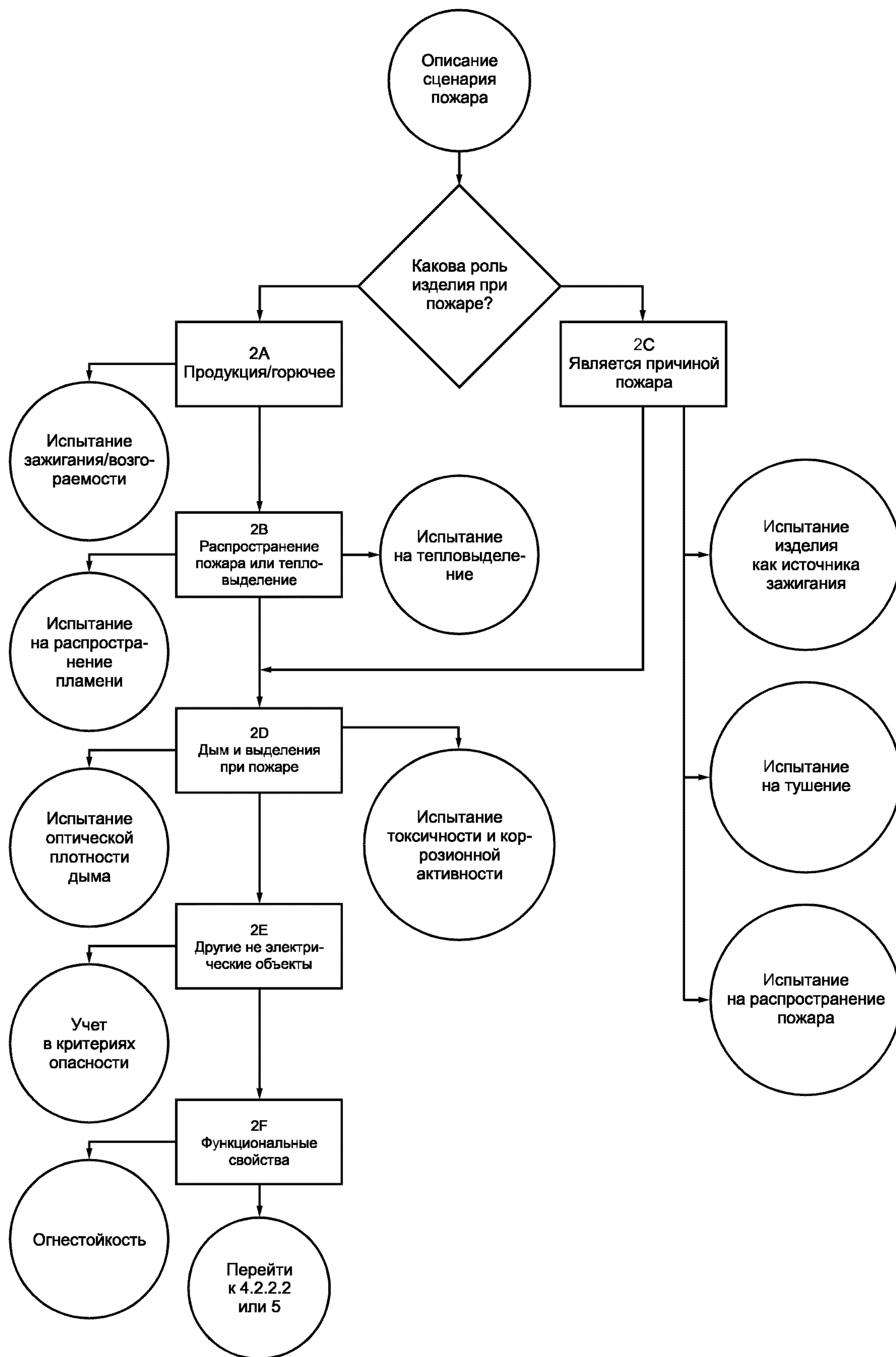
Рисунок А.2 — Блок-схема 2. Описание сценария пожара
