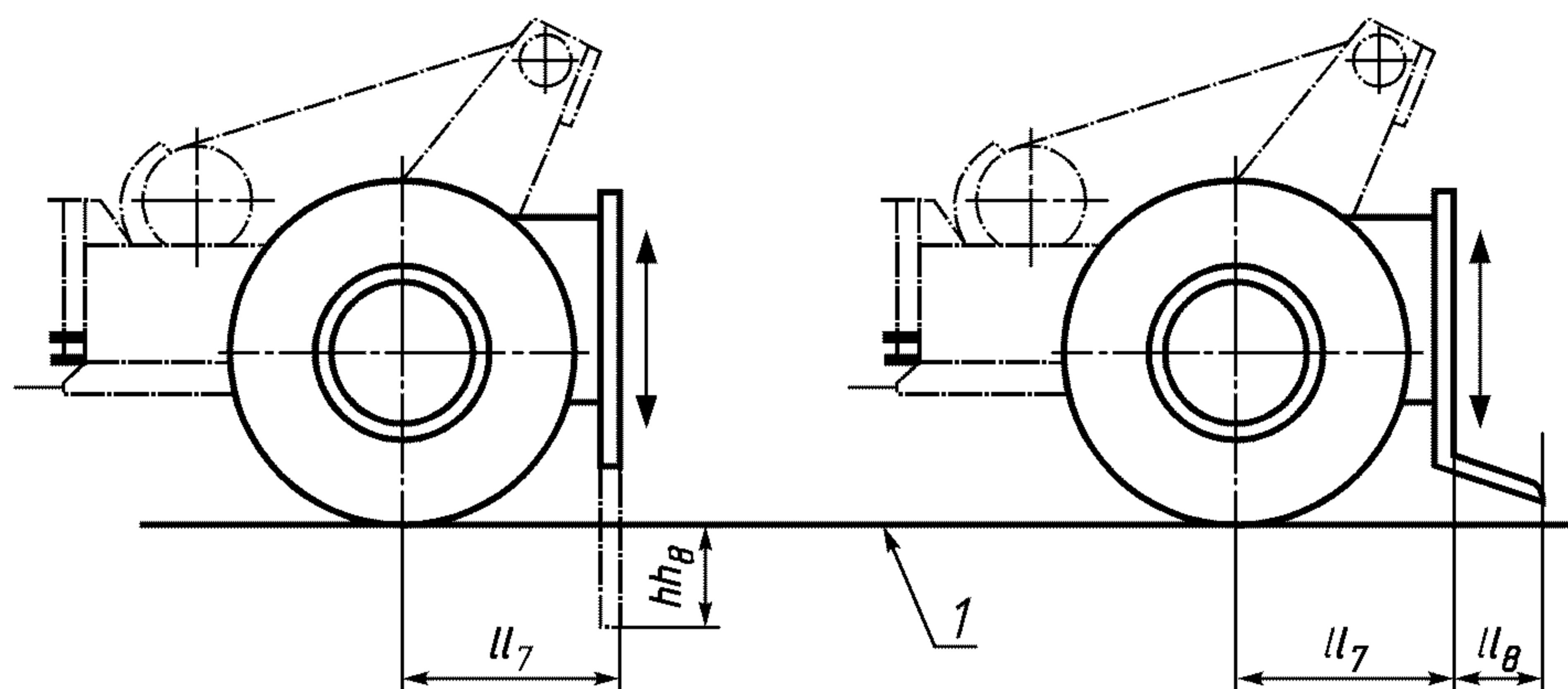
Рисунок 5 — Конструктивные параметры захвата
