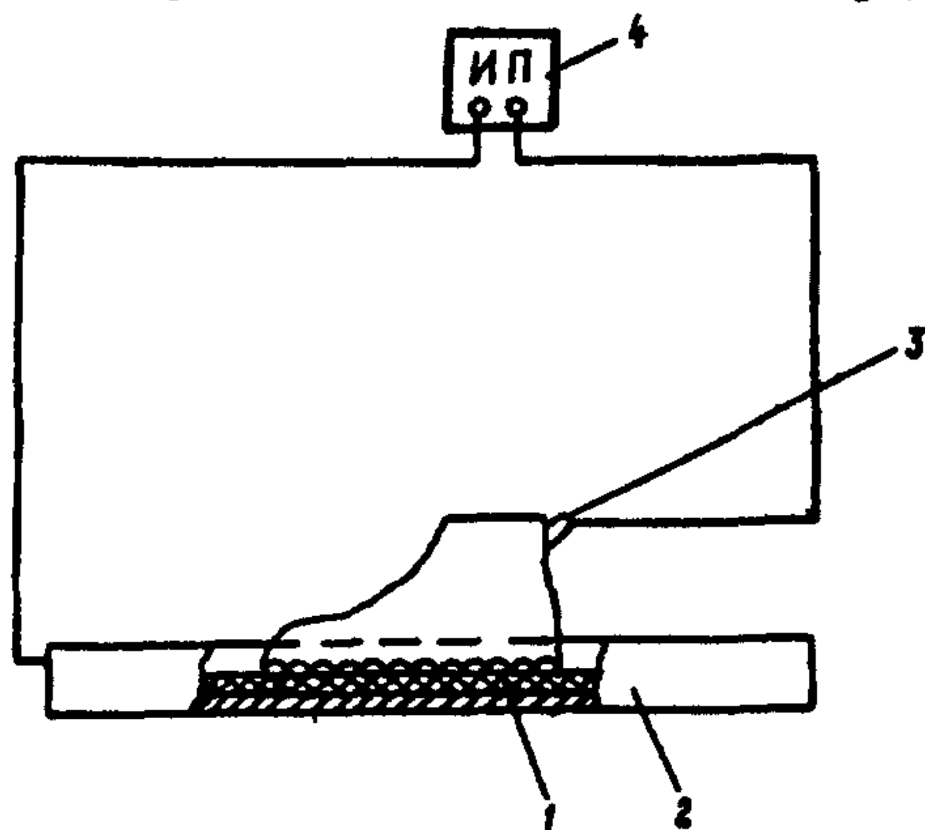
Схема измерения электрического сопротивления электропроводящей спецобуви
