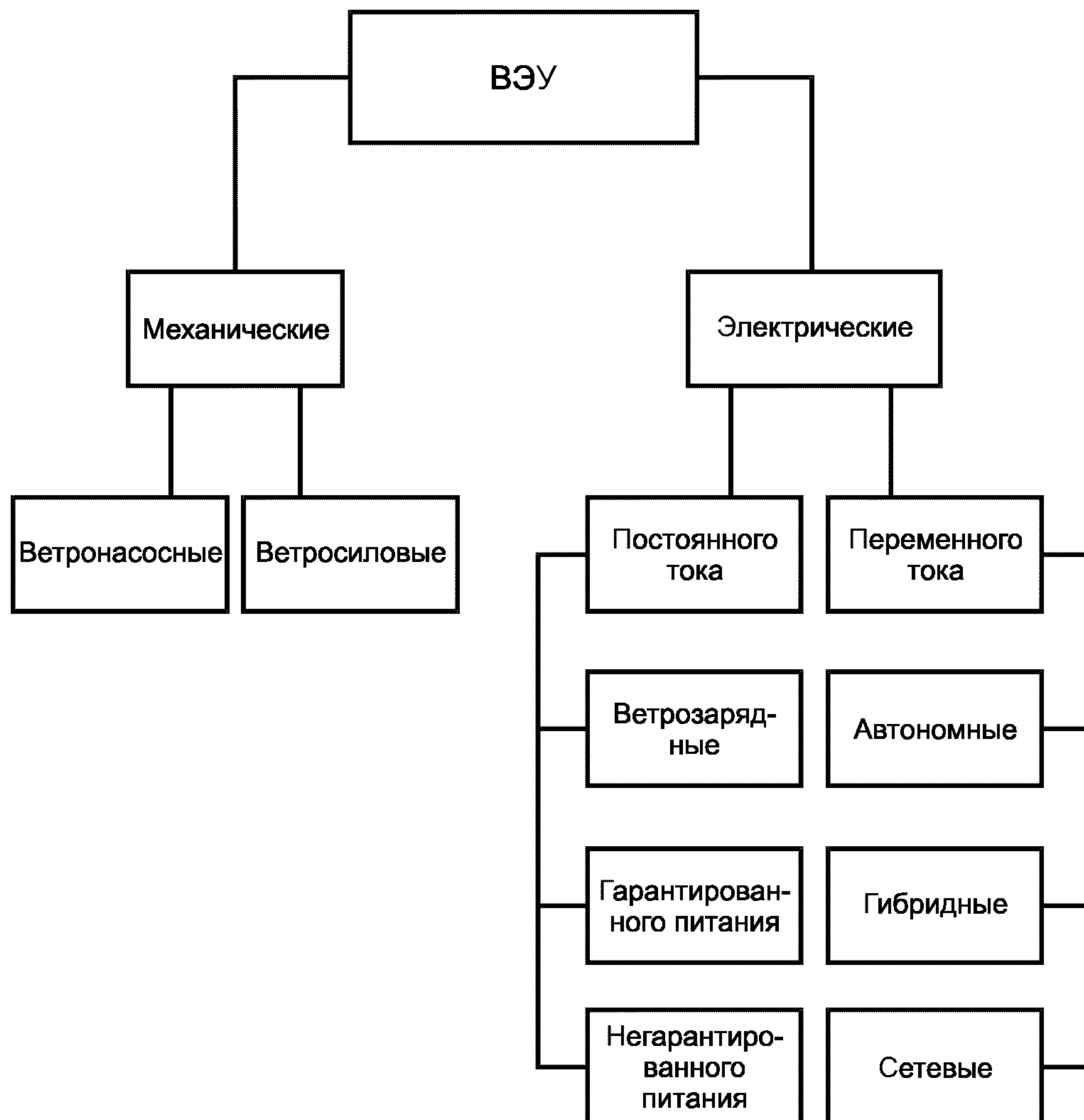
Рисунок 1 — Общая классификация ВЭУ
