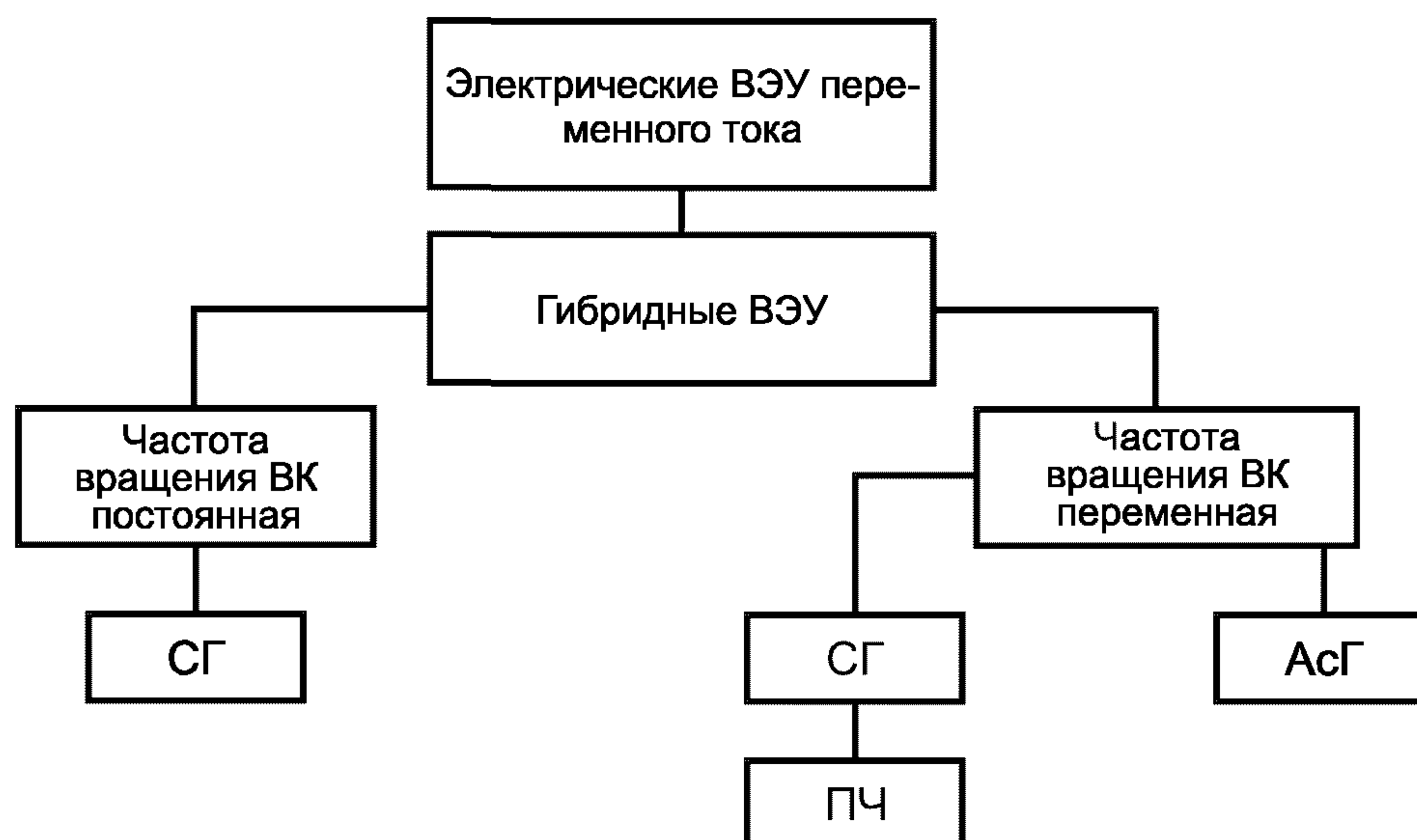
Рисунок 2 — Структурная схема автономных ВЭУ
