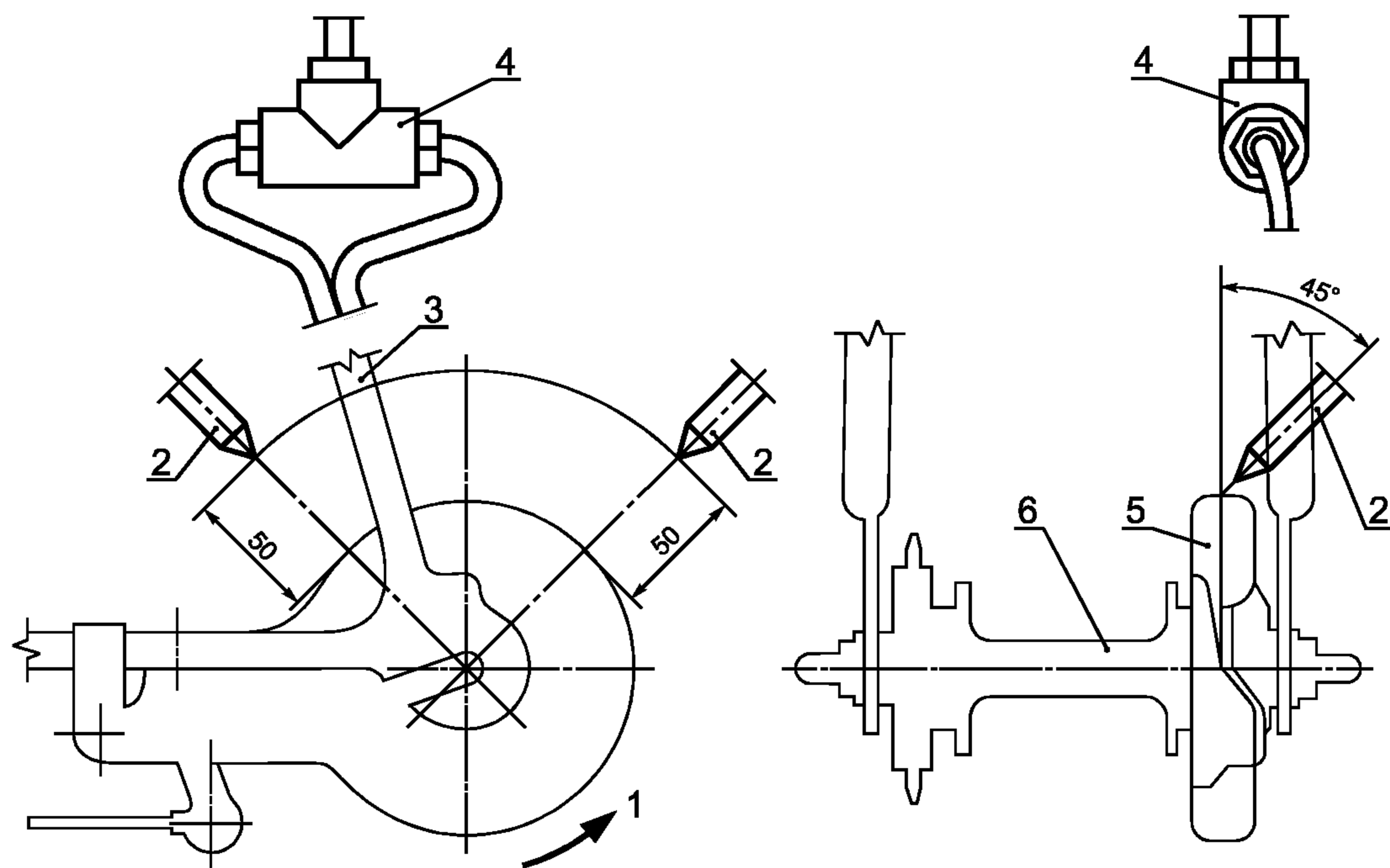
1 — направление вращения колеса; 2 — патрубок; 3 — рама; 4 — задний тройник; 5 — ленточный тормоз; 6 — задняя втулка Рисунок 9 — Патрубки для подачи воды для ленточного тормоза
