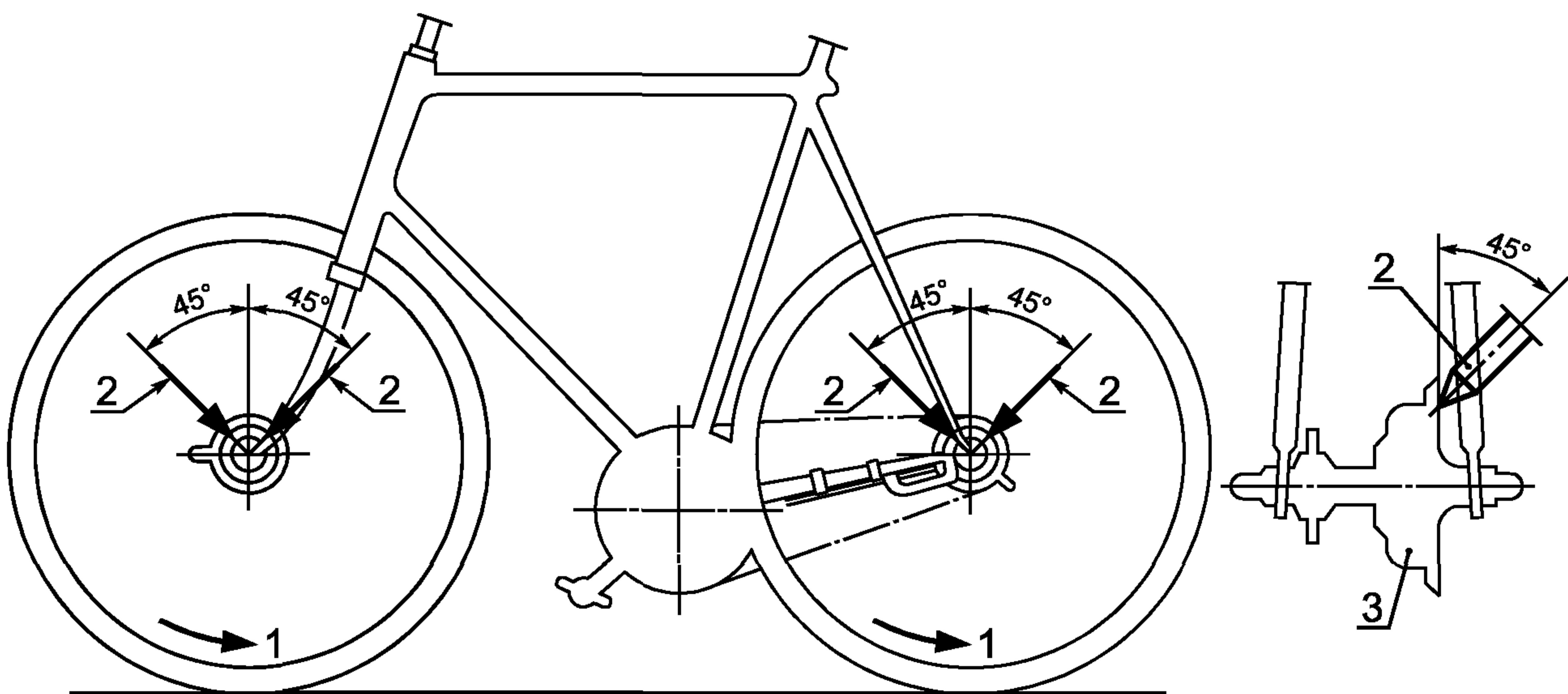
1 — направление вращения колеса; 2 — патрубки; 3 — тормозная втулка
