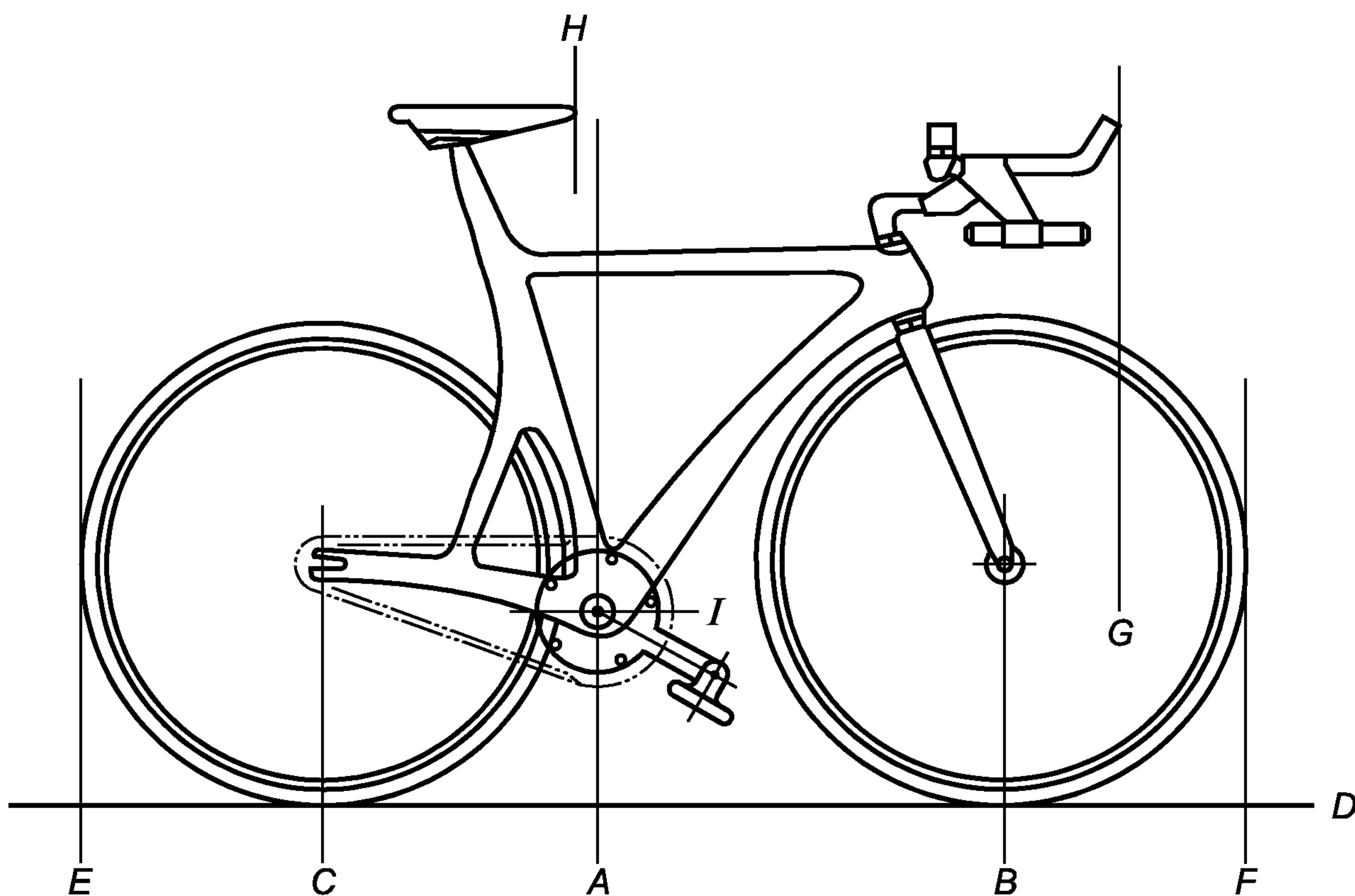
Рисунок 1 — Основные параметры и размеры велосипеда
