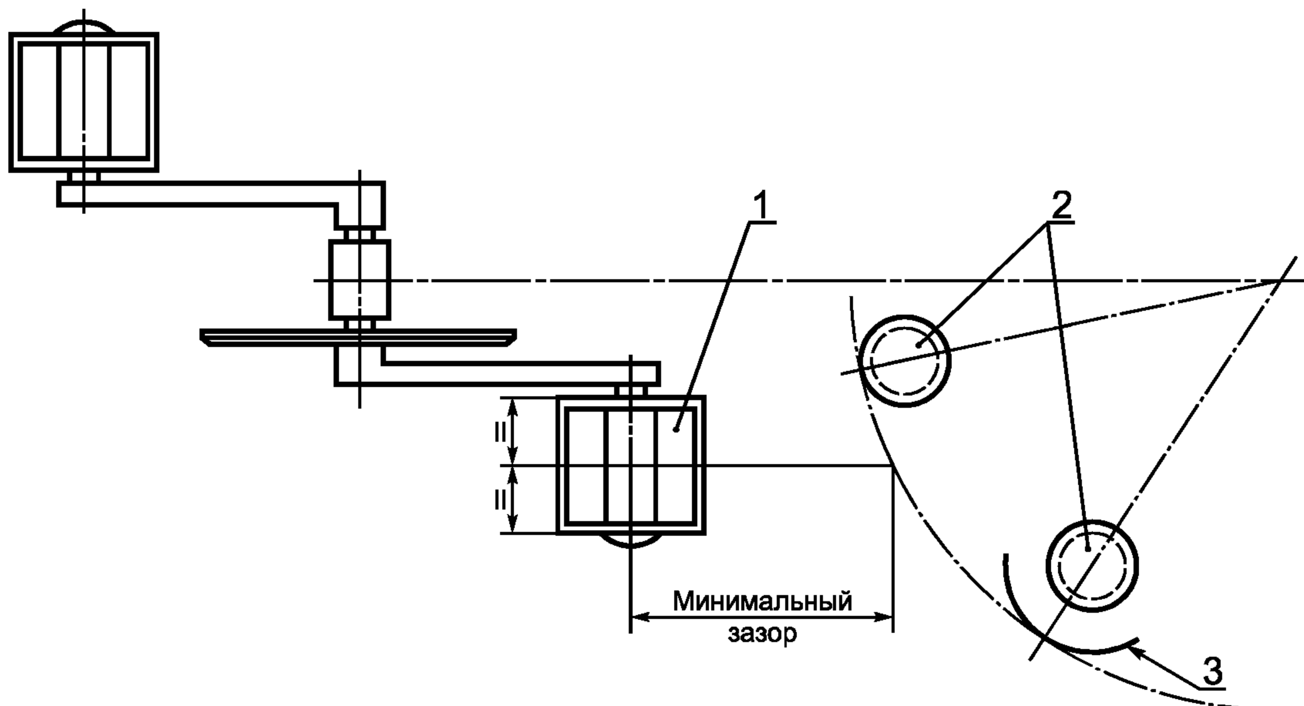
1 — педаль; 2 — шина; 3 — щиток колеса
