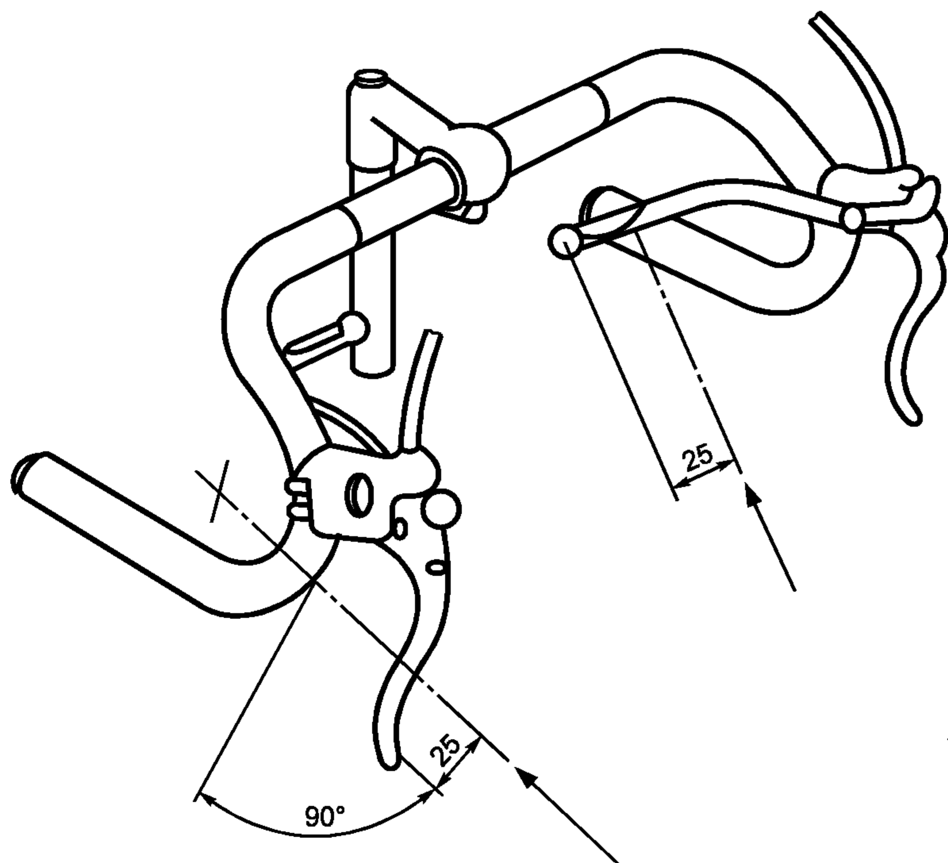
Рисунок 4 — Испытание ручного тормоза нагрузкой
