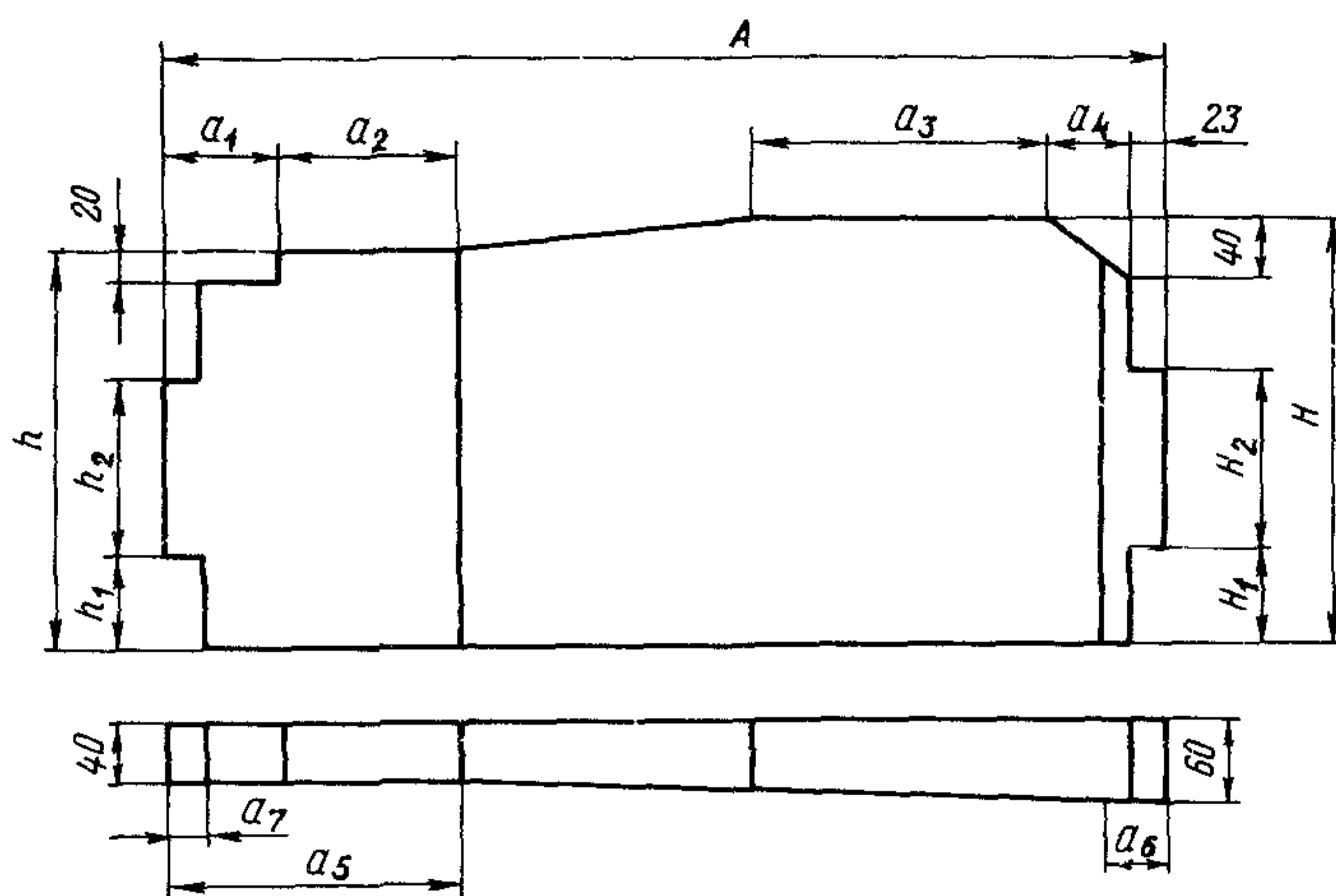
Профилированные лопатки конструкции Донтехэнерго
