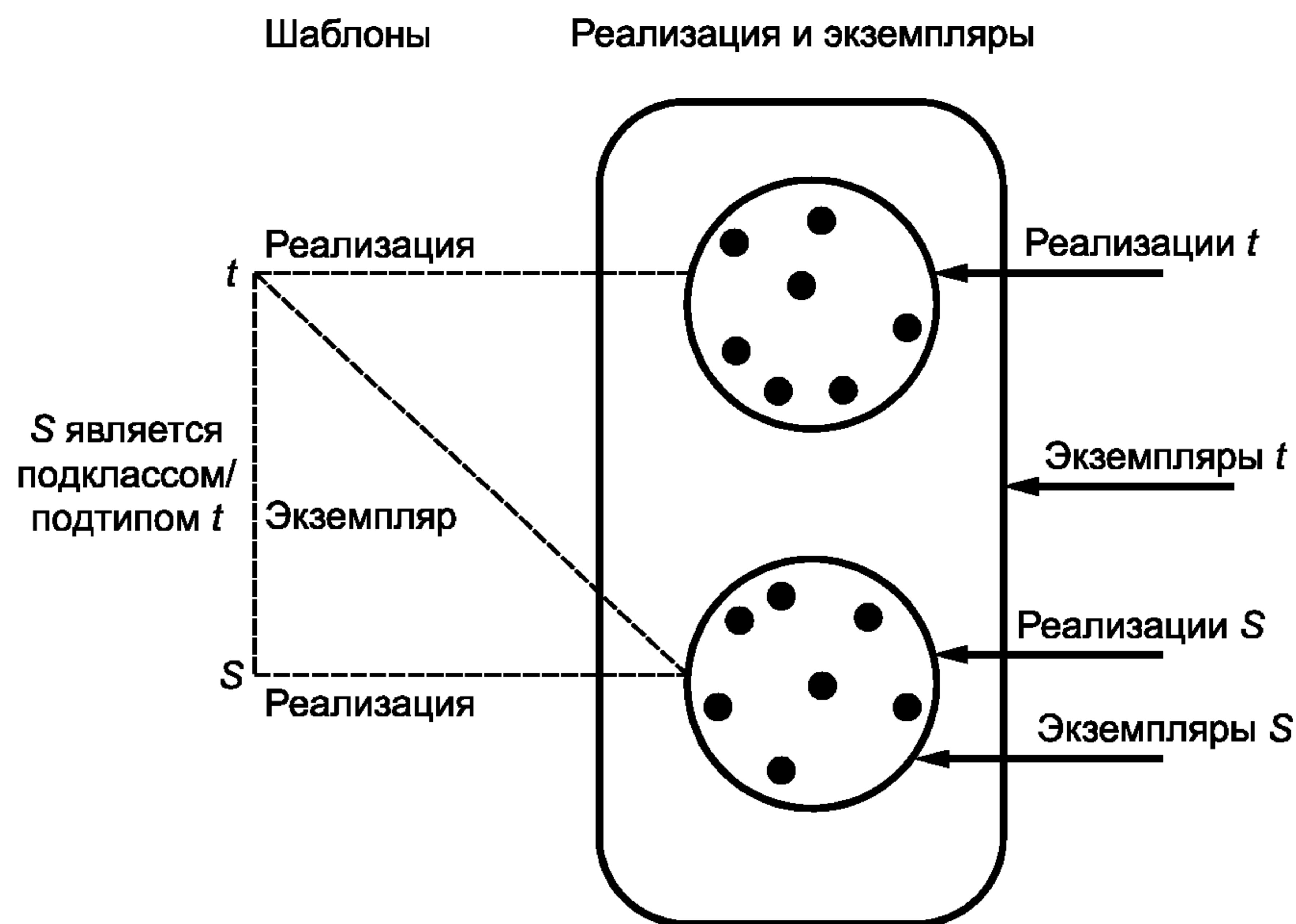
Рисунок 1 — Взаимоотношения между шаблонами, реализациями и экземплярами
