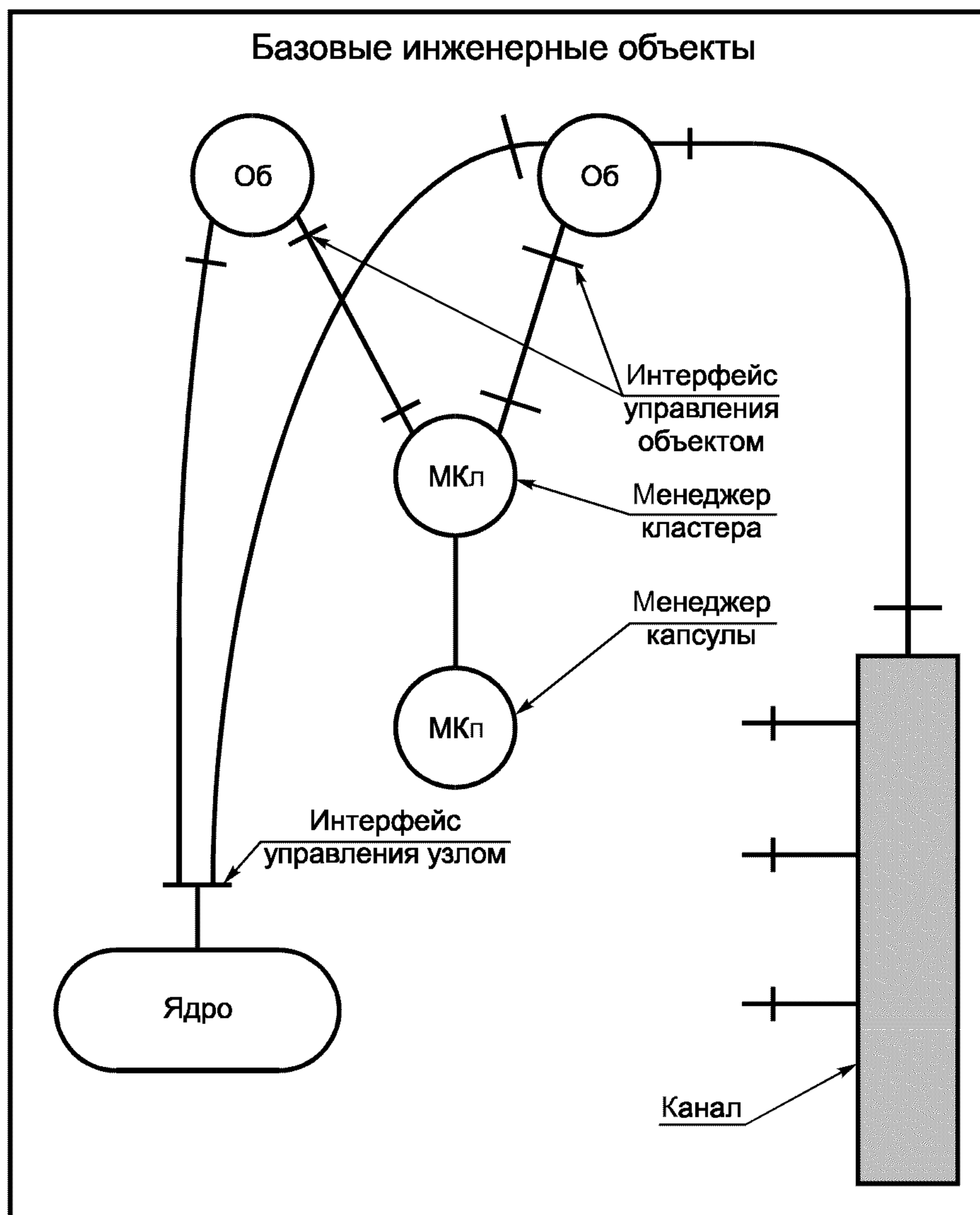
Рисунок 4 — Пример структуры, поддерживающий базовый инженерный объект
