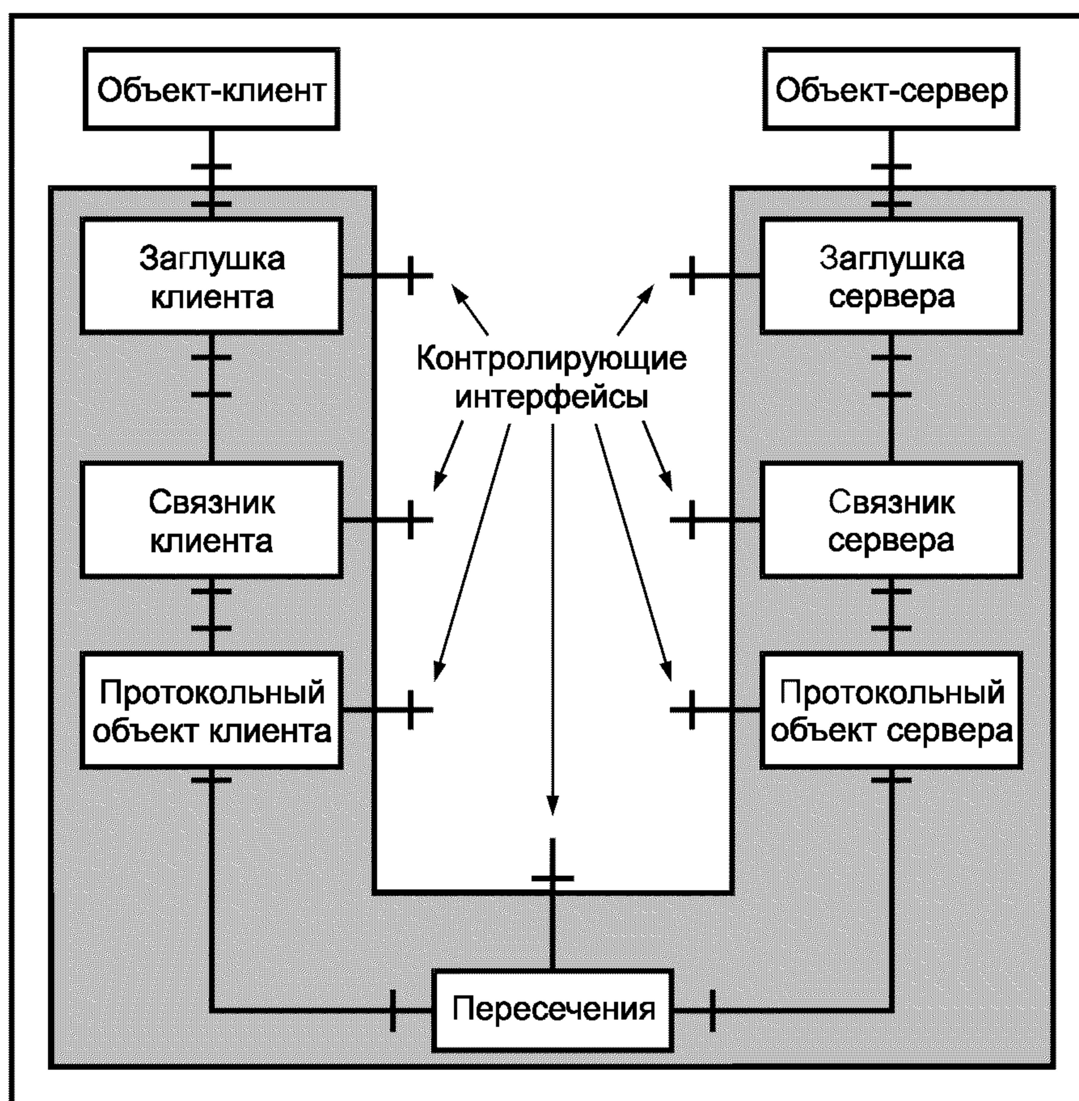
Рисунок 2 — Пример базового канала клиент/сервер
