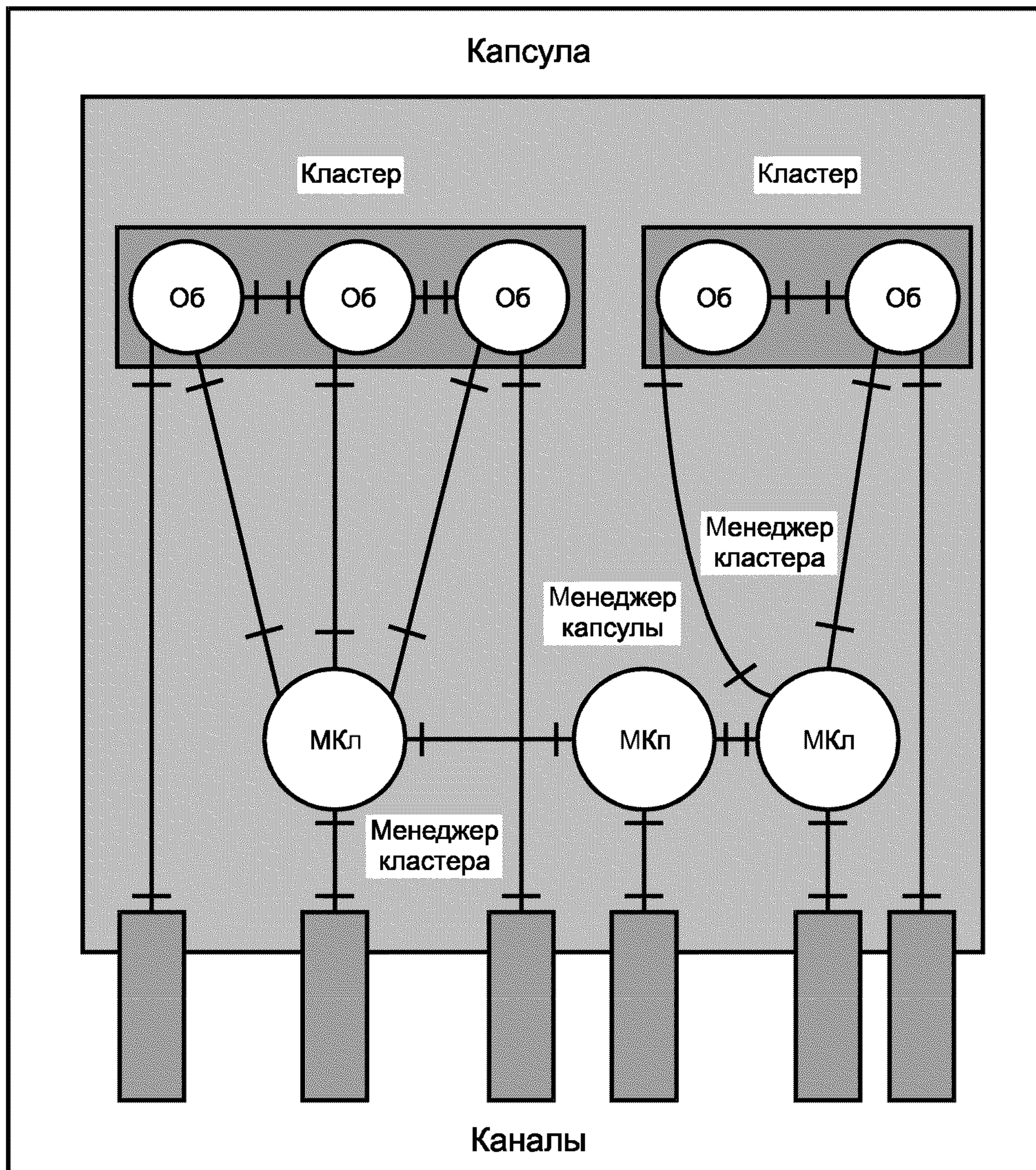
Рисунок 5 — Пример структуры капсулы
