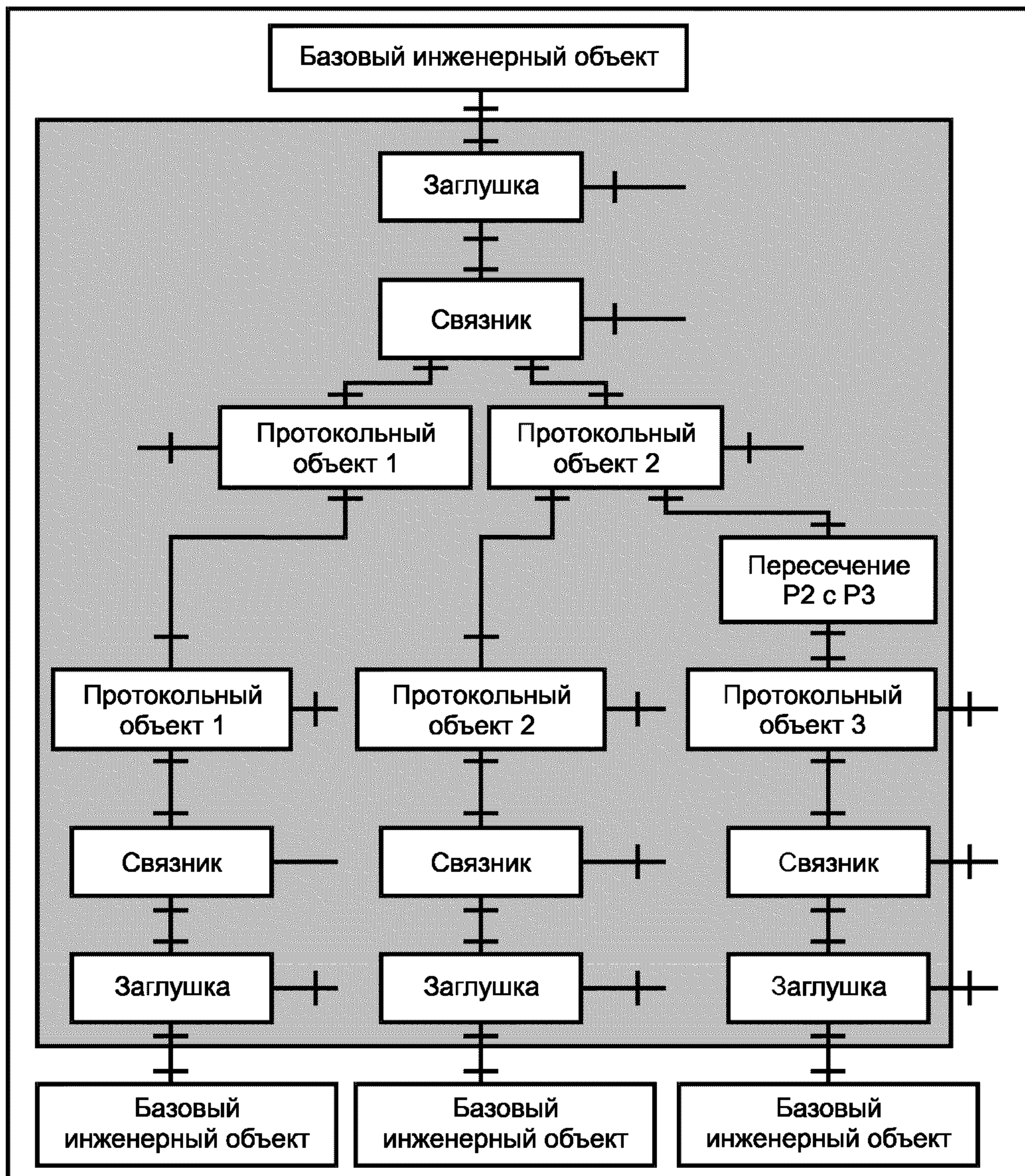
Рисунок 3 — Пример канала с несколькими оконечными точками
