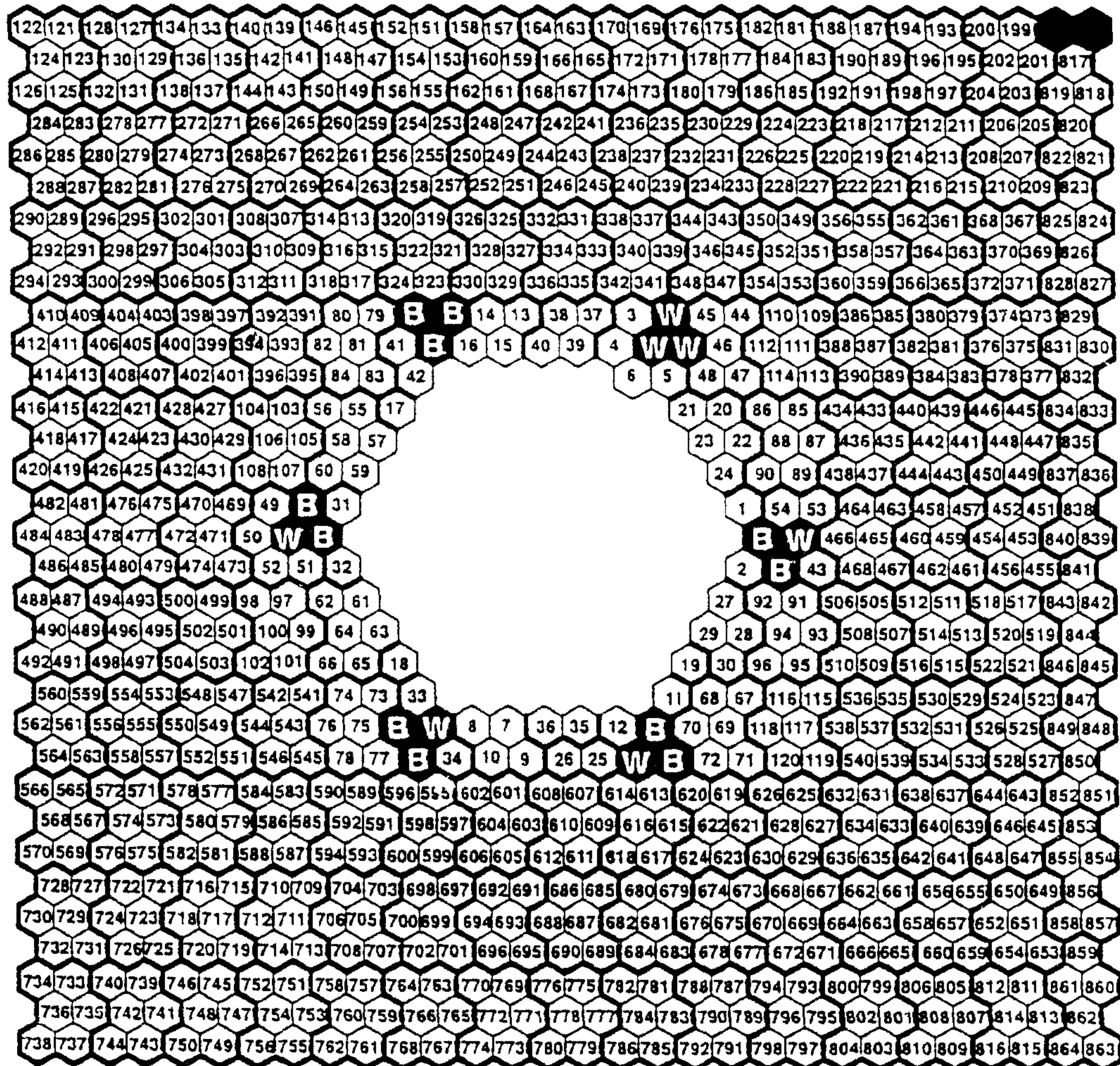
Рисунок 5 — Последовательность модулей MaxiCode
