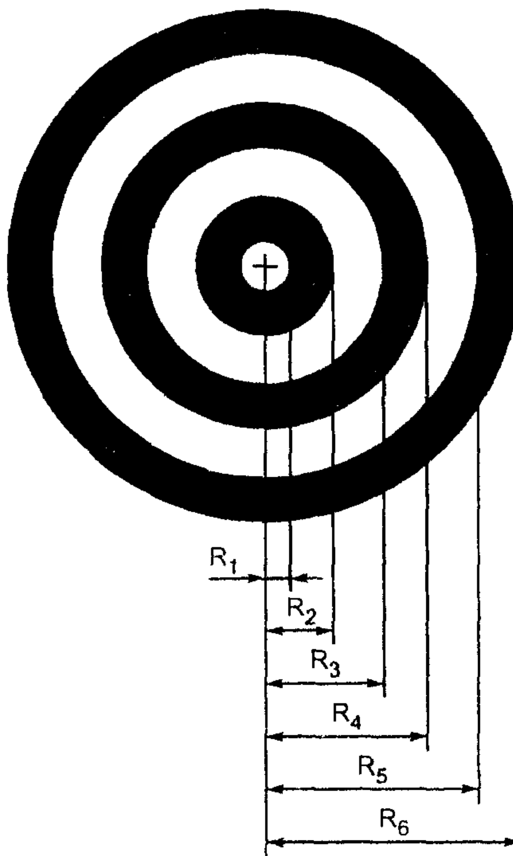
Рисунок 9 — Размеры шаблона поиска MaxiCode
