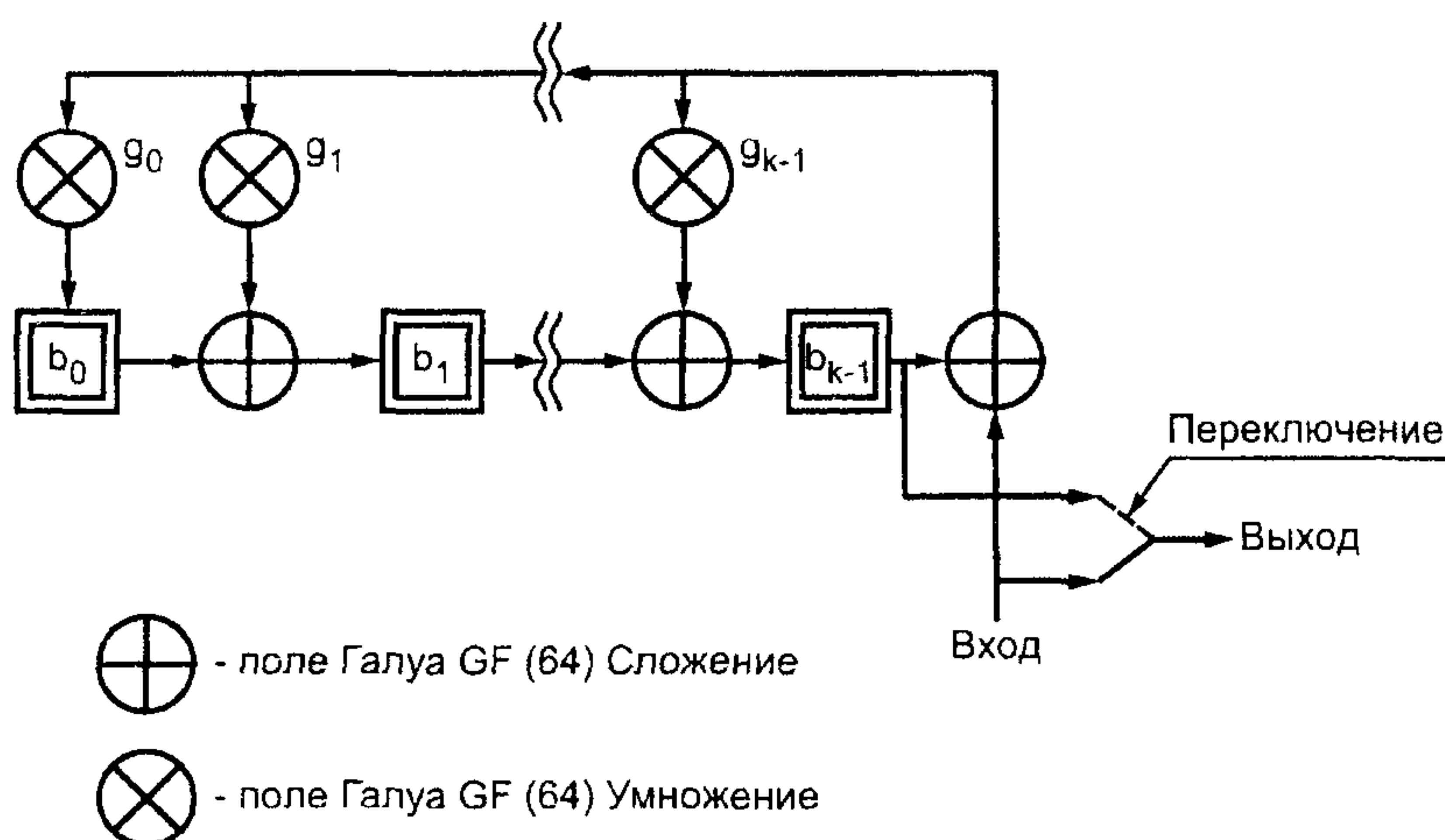
Рисунок 7 — Схема кодирования кодовых слов коррекции ошибок
