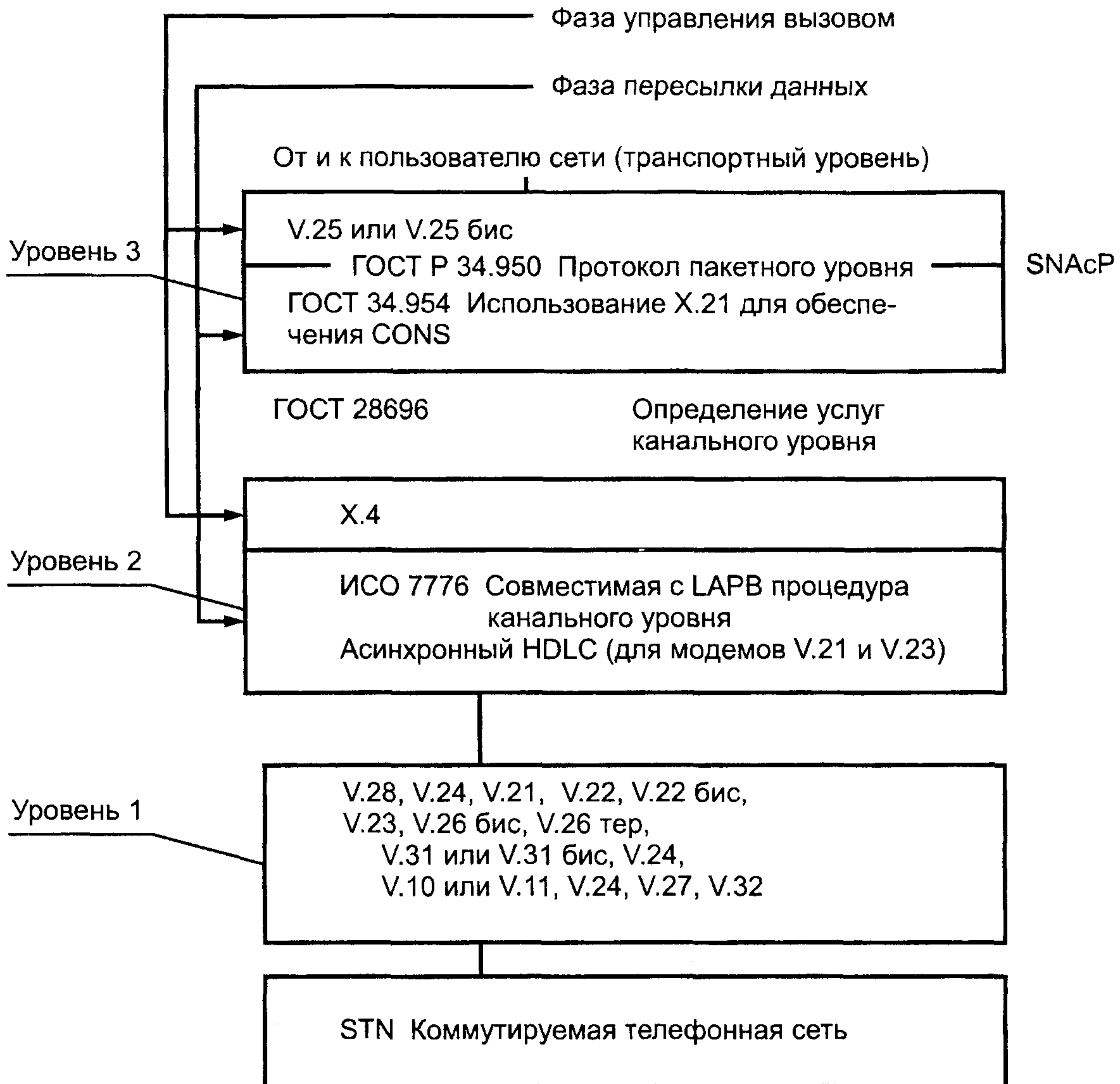
Рисунок 6 — Описание модели коммутируемой телефонной сети
