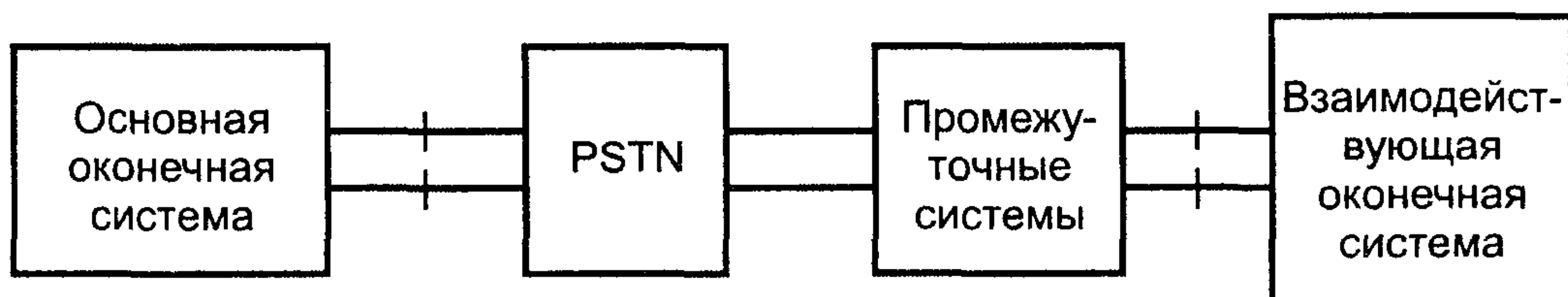
Рисунок 5 — Схема организации коммутируемого телефонного канала
