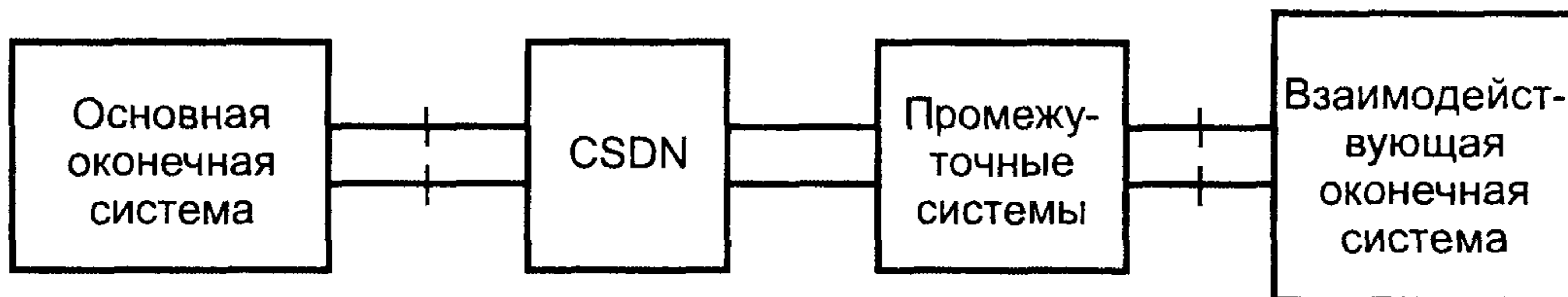
Рисунок 3 — Схема сети передачи данных с коммутацией каналов
