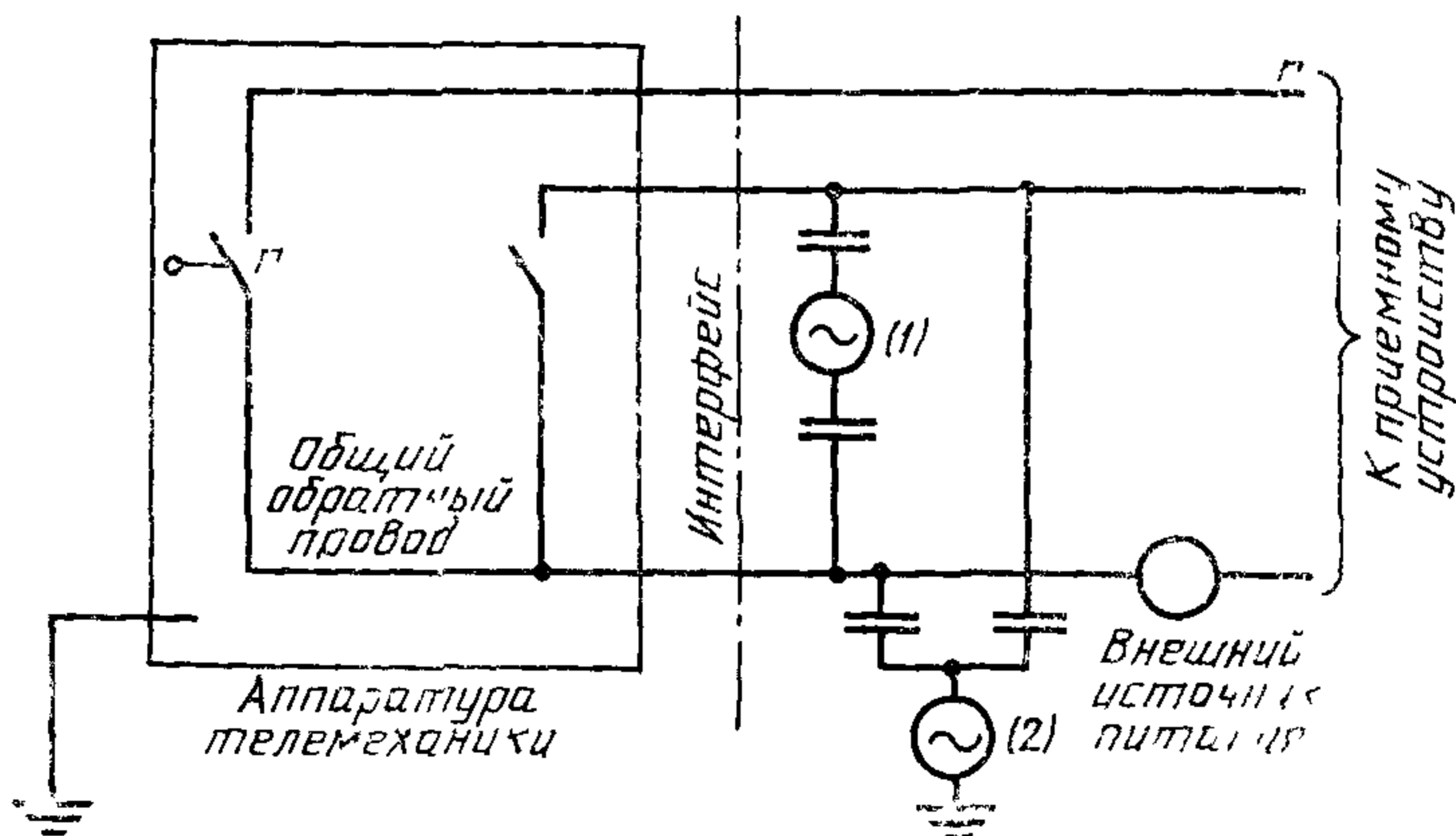
а) схема для пассивных двоичных выходных сигналов
