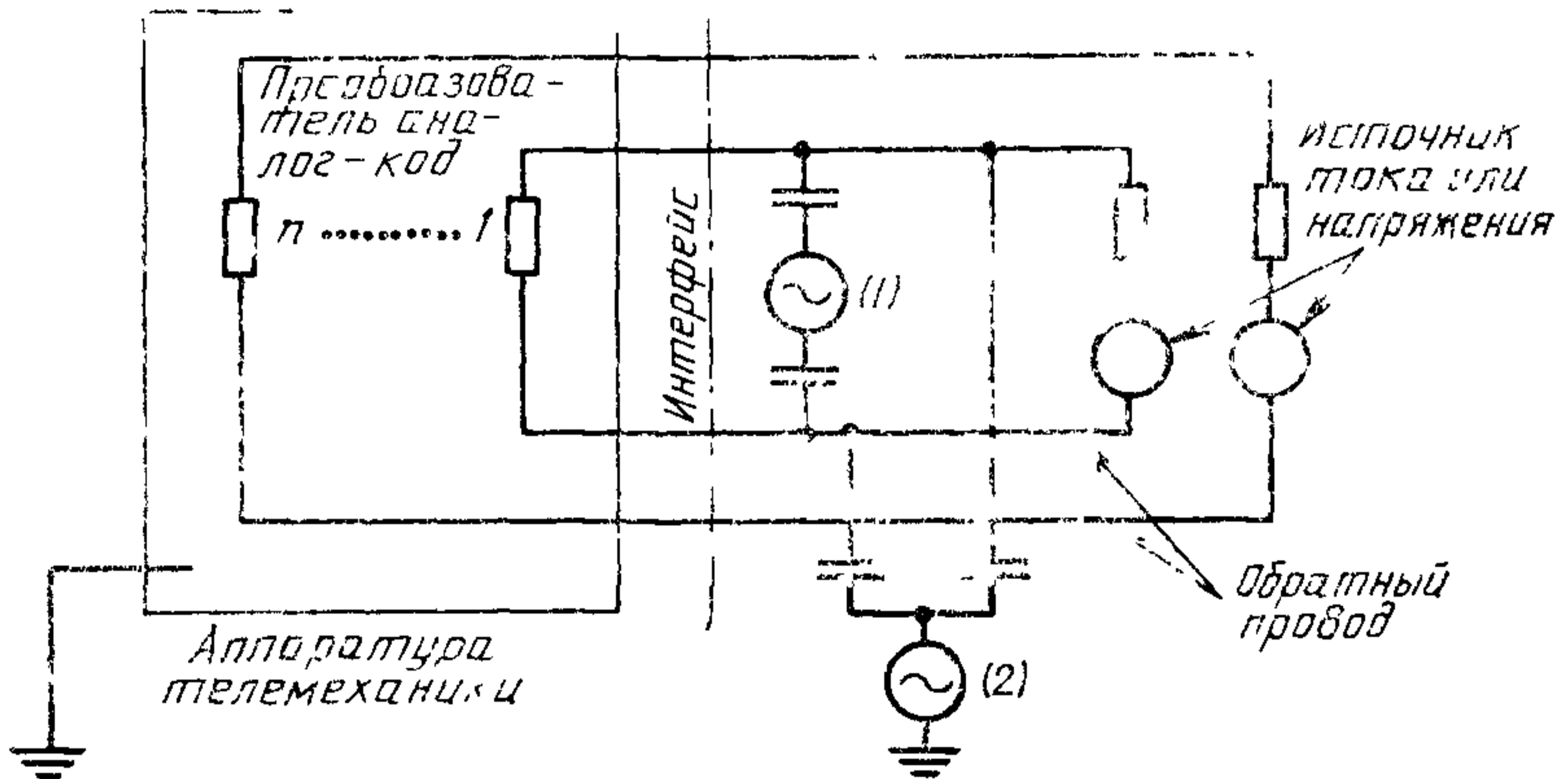
Схема для аналоговых входных сигналов
