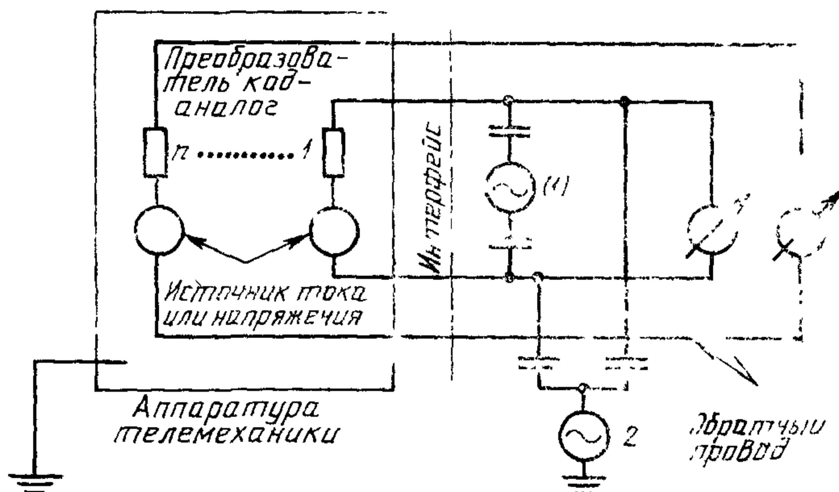
Схема для аналоговых выходных сигналов
