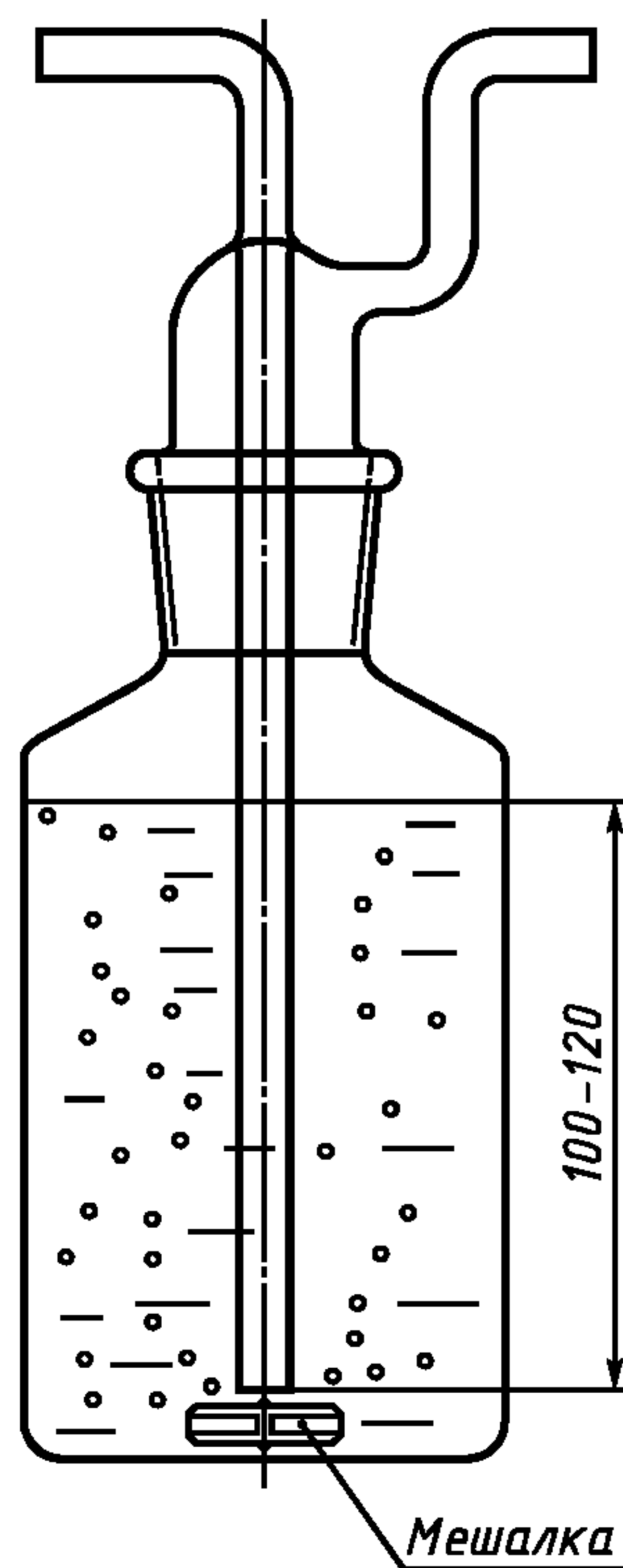
Рисунок А.2 — Пример промывочного сосуда
