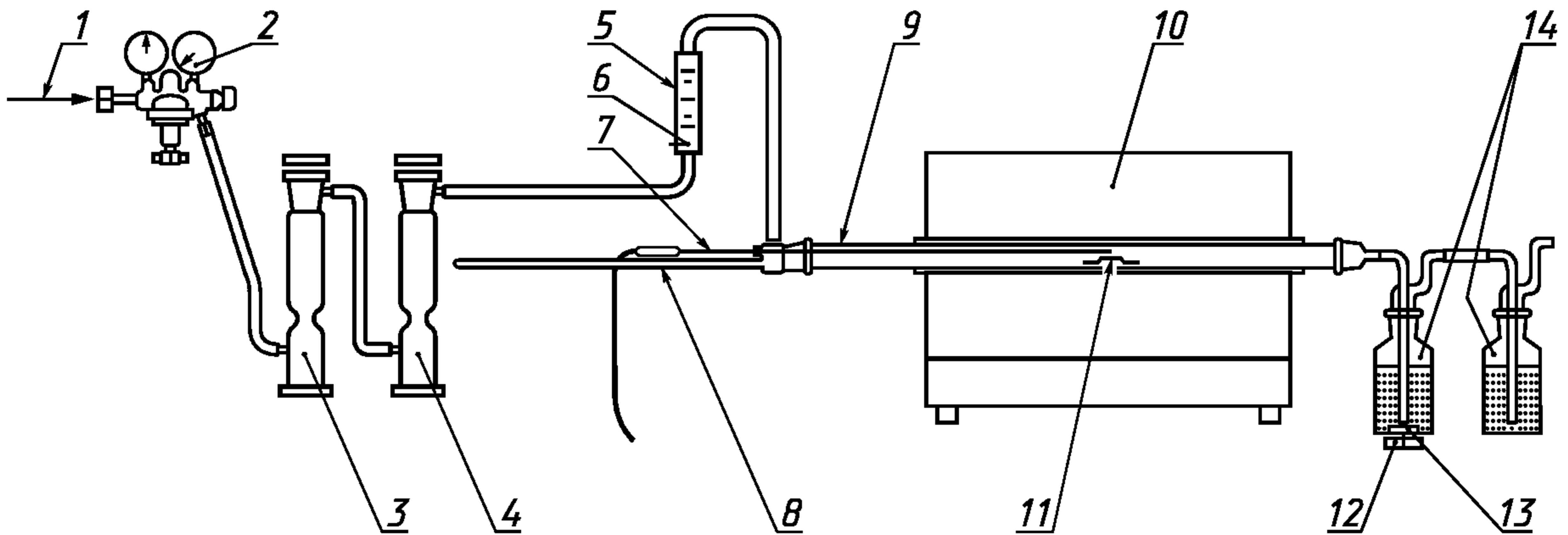
1 — сжатый воздух; 2 — редуктор; 3 — воздушный фильтр (активированный уголь); 4 — осушитель воздуха (селикагель); 5 — ротаметр; 6 — игольчатый вентиль; 7 — термопара; 8 — устройство для ввода лодочки с образцом; 9 — трубка из квар- цевого стекла; 10 — печь; 11 — лодочка с образцом; 12 — магнитная мешалка; 13 — стержень магнитной мешалки; 14 — промывочные сосуды
