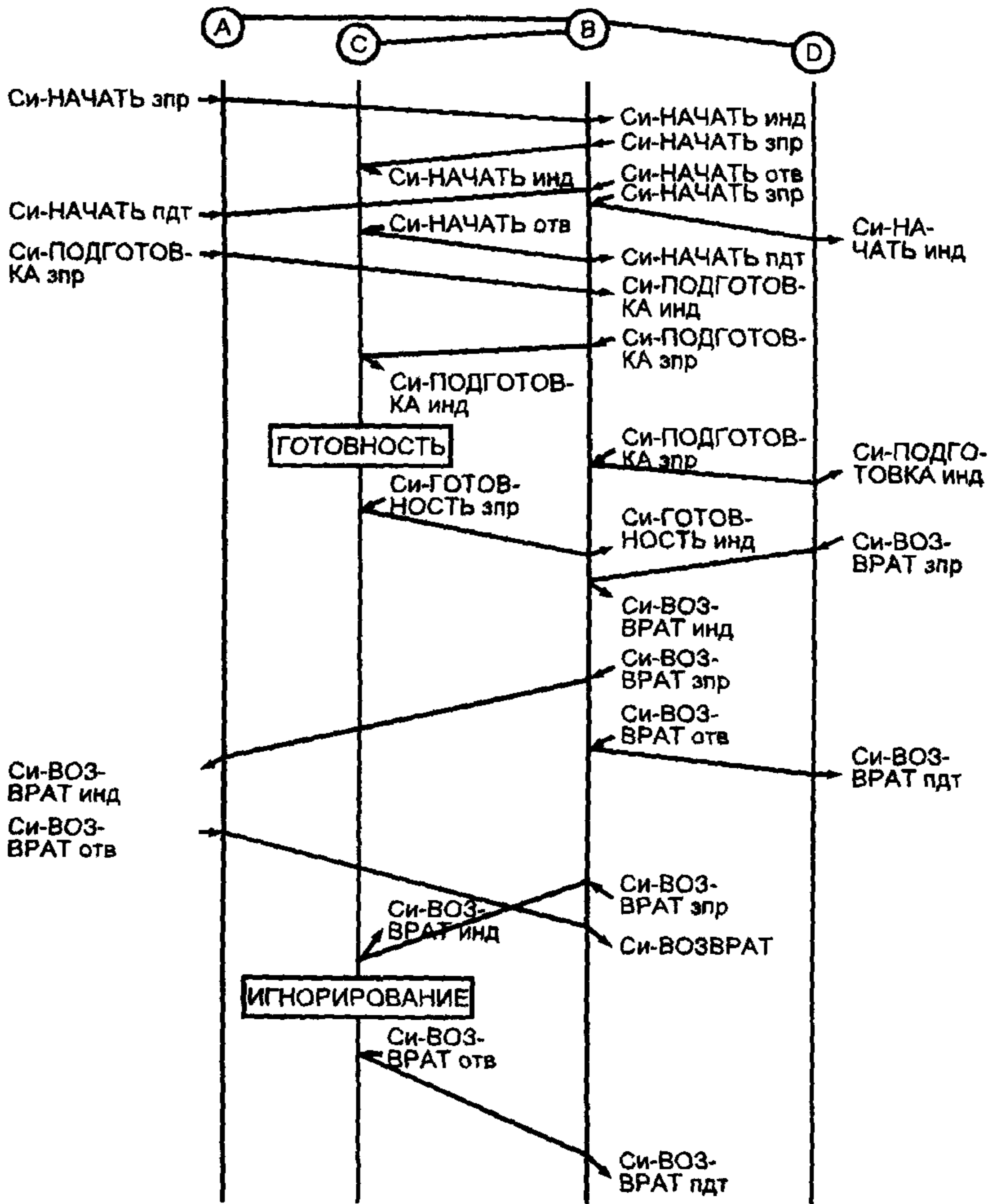
Рисунок С.5 — Последовательность примитивов — ВОЗВРАТ атомарного действия
