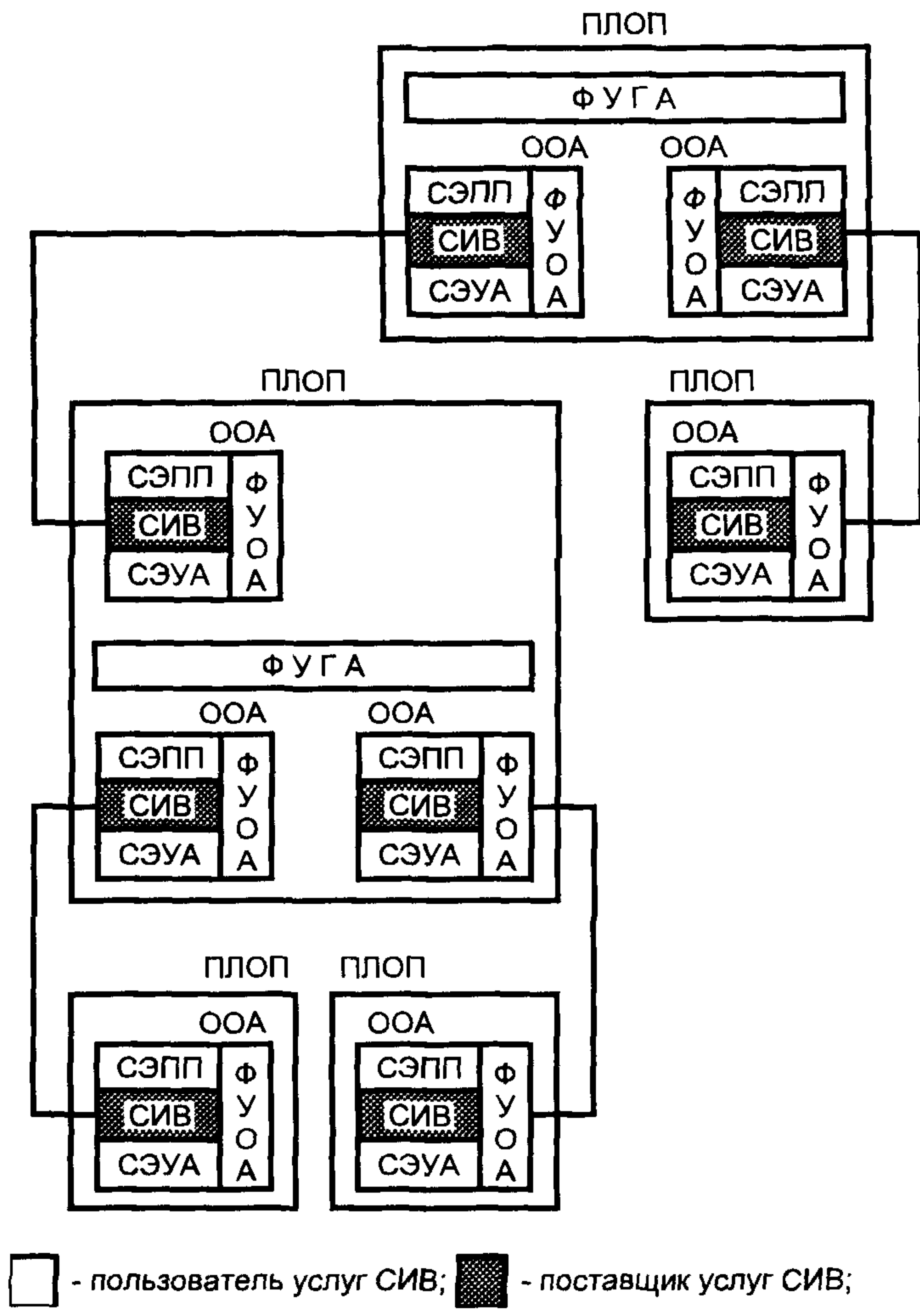
Рисунок В.1 — Архитектура дерева атомарного действия
