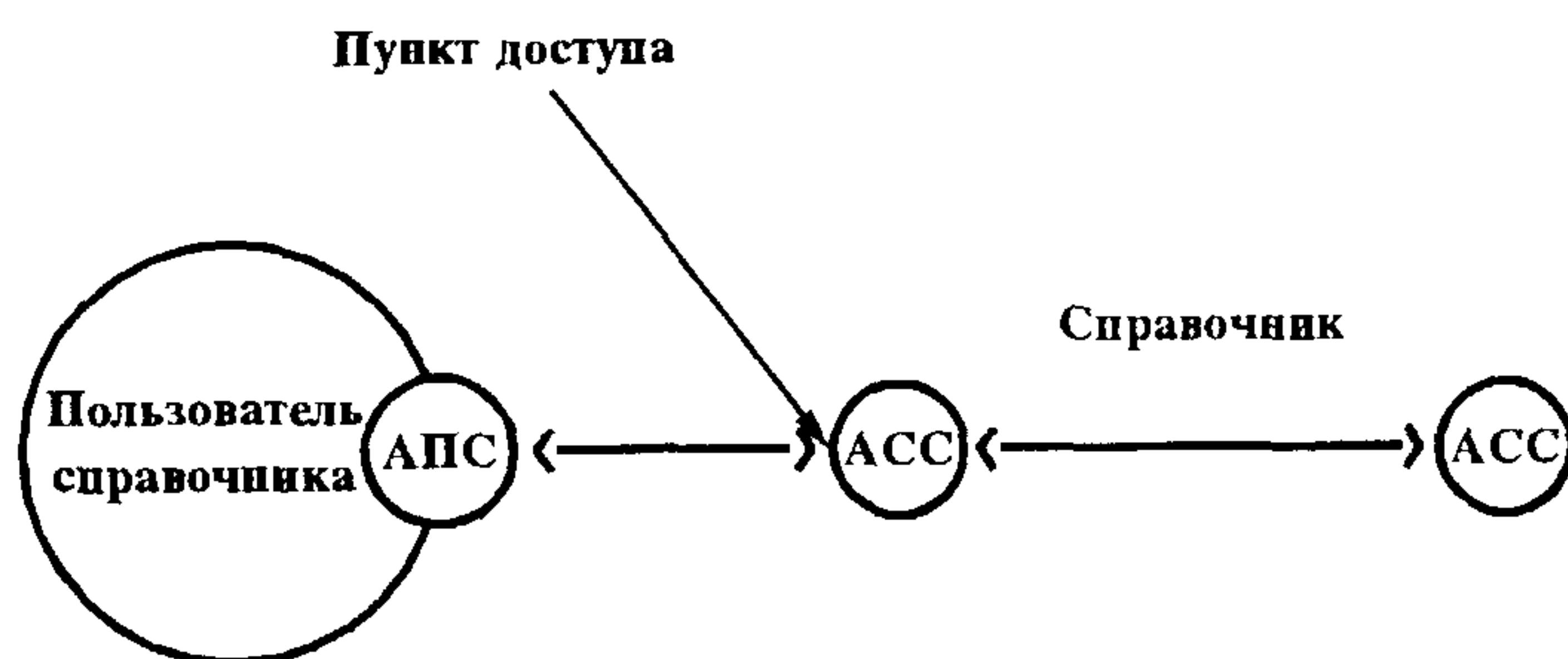
Рисунок 1 — Взаимодействия справочника
