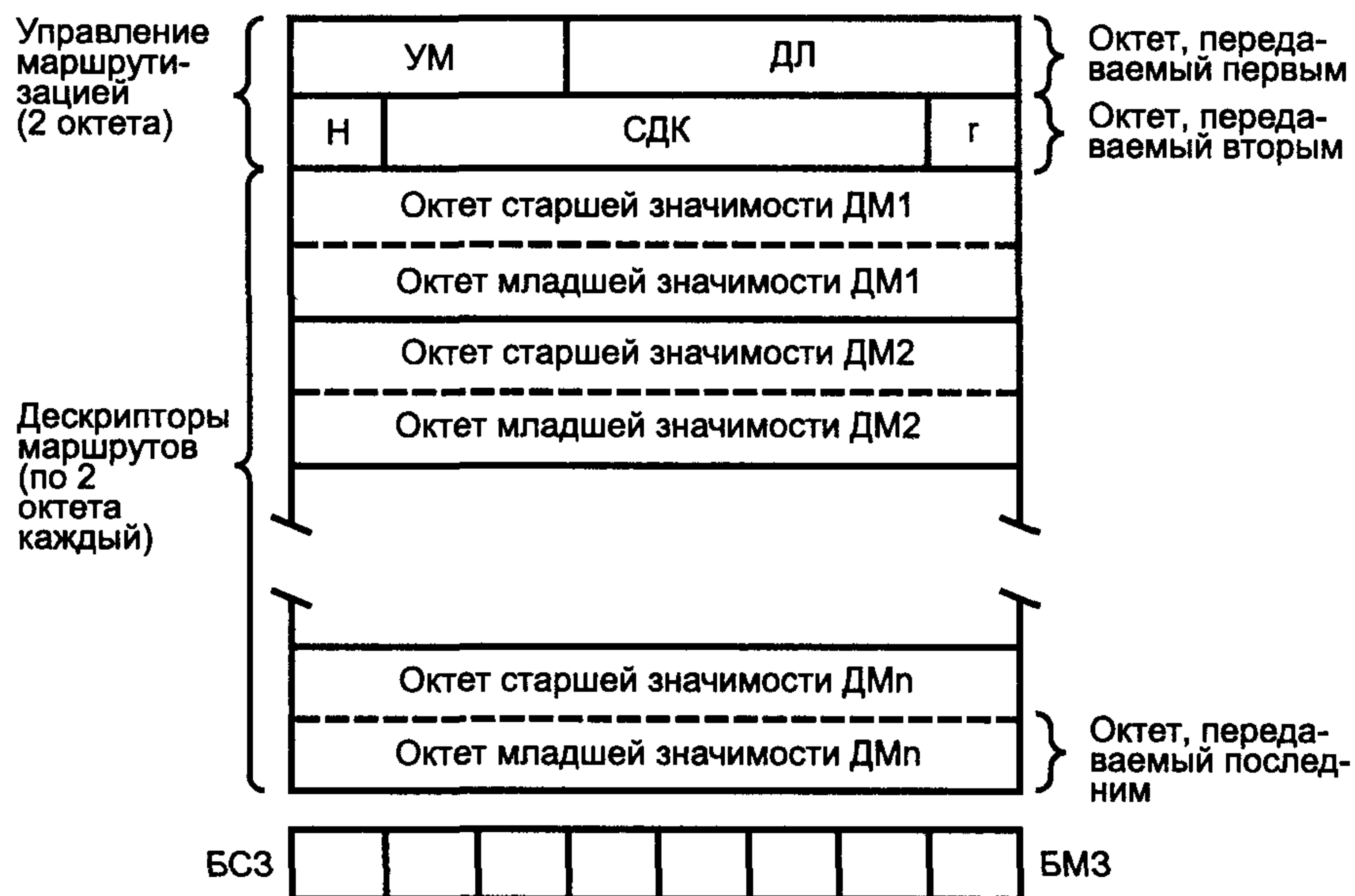
Рисунок С.3 — Поле информации маршрутизации
