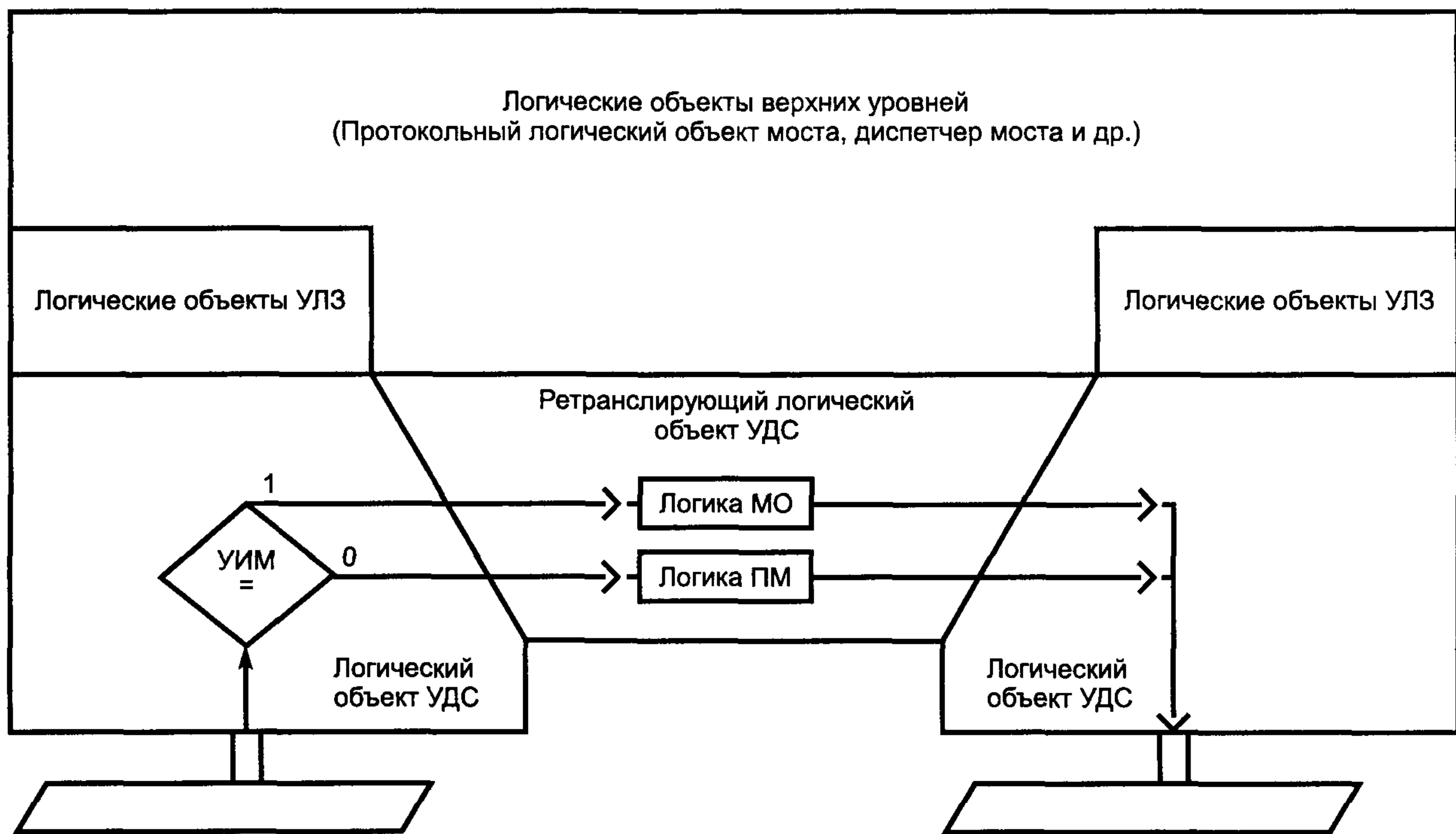
Рисунок С.1 — Логика операций моста ПМСО
