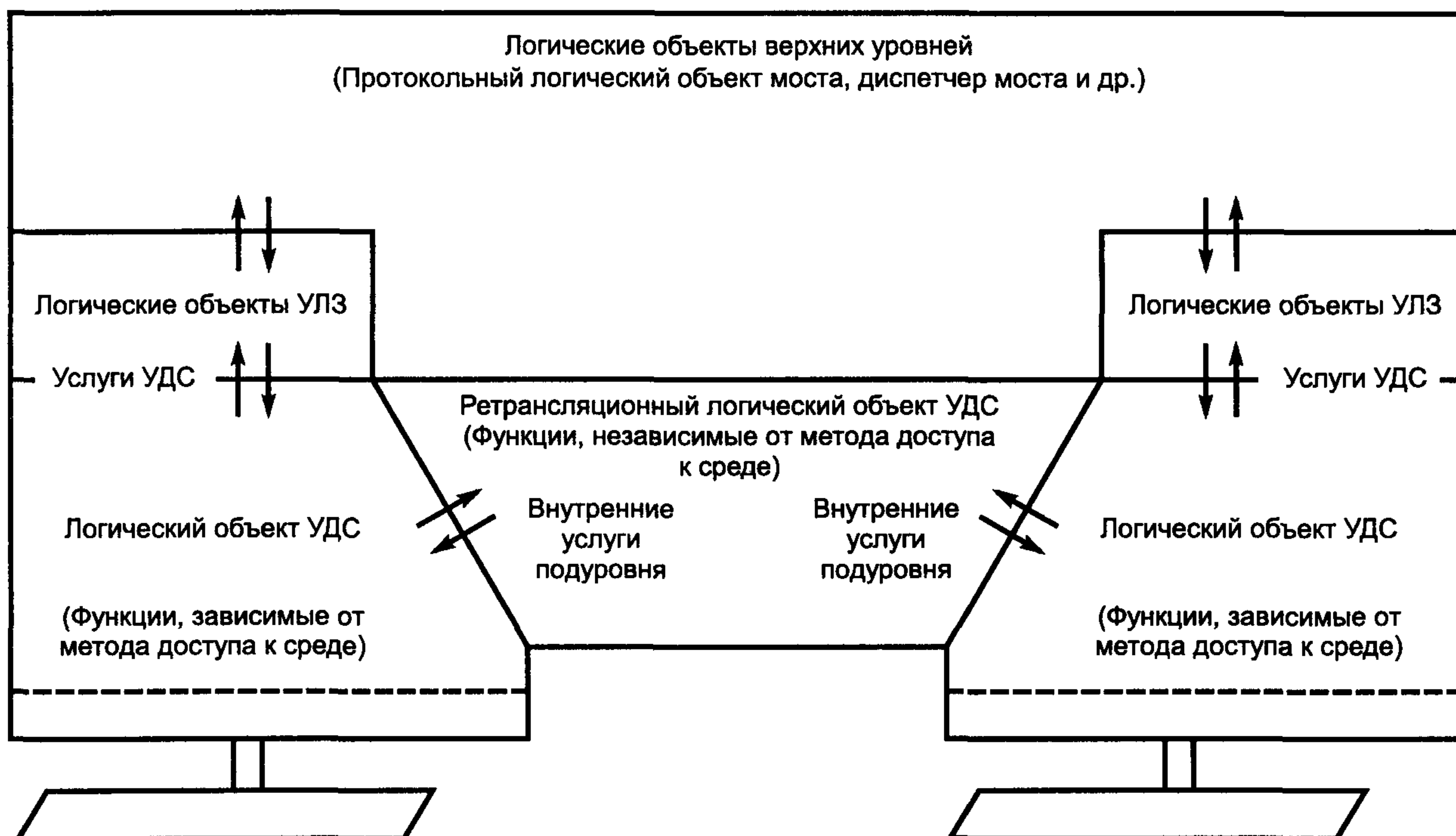
Рисунок 3.3 — Архитектура моста
