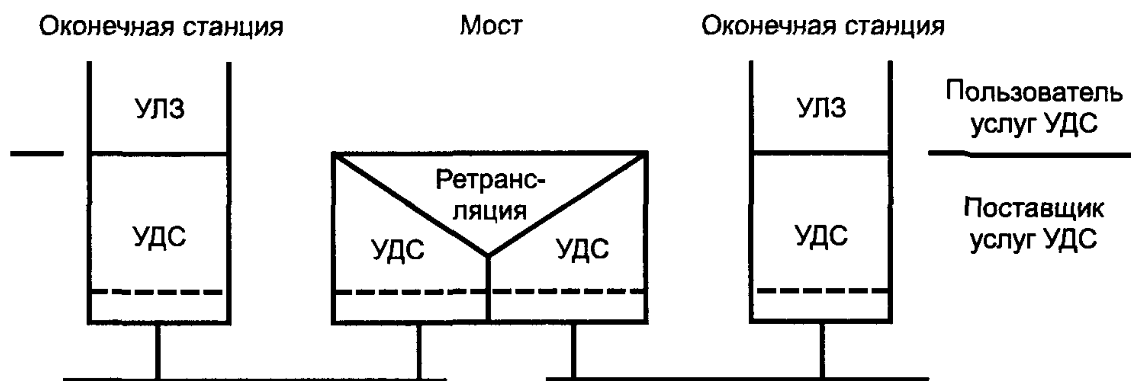
Рисунок 2.1 — Внутренняя организация подуровня УДС
