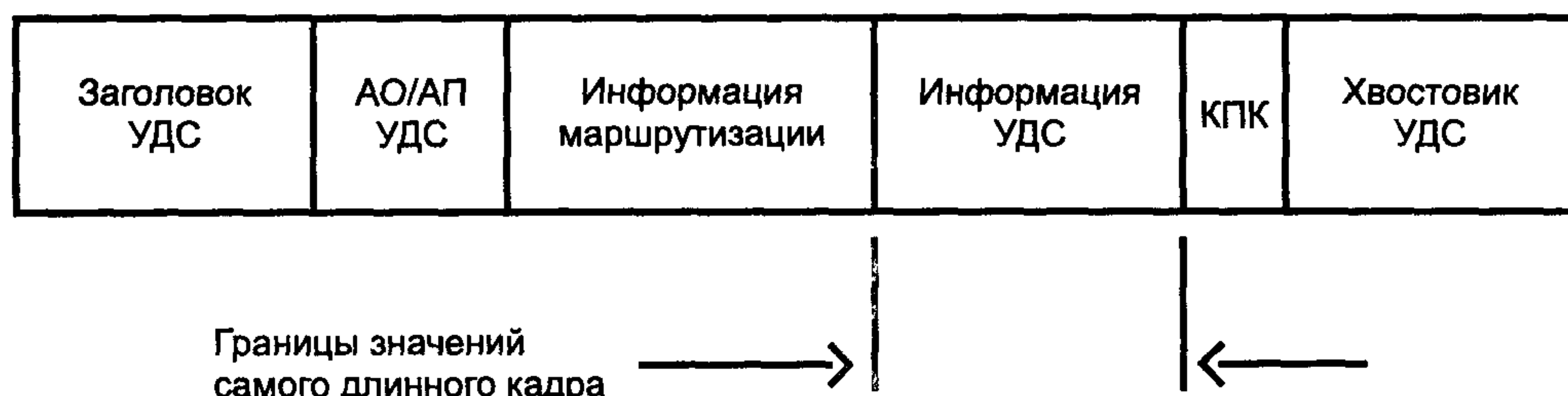
Рисунок С.6 — Границы значений самого длинного кадра
