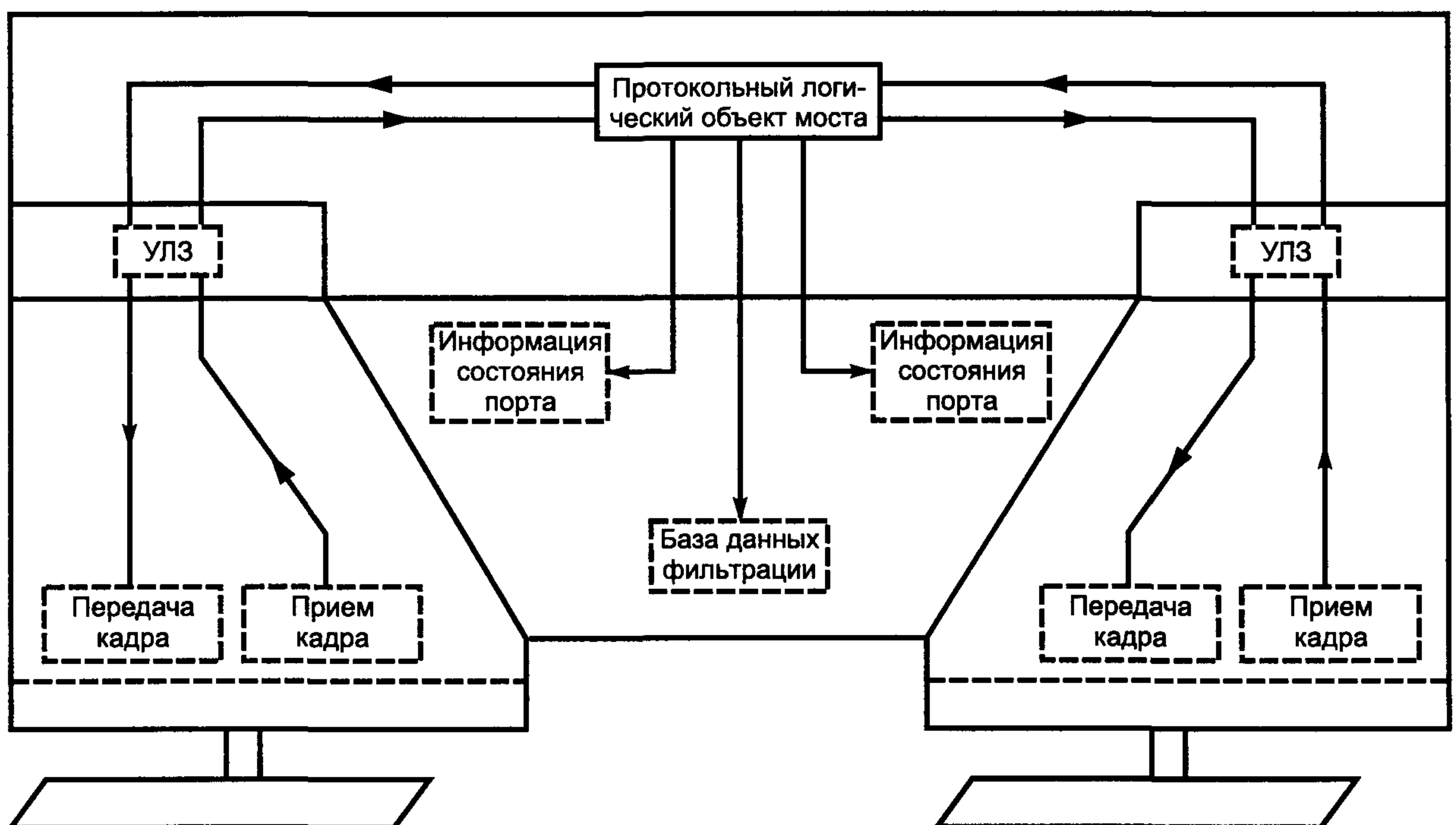
Рисунок 3.6 — Операции межмостового протокола
