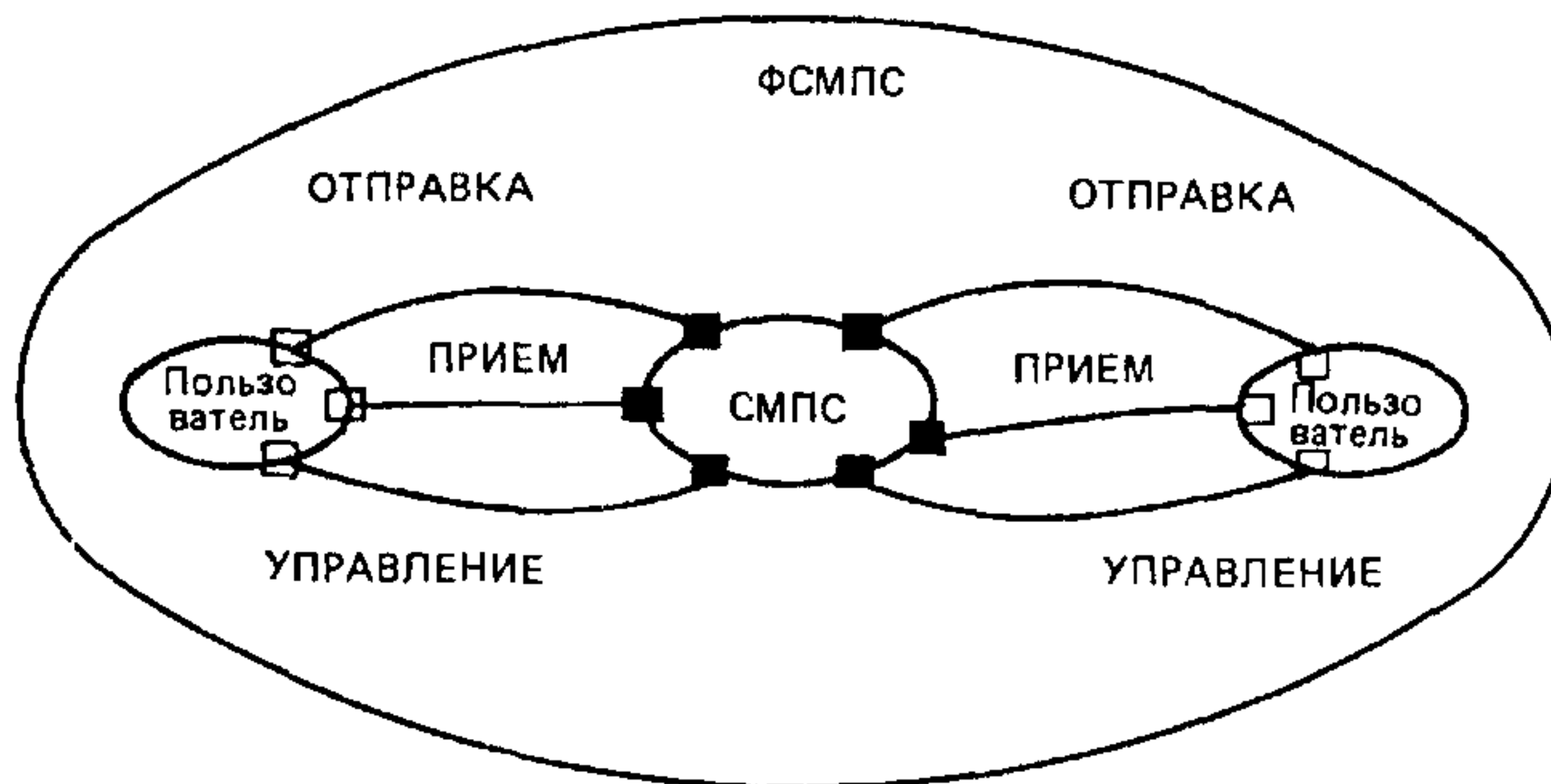
Рисунок 3 — Функциональная среда межперсональных сообщений
