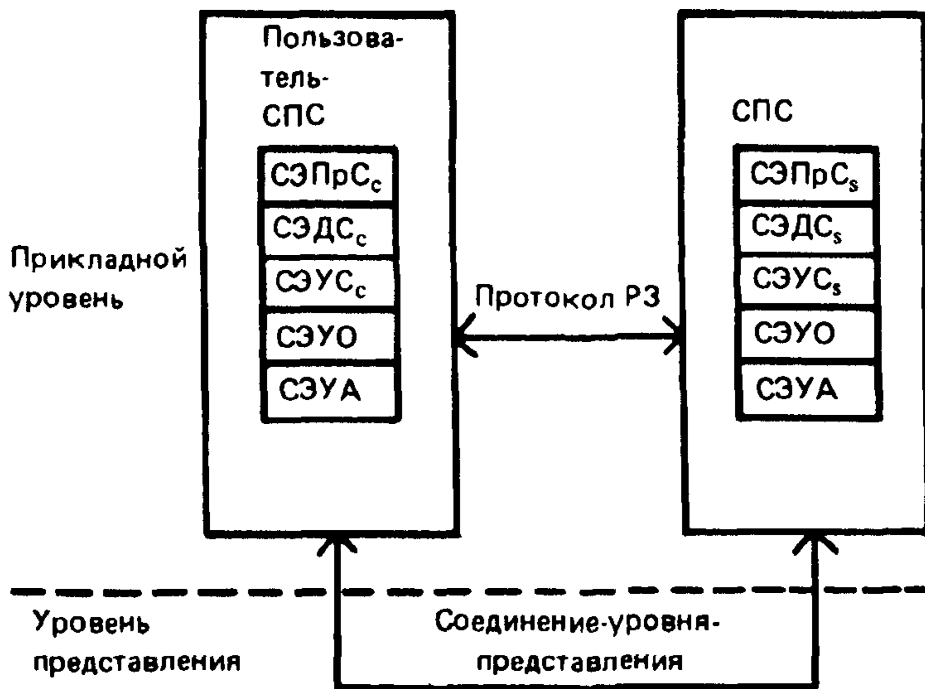
Рисунок 1 — Модель протокола доступа СПС
