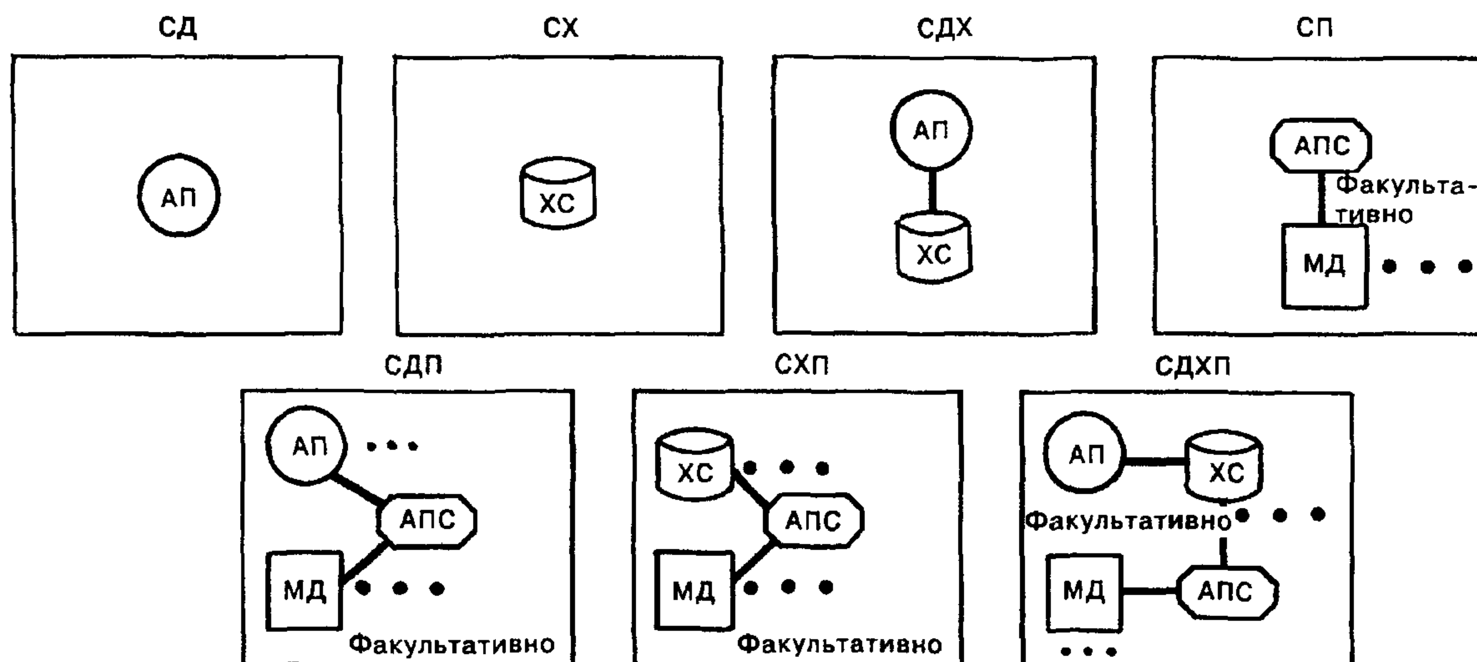
Рисунок 8 — Типы систем сообщений
