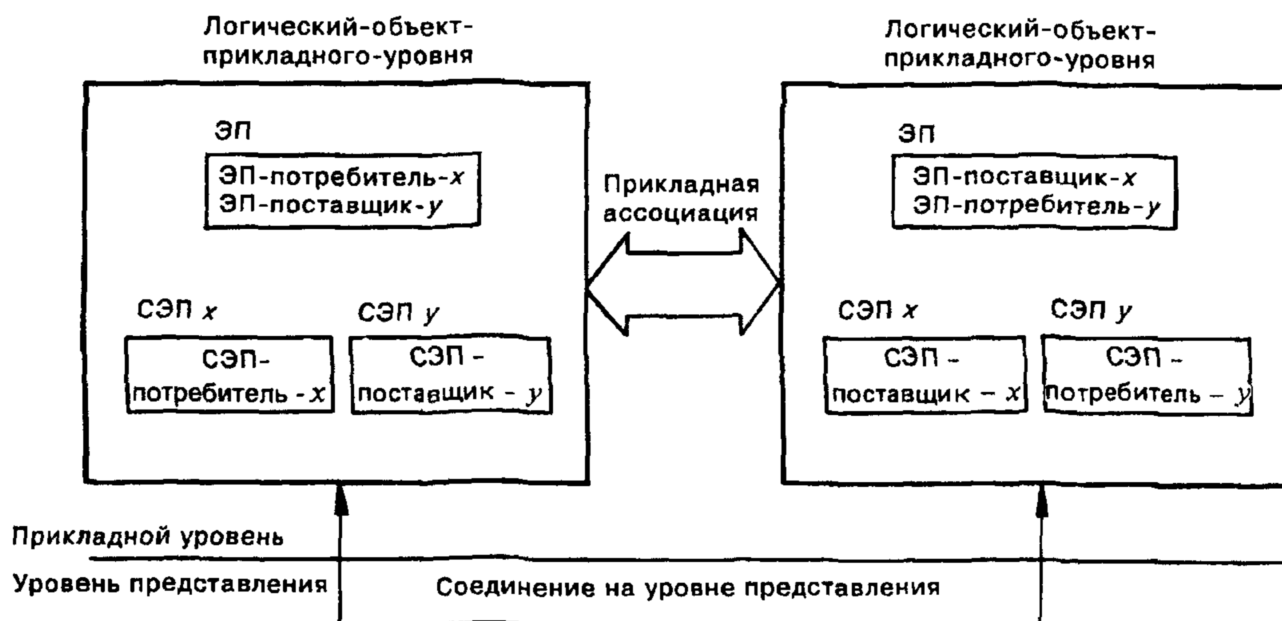
Рисунок 15 — Несколько асимметричных СЭП
