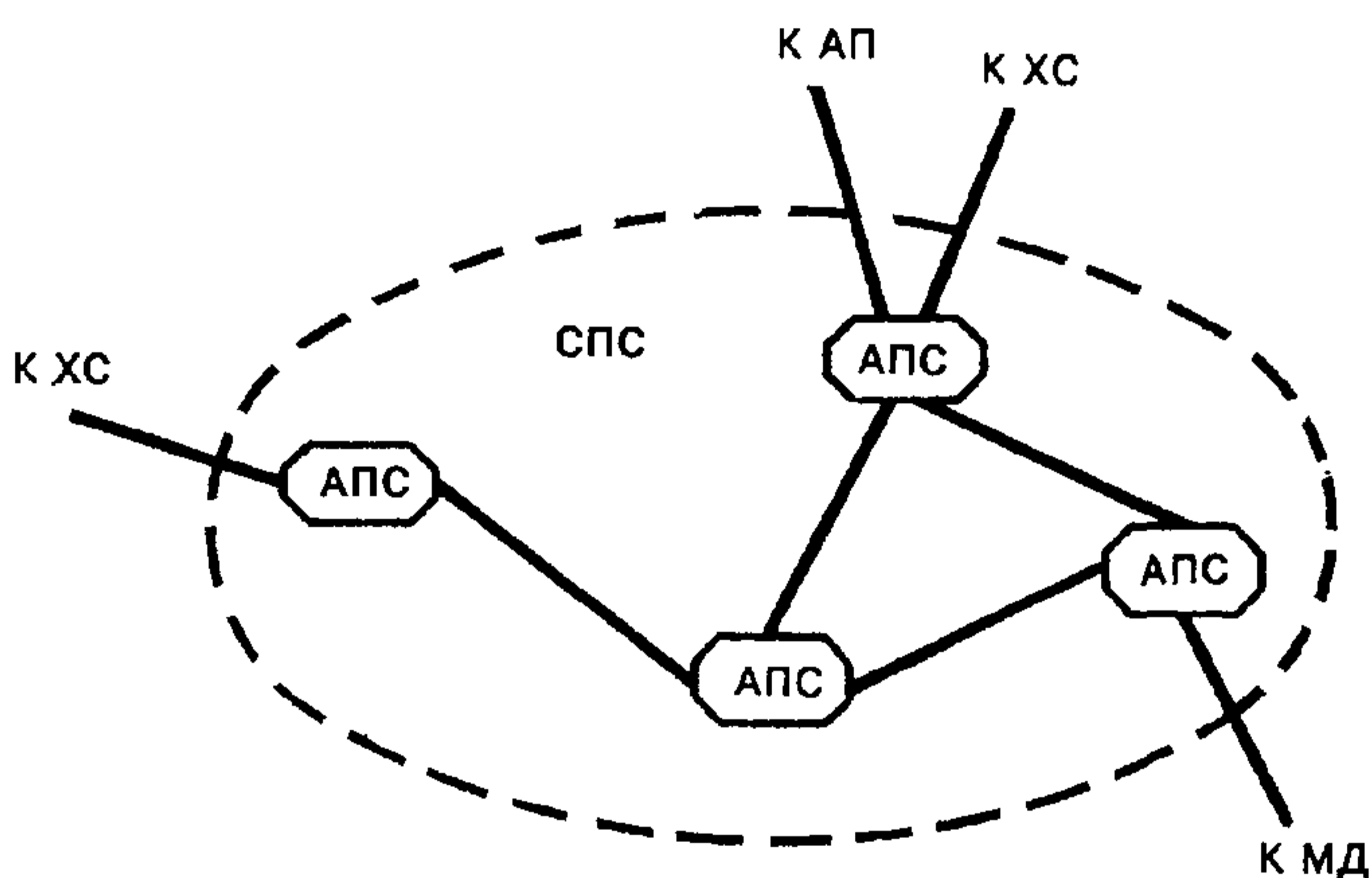
Рисунок 3 — Система передачи сообщений
