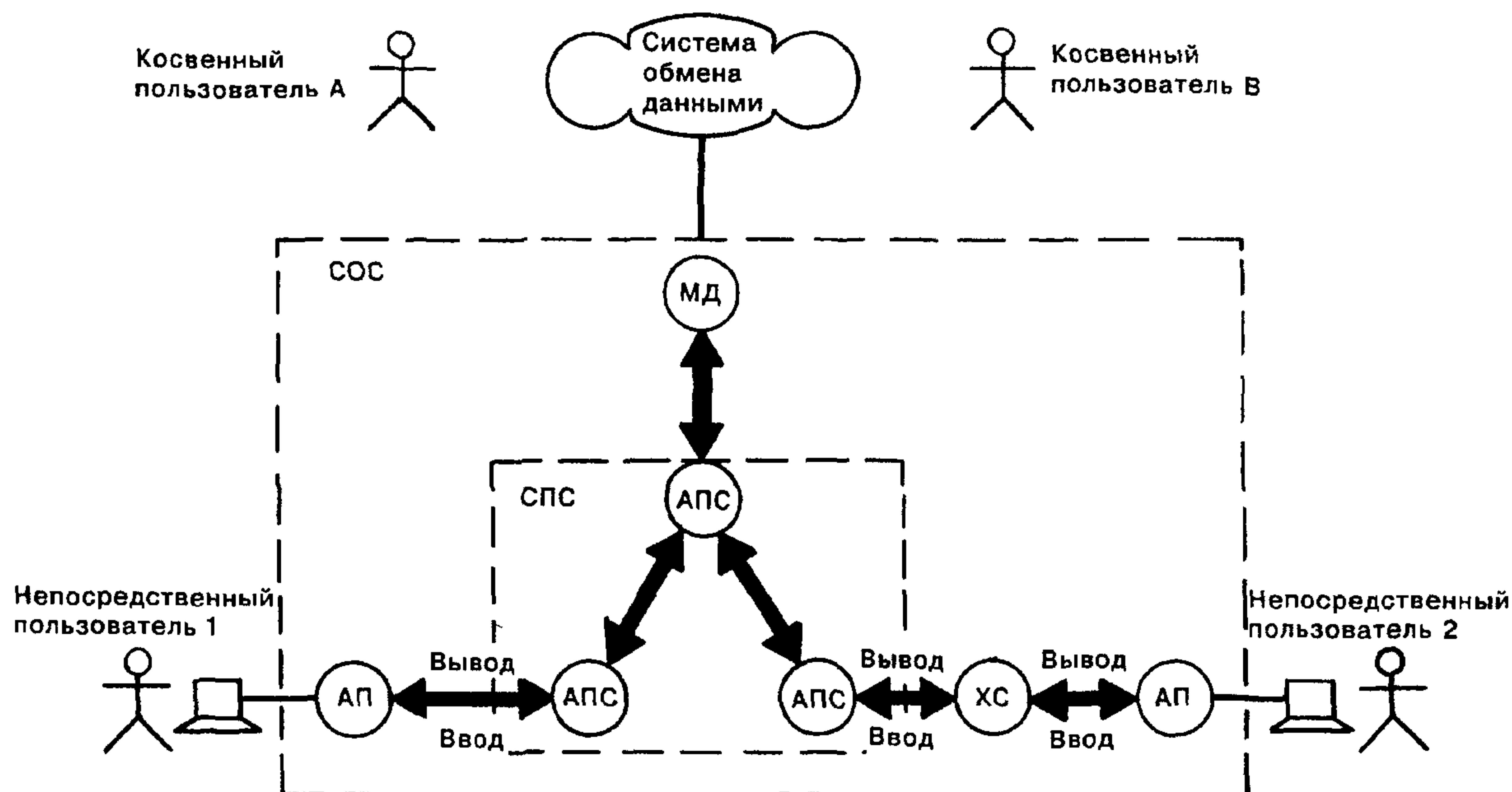
Рисунок 7 — Функциональные конфигурации, касающиеся использования ХС
