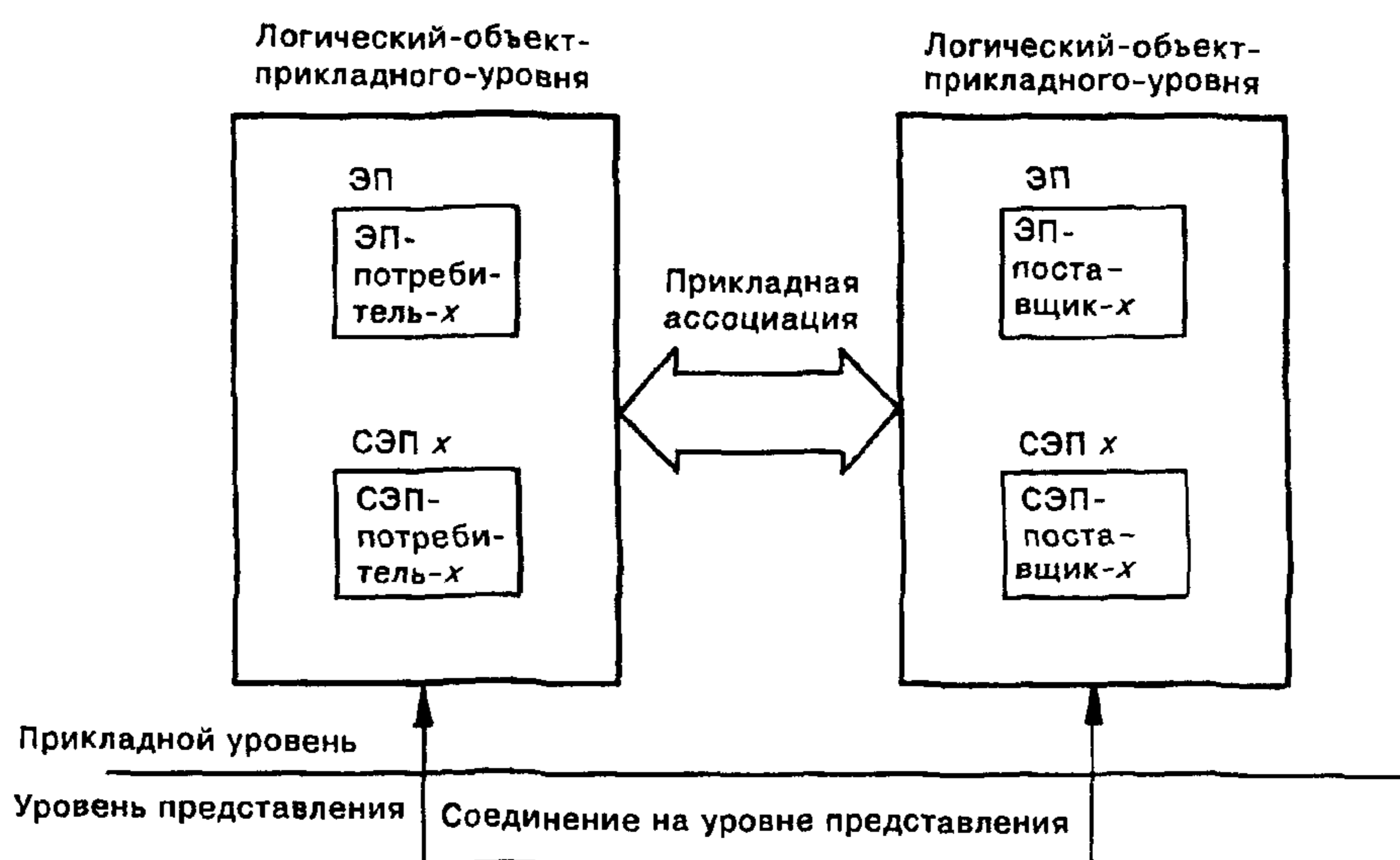
Рисунок 14 — Терминология асимметричных СЭП
