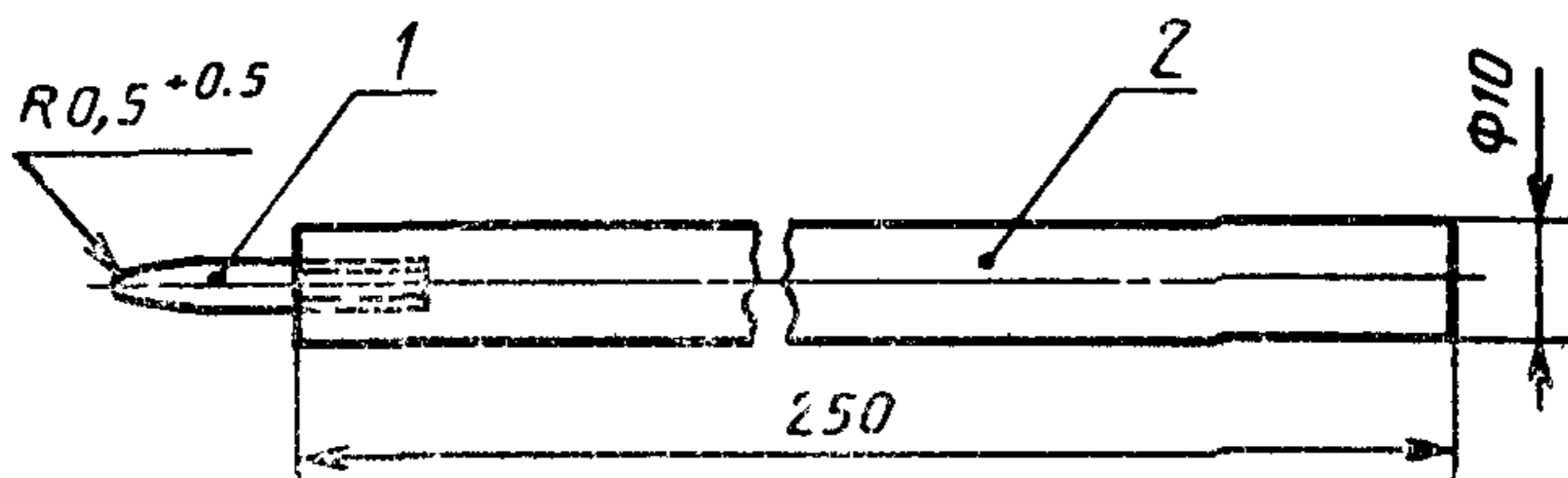
1 — пластмассовый наконечник; 2 — сталь Черт. 3
