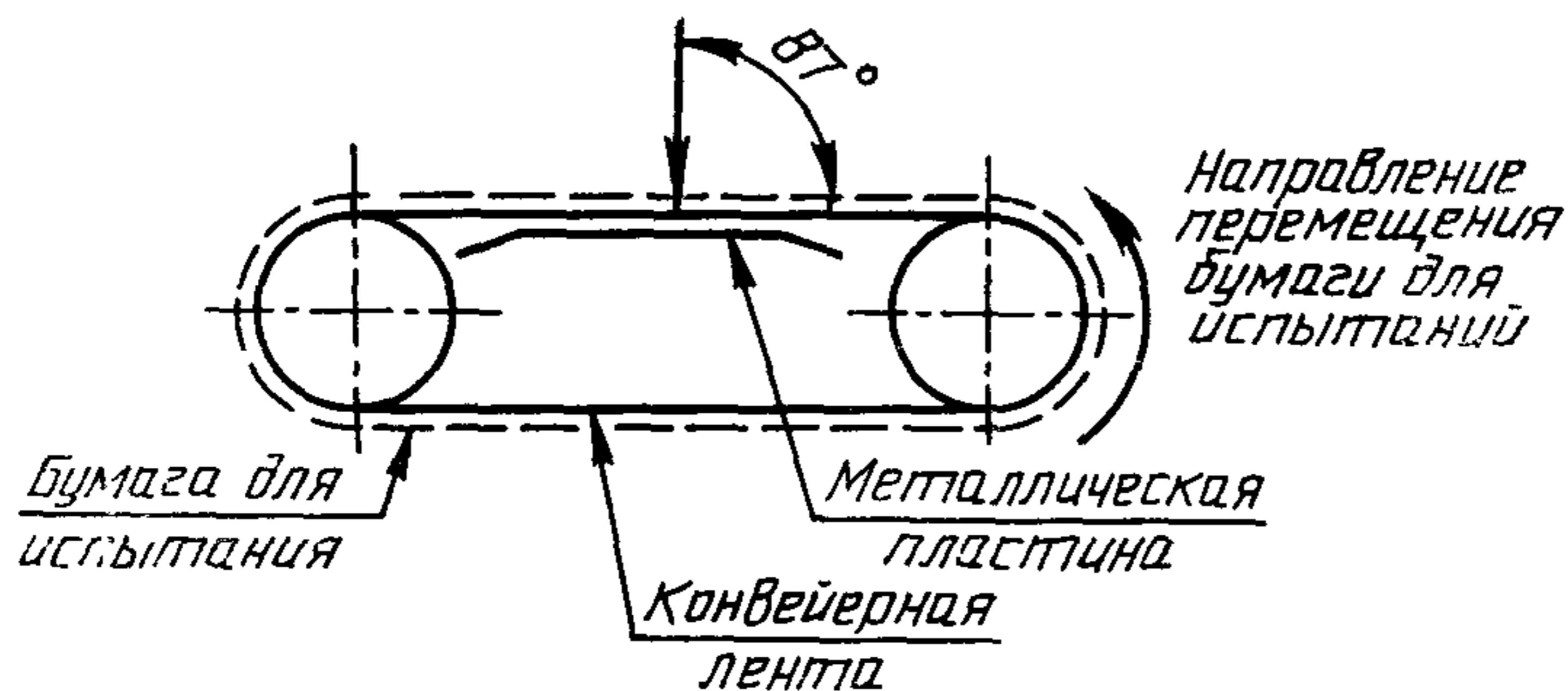
Рисунок 1 — Схема испытательного устройства
