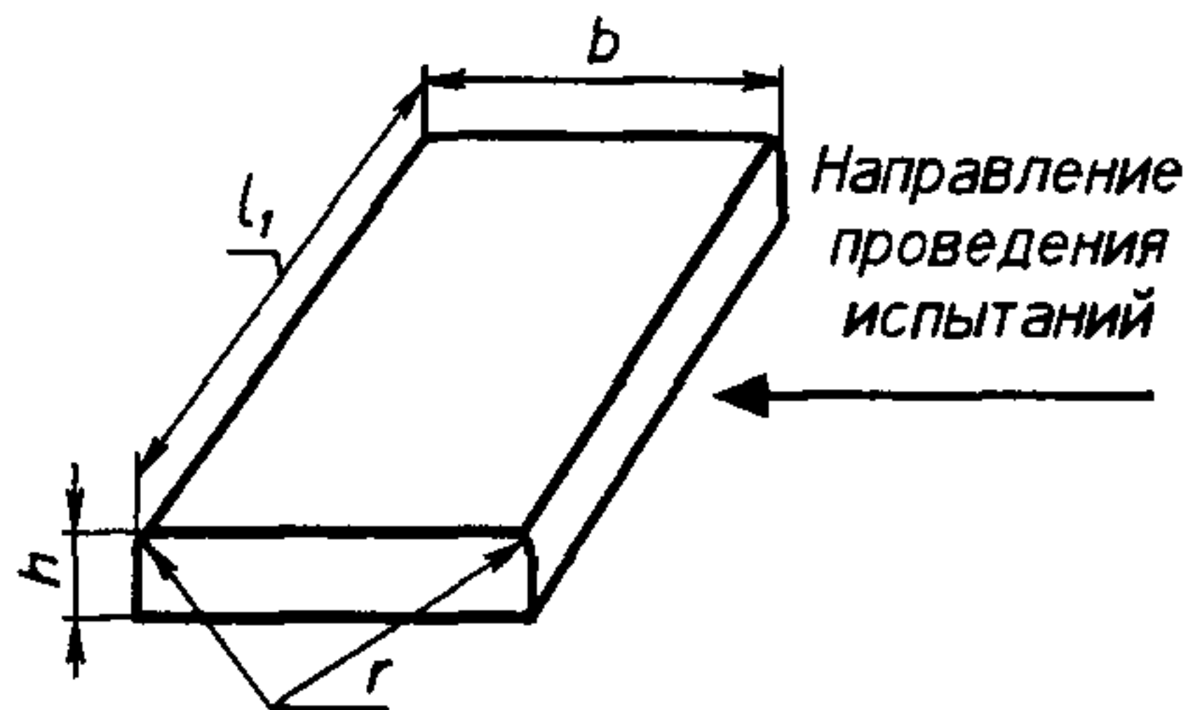
Рисунок 1 — Препятствие для проведения испытаний
