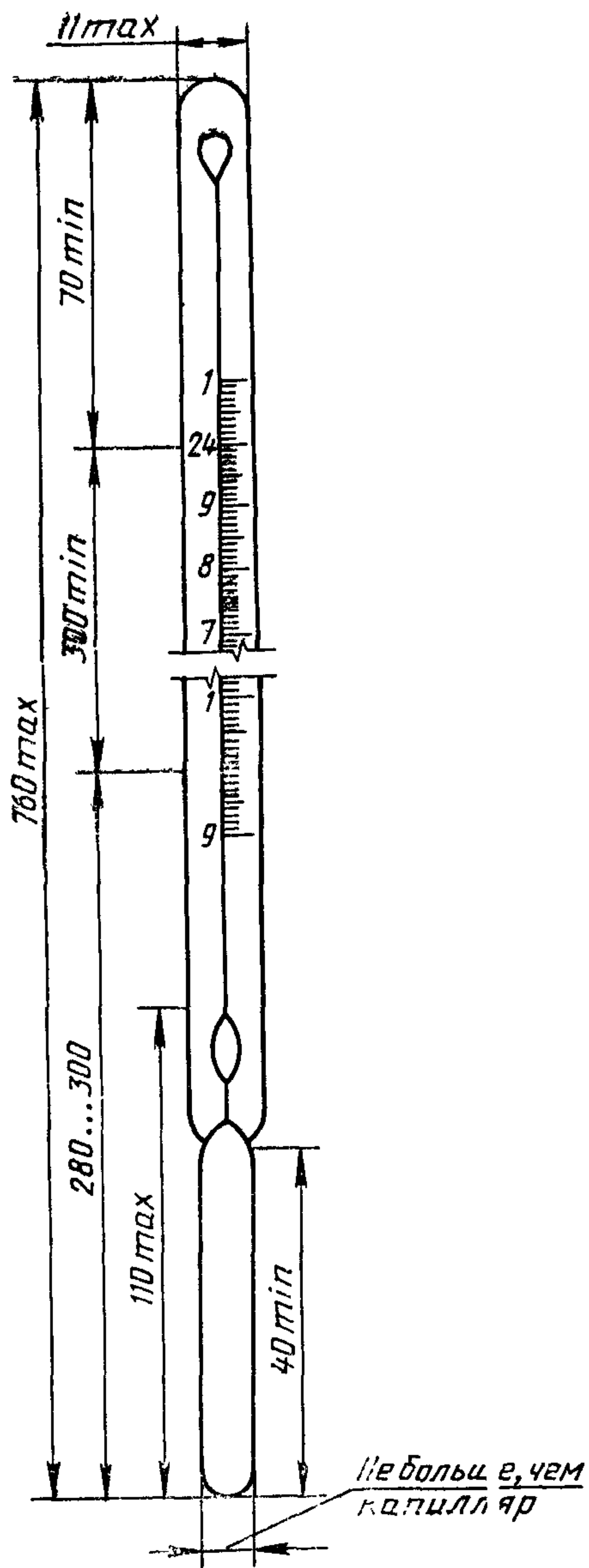
Рисунок 1 — Термометр палочный калориметрический
