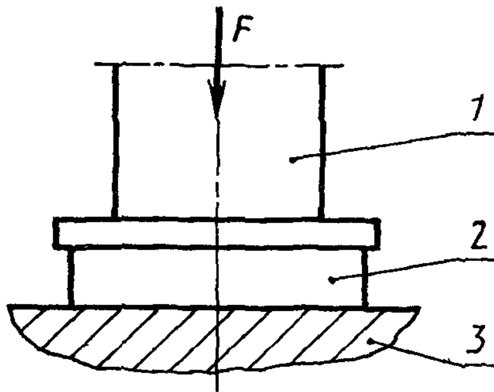
1 — плунжер; 2 — образец типа 3; 3 — нагревательная плита
