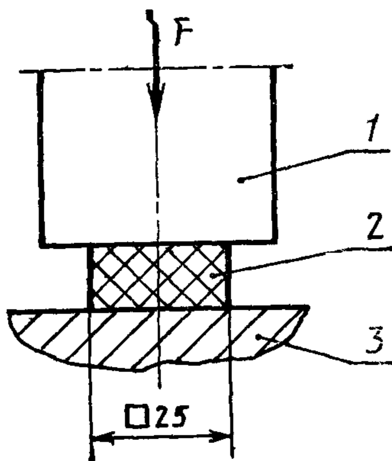
1 — силовой цилиндр (плунжер), 2 — образец типа 1; 3 — нагревательная плита
