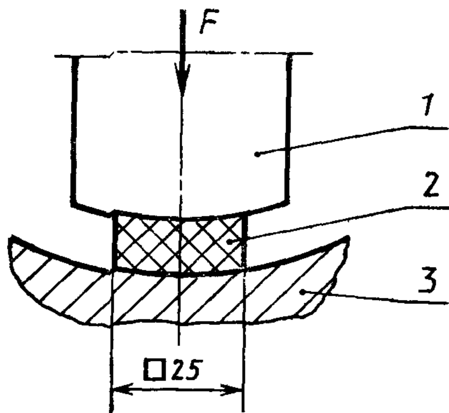
1 — силовой цилиндр (плунжер); 2 — образец типа 2, 3 — нагревательная плита
