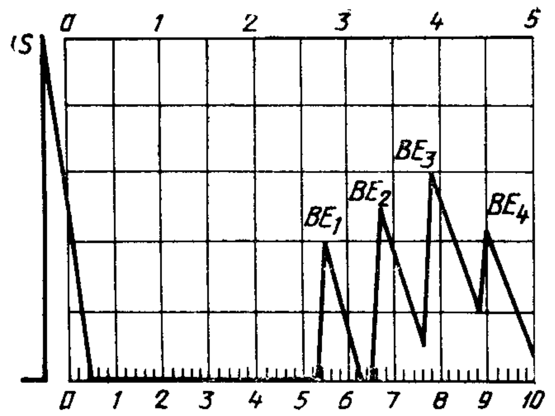
Удовлетворительное соединение (преобразователь с двумя кристаллами)
