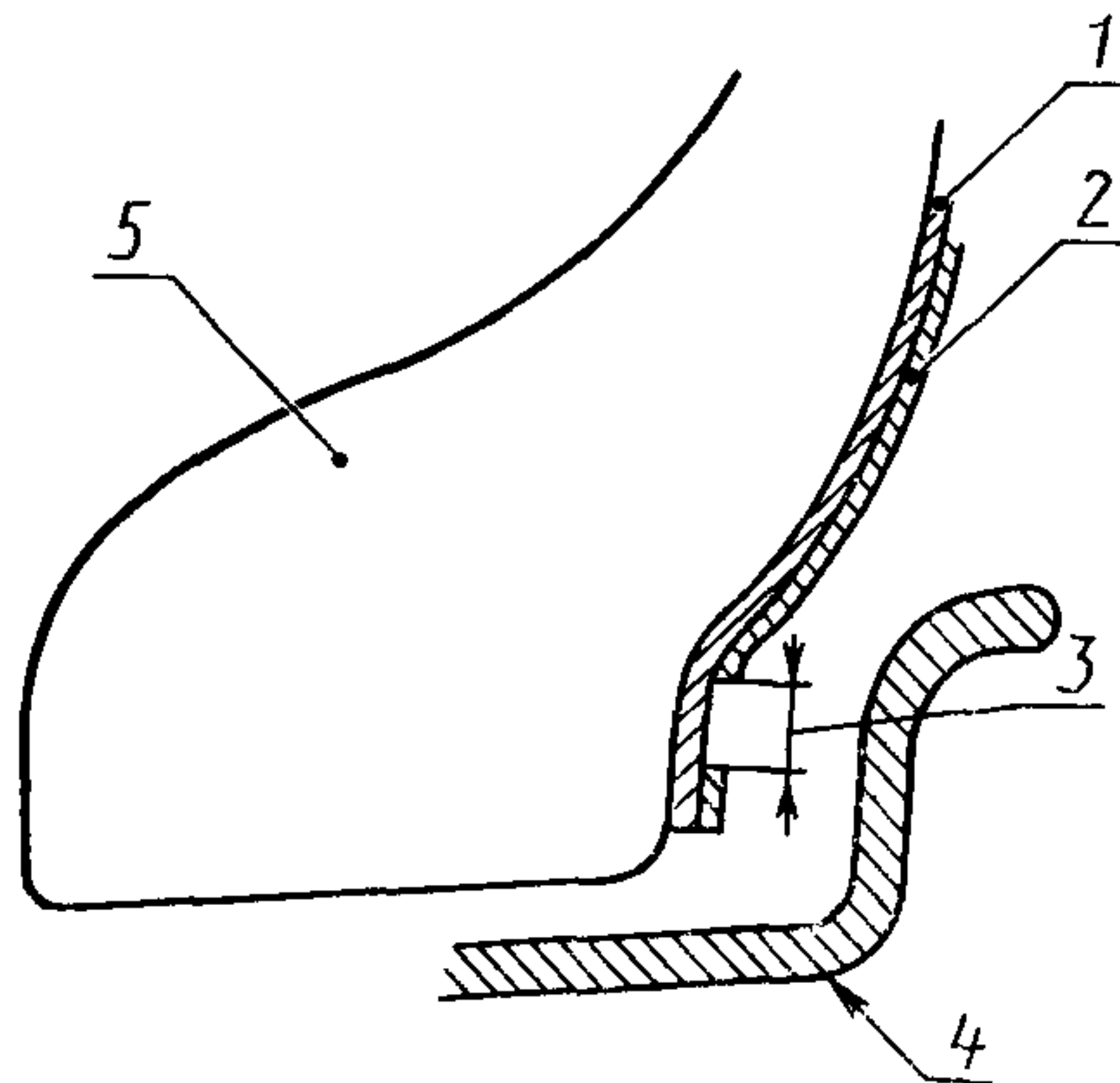
Давление посадки на обод — электрический метод
