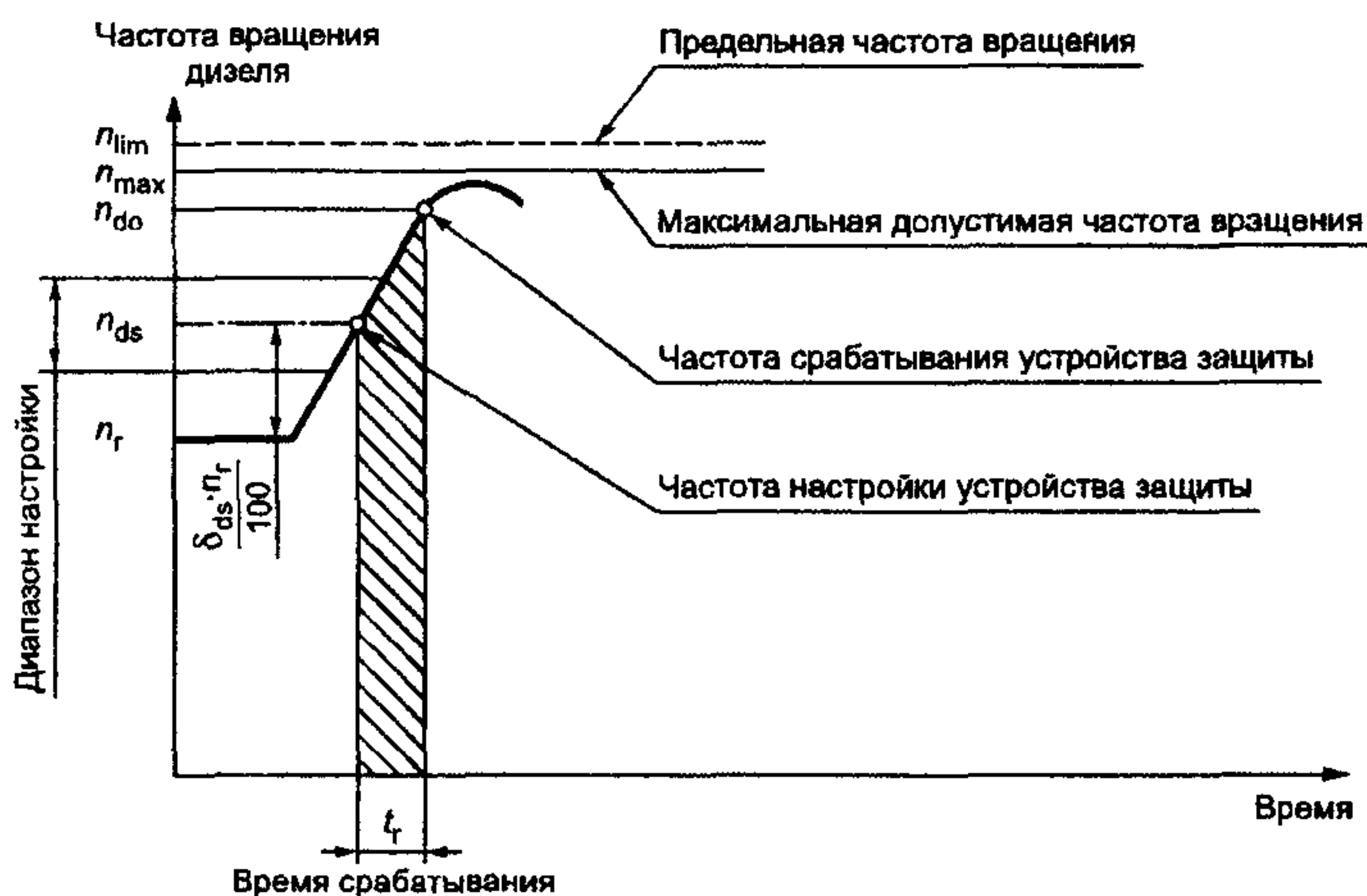
Рисунок 1 — Типичная кривая срабатывания устройства защиты
