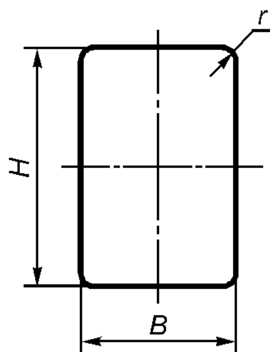
Рисунок В.1 — Размеры прямоугольных знаков вертикального формата
