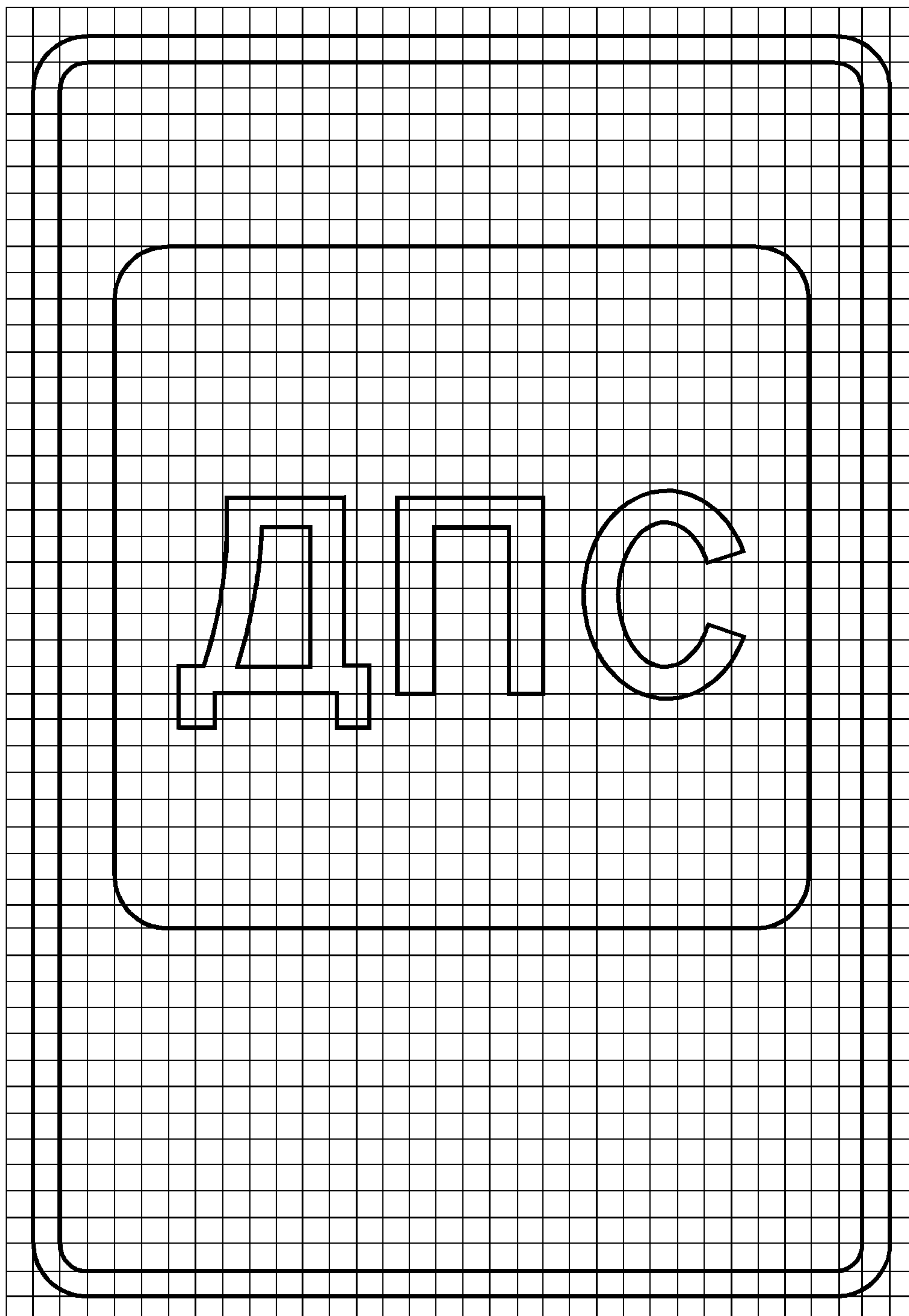
Рисунок Б.2 — Знак 6.14
