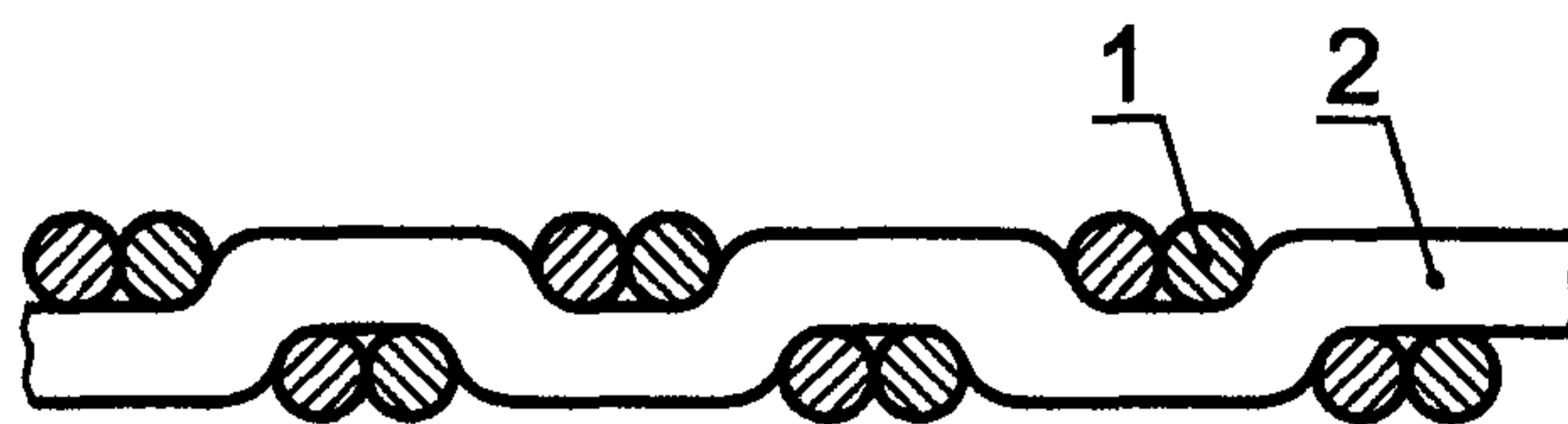
1 — нить основы ворсованная, 2 — нить утка ворсованная
