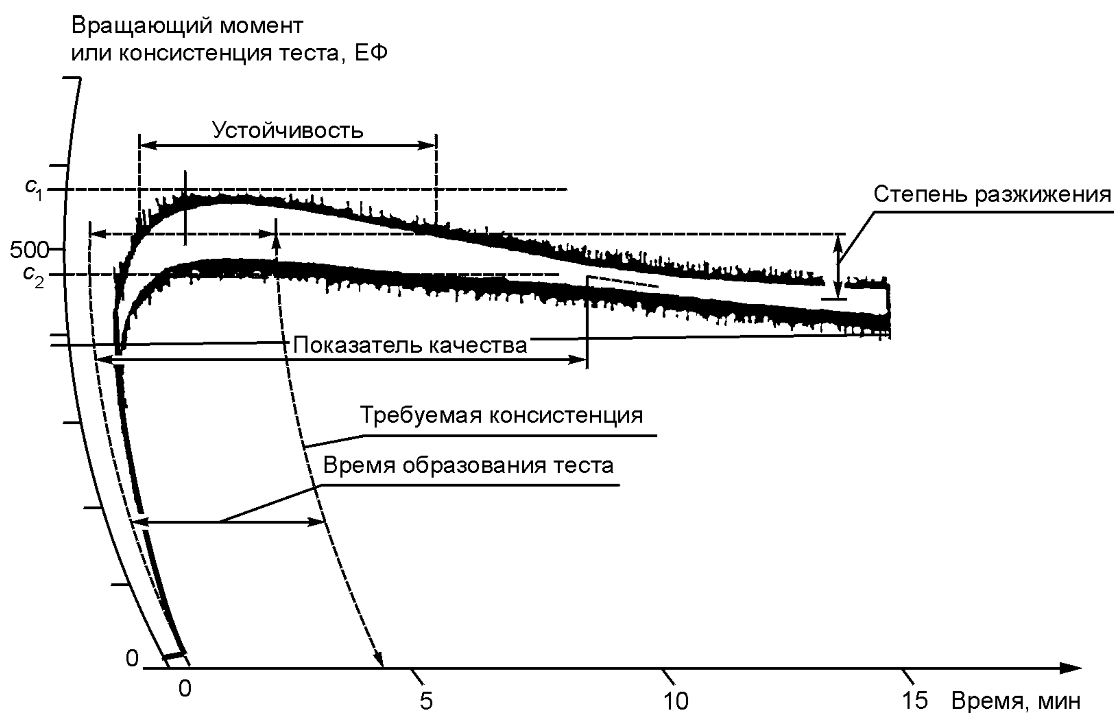
Рисунок 1 — Репрезентативная фаринограмма, показывающая измеряемые показатели
