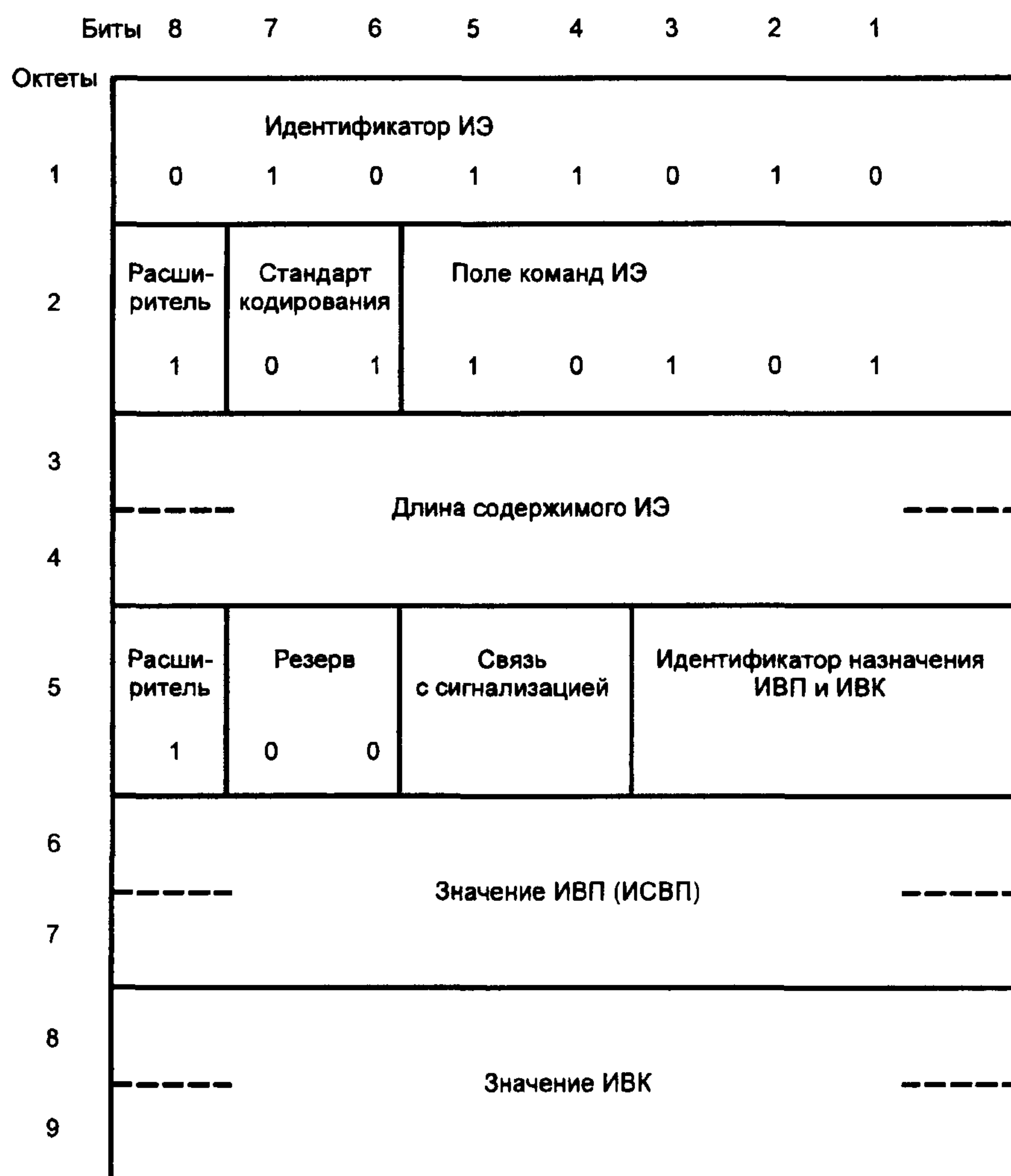
Рисунок 11 — Формат ИЭ «Идентификатор виртуального соединения»
