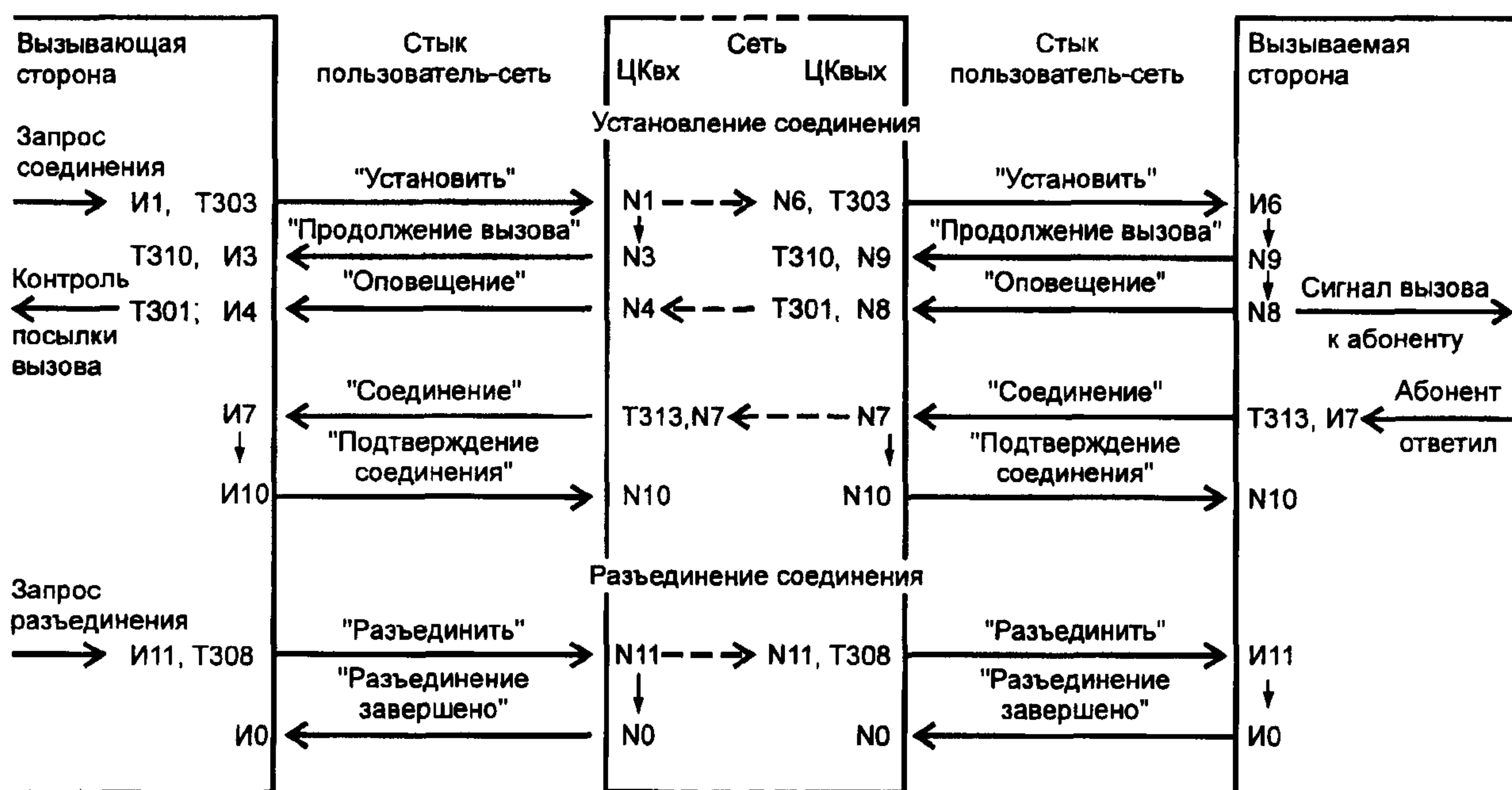
Рисунок 18 — Последовательность передачи сообщений
