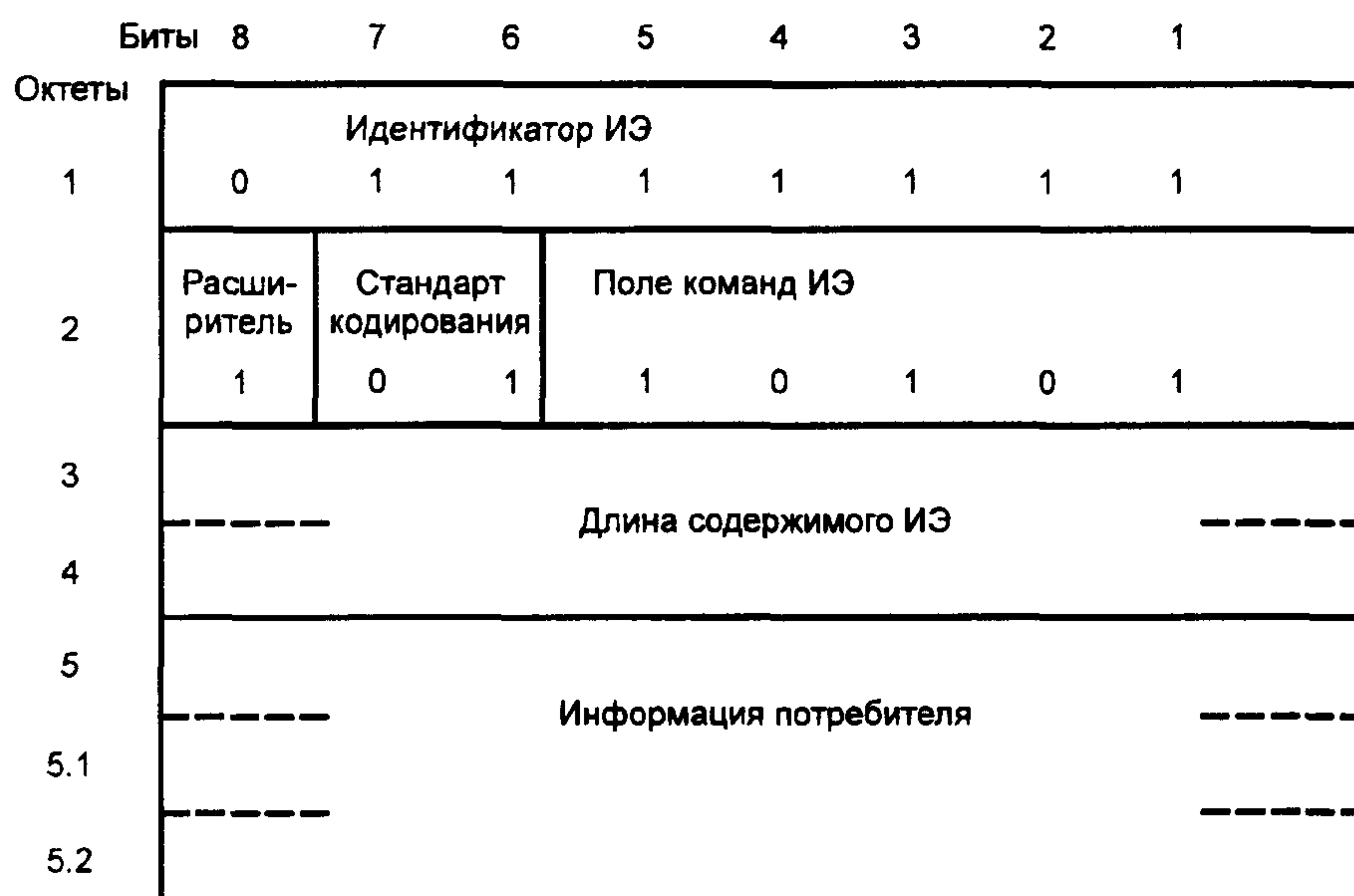
Рисунок 17 — Формат ИЭ «Информация потребитель—потребитель»
