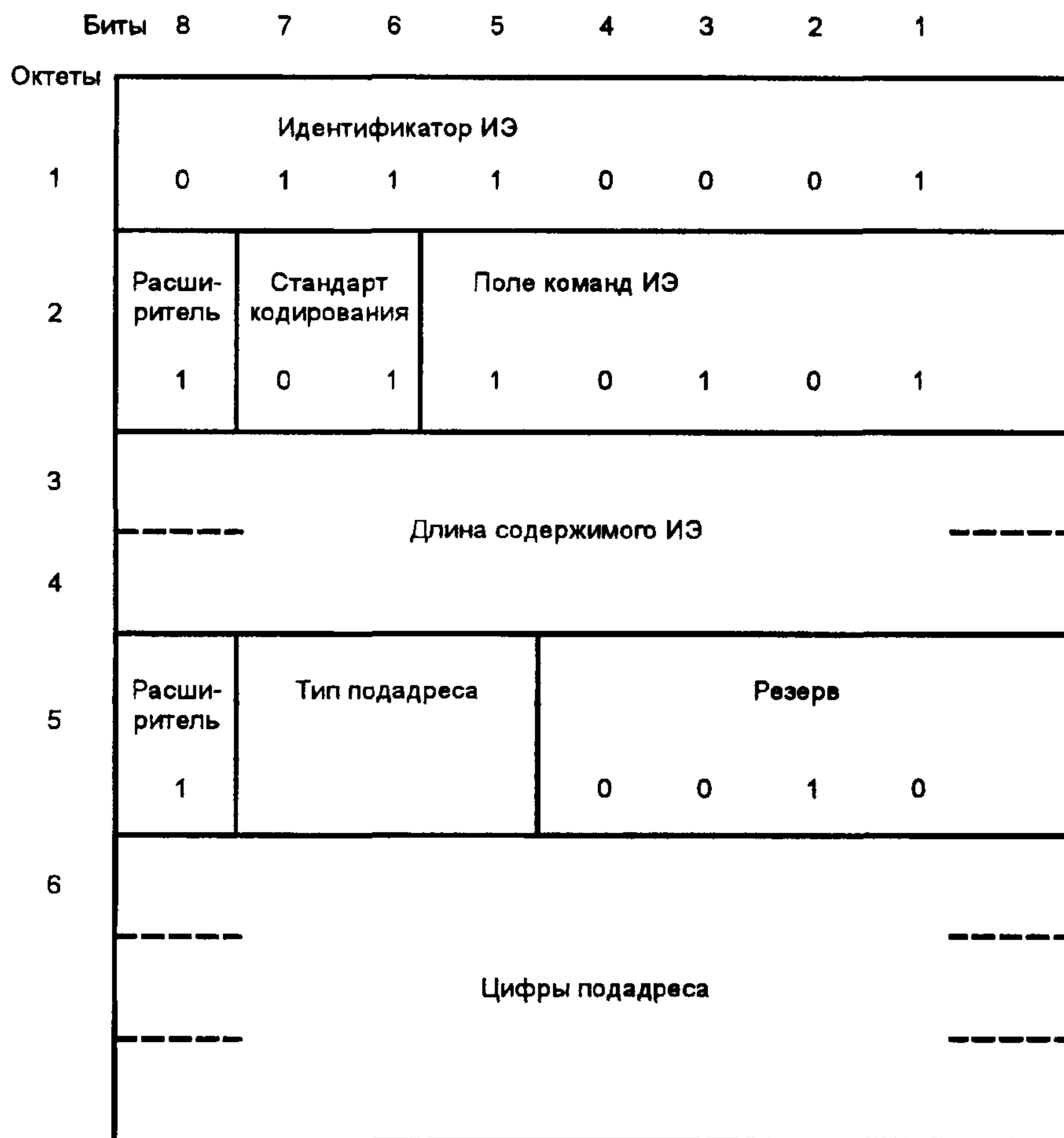
Рисунок 10 — Формат ИЭ «Субадрес вызываемой стороны»
