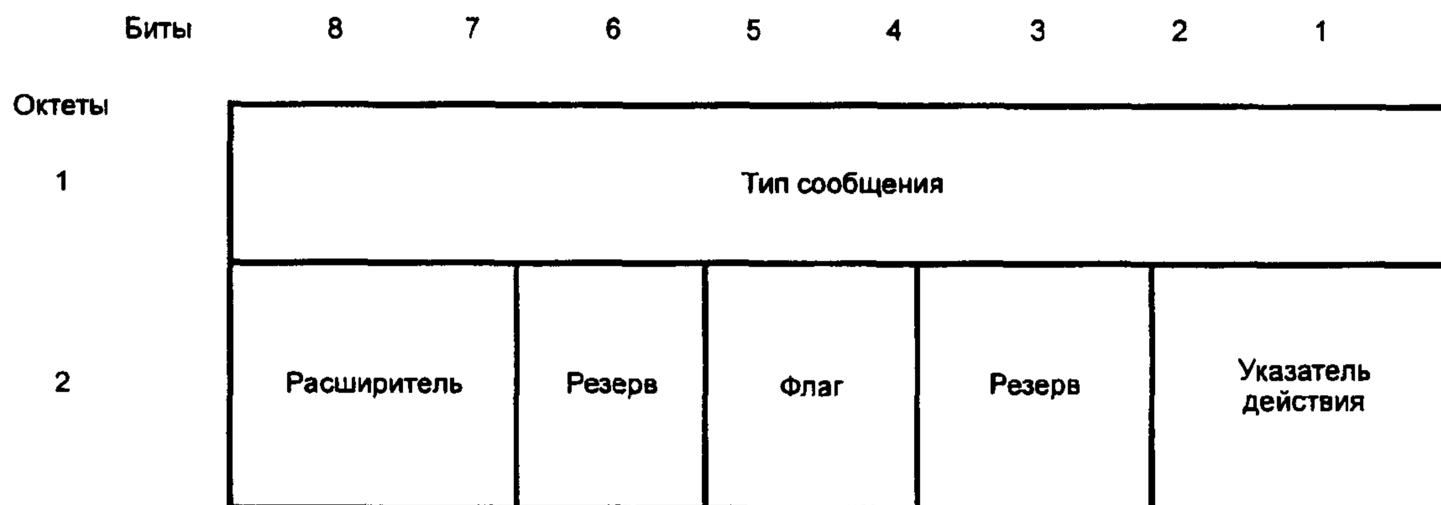
Рисунок 2 — Структура поля «Тип сообщения»
