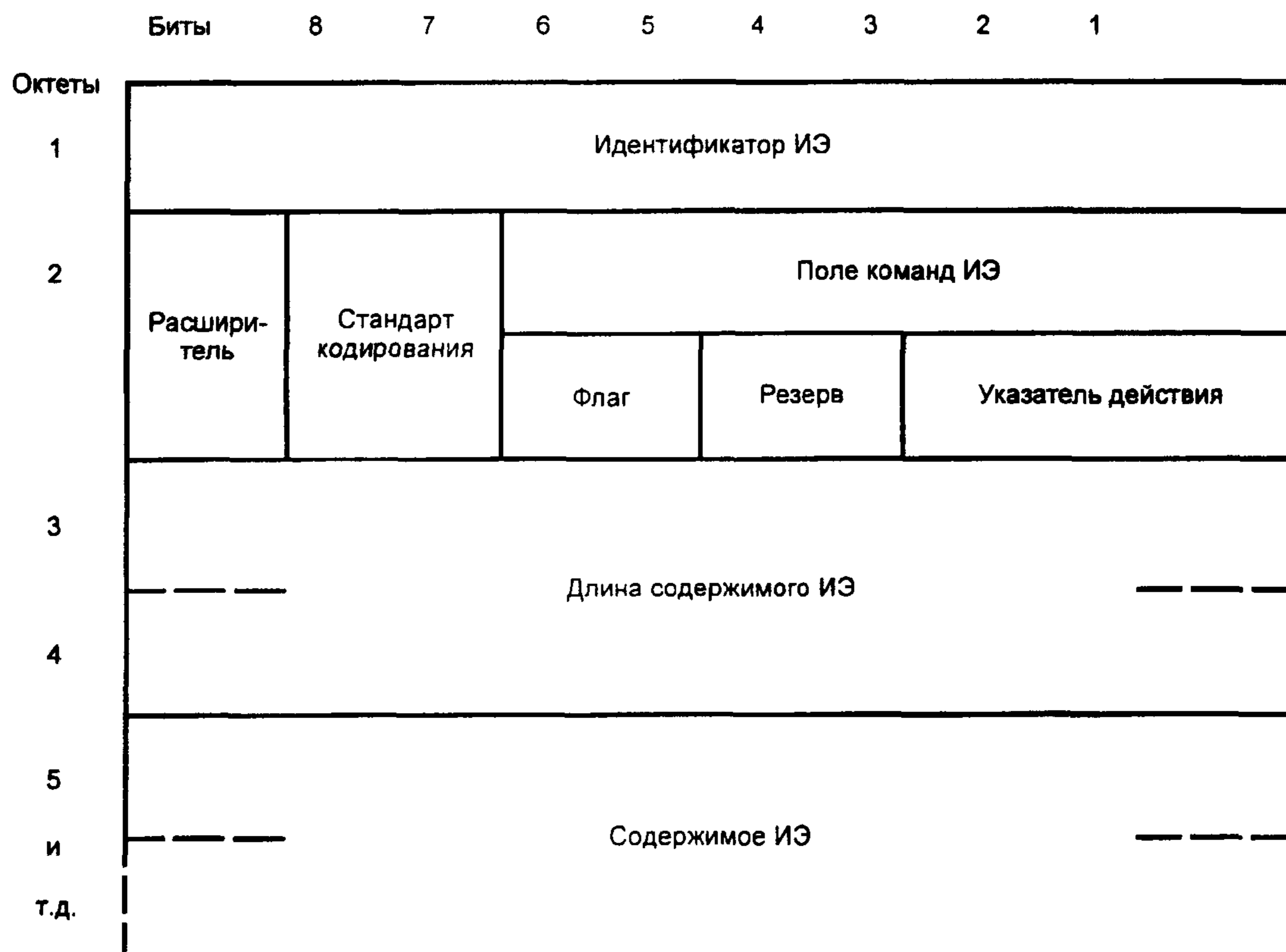
Рисунок 3 — Структура формата ИЭ
