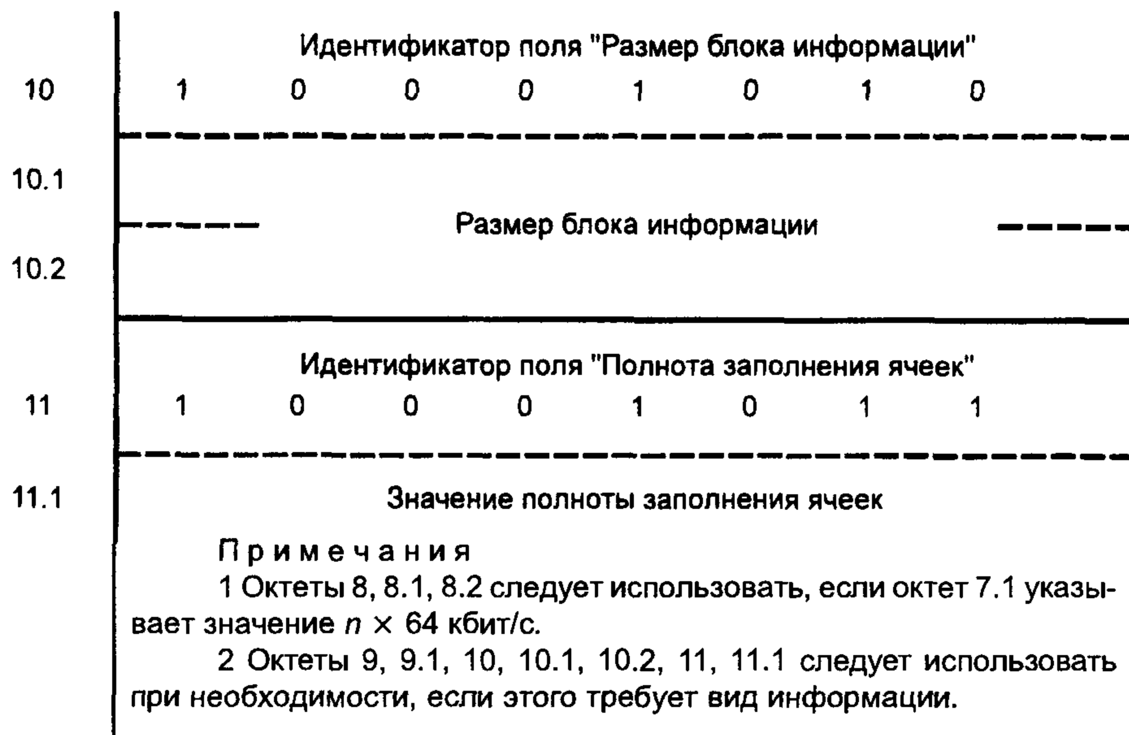
Рисунок 4 — Формат ИЭ «Параметры уровня адаптации» типа 1
