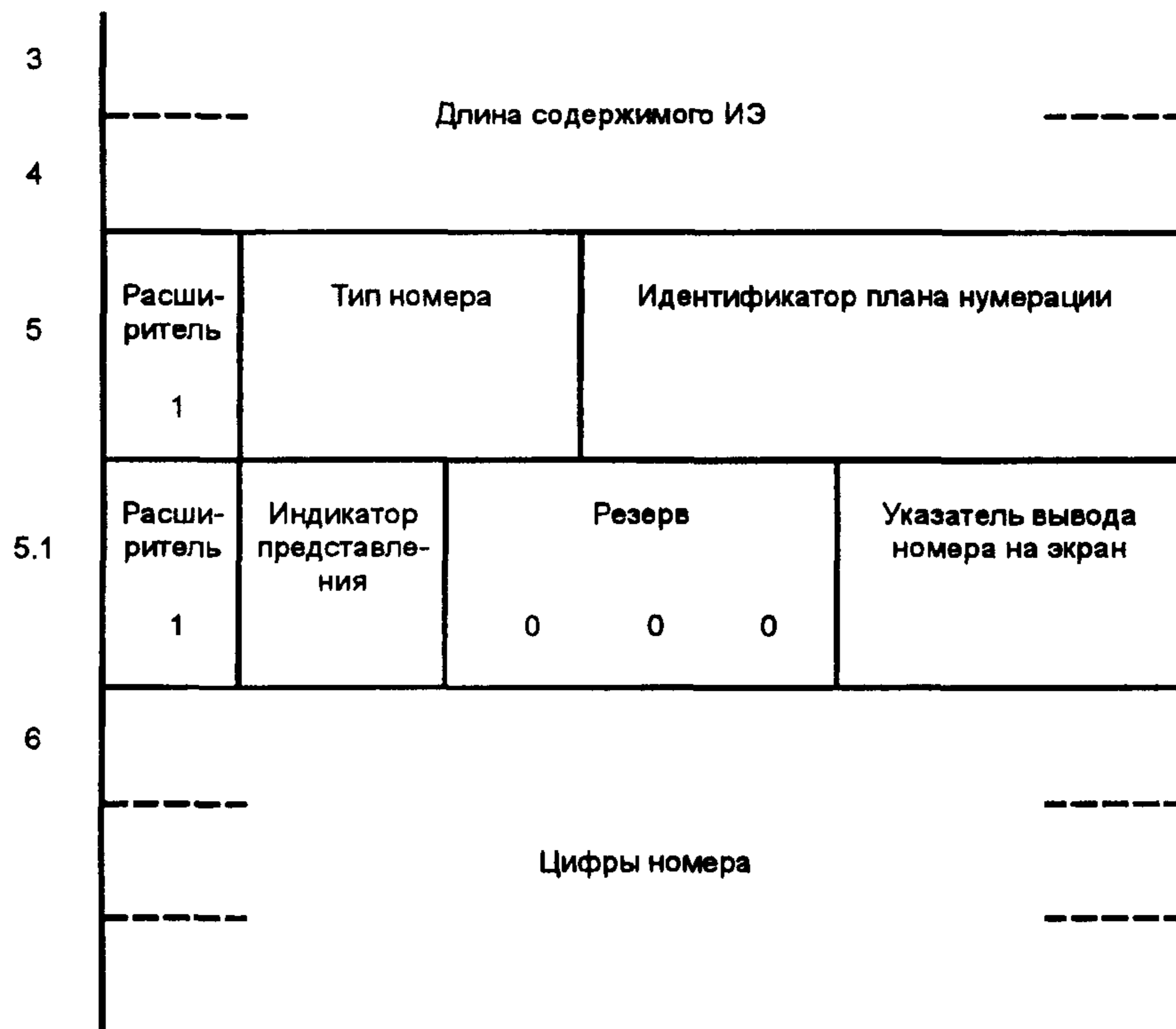
Рисунок 9 — Формат ИЭ «Номер вызывающей стороны»
