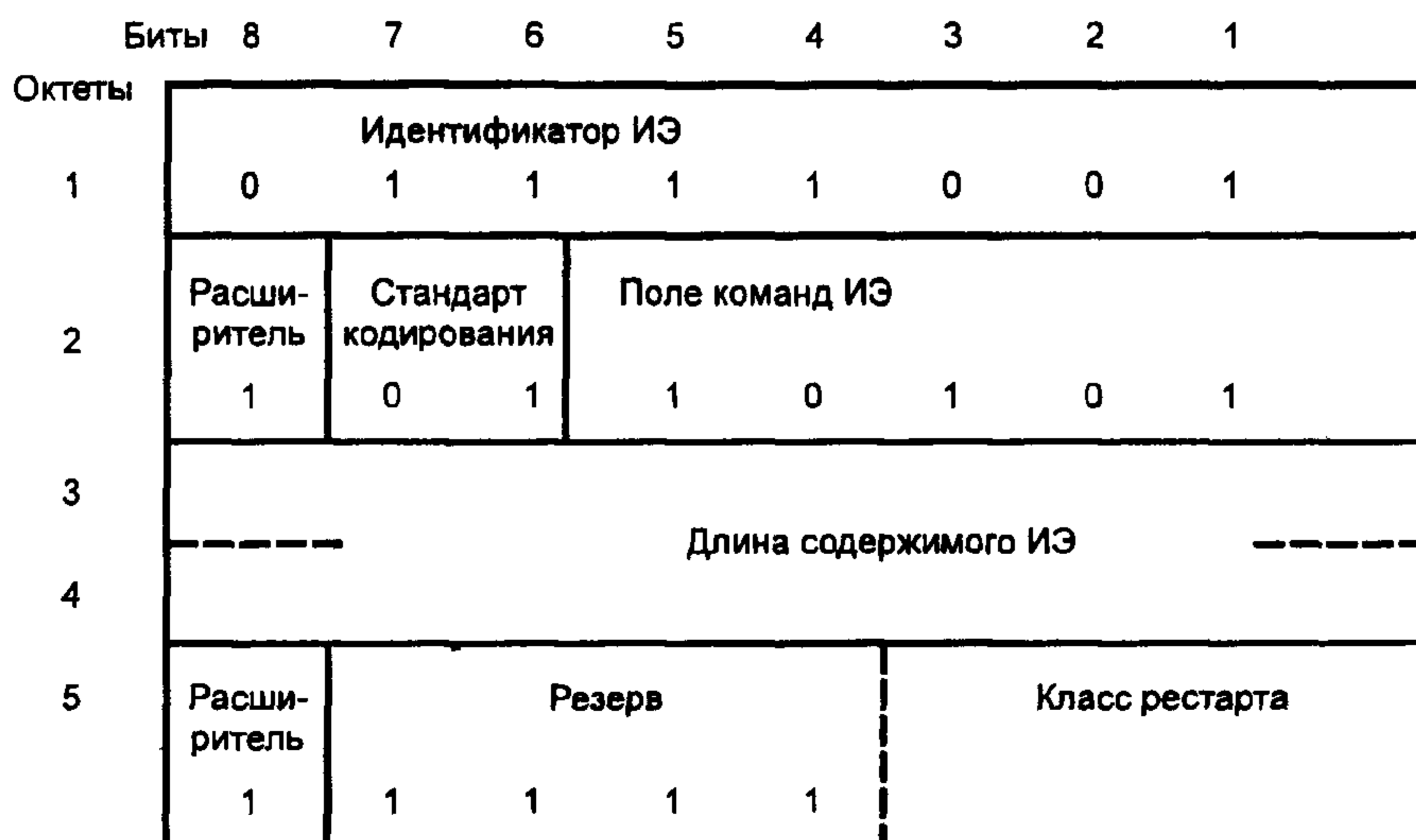
Рисунок 16 — Формат ИЭ «Индикатор рестарта»
