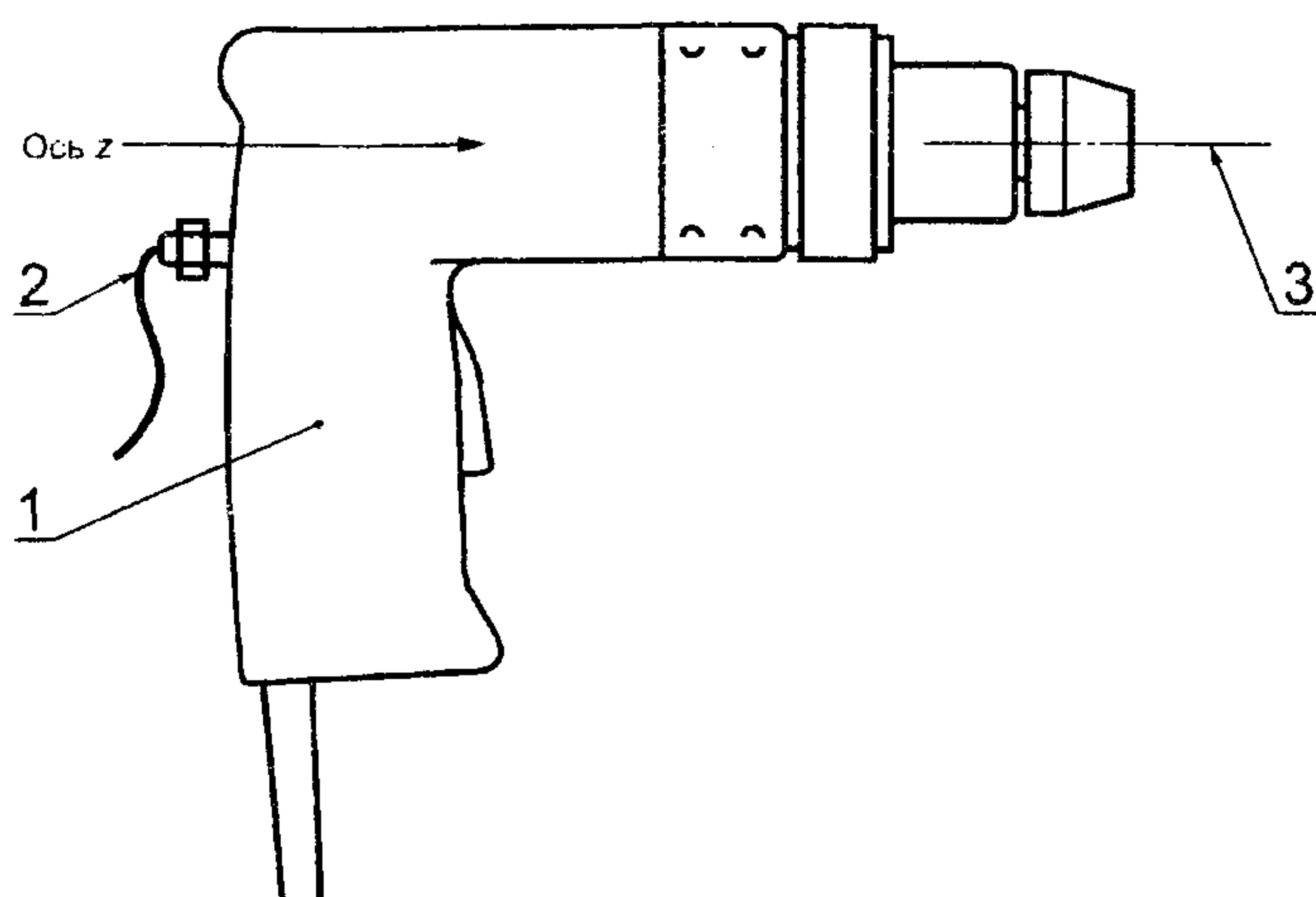
Рисунок 1 — Направление измерений, пример расположения и крепления вибропреобразователя
