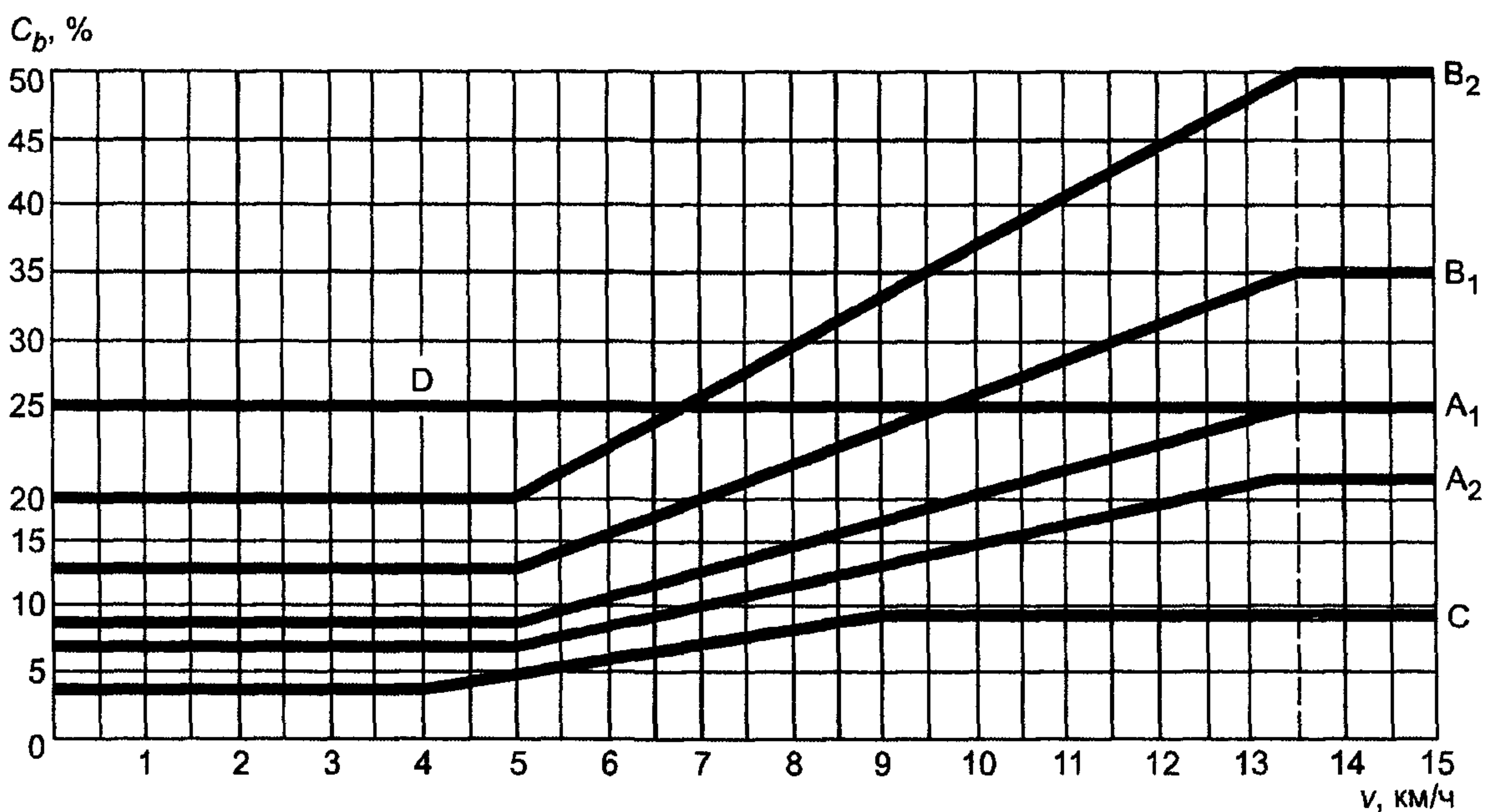
Рисунок 1 — График зависимости коэффициента торможения от скорости машины
