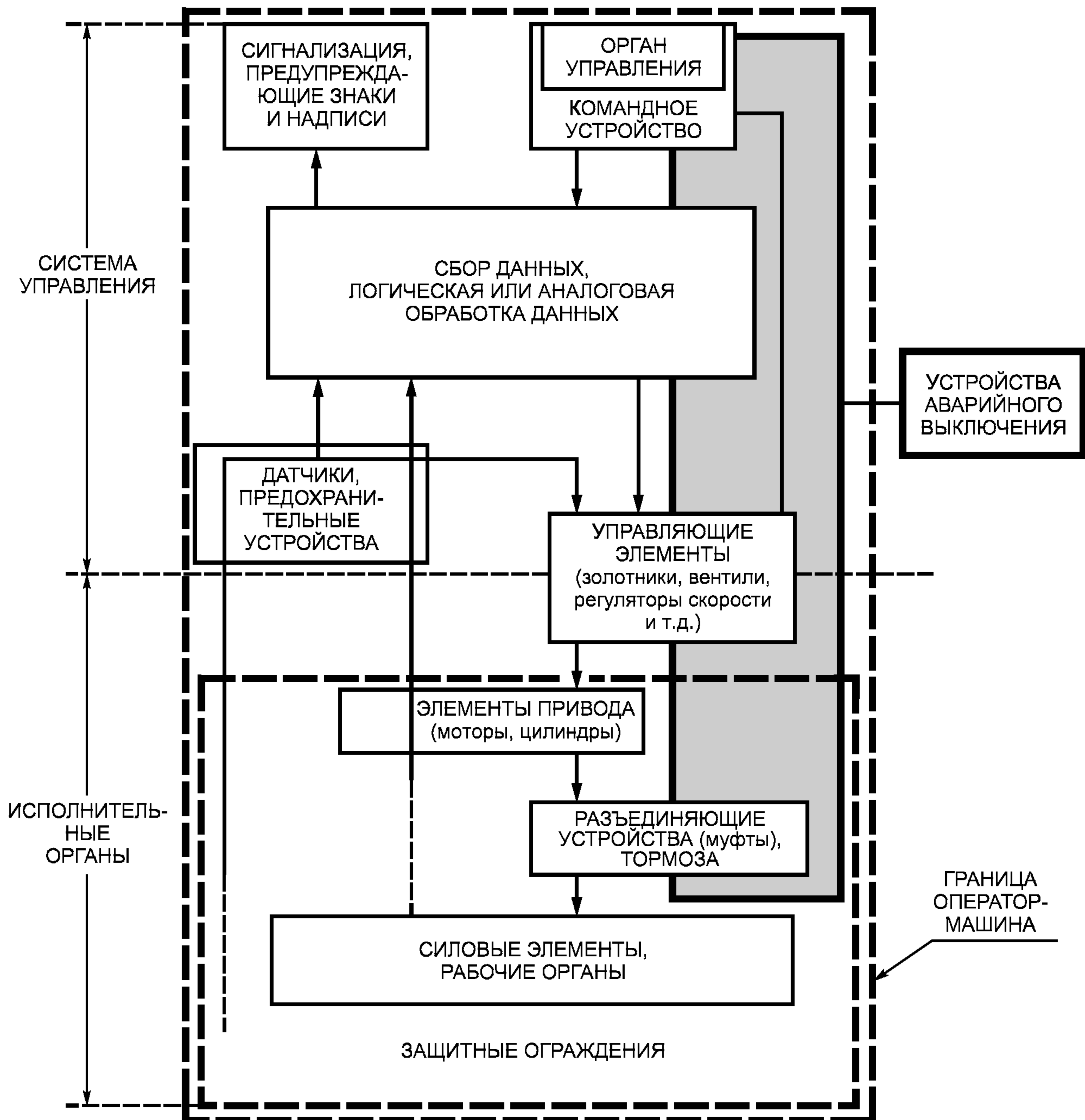
Рисунок 2 — Устройства аварийного отключения машины/сооружения
