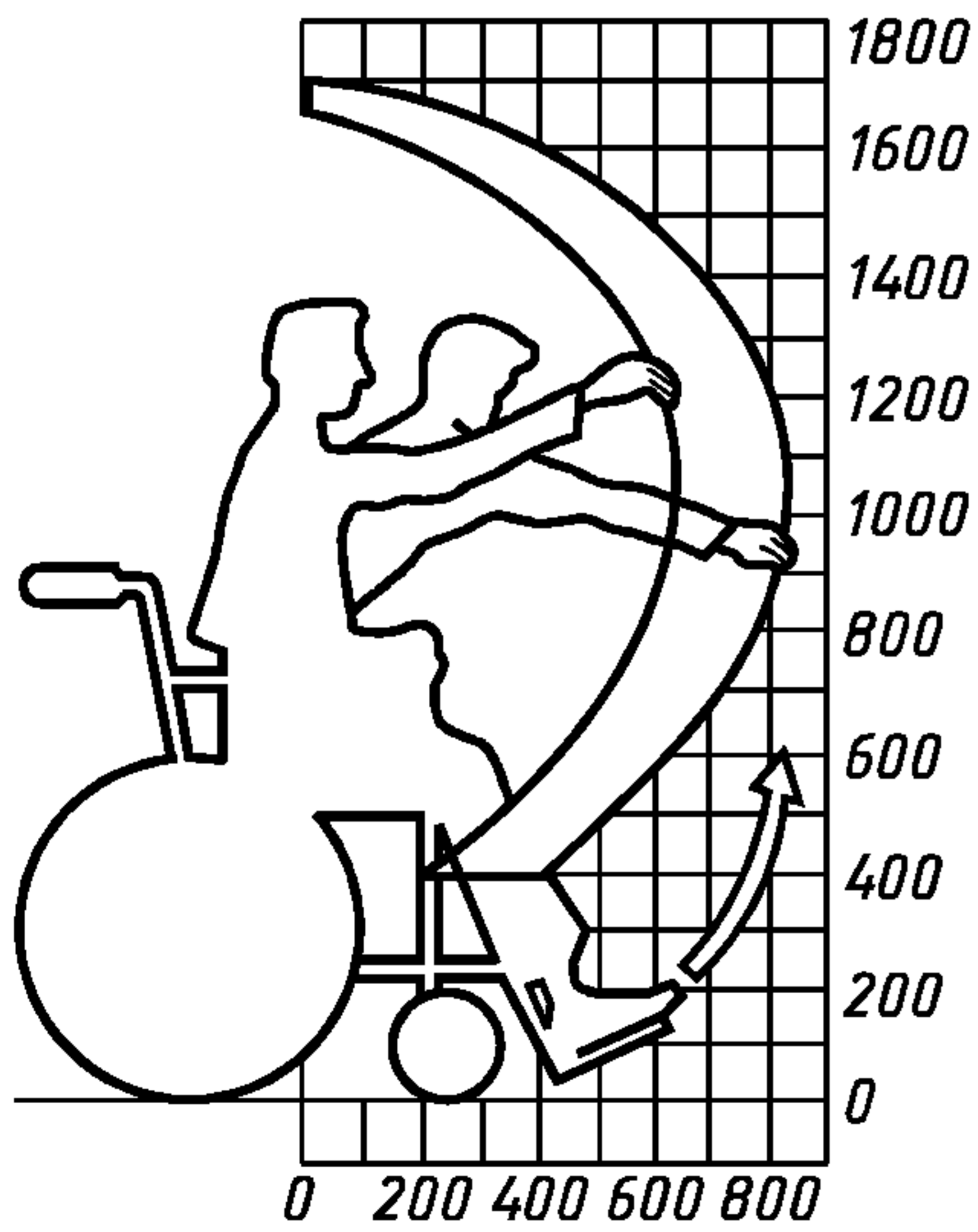
Рисунок Б.1 — Зона досягаемости для инвалидов-мужчин в кресле-коляске
