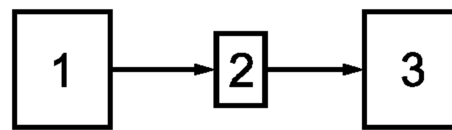
1 — панорамный измеритель КСВН; 2 — рефлектометр на проверяемую полосу частот; 3 — антенна
