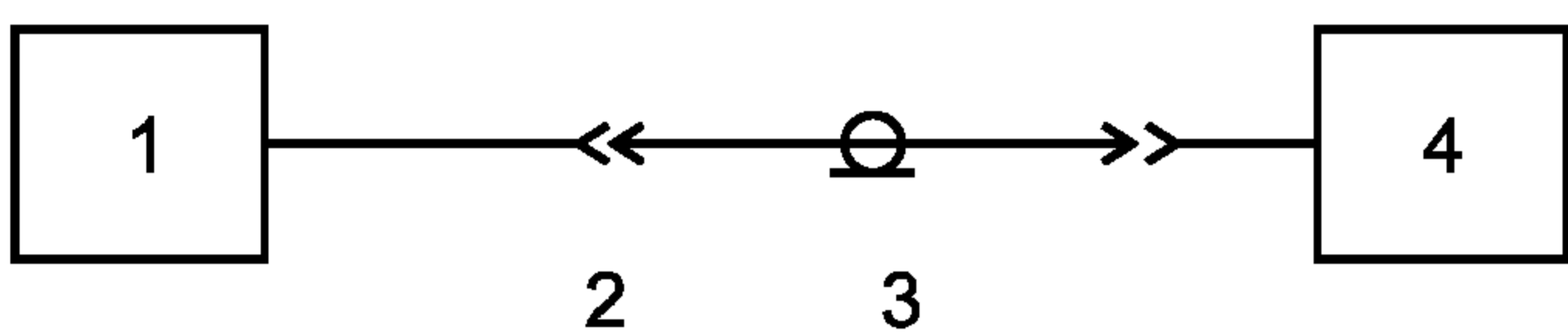
1 — измеритель КСВН; 2 — коаксиальный переход; 3 — фидер антенны; 4 — антенна
