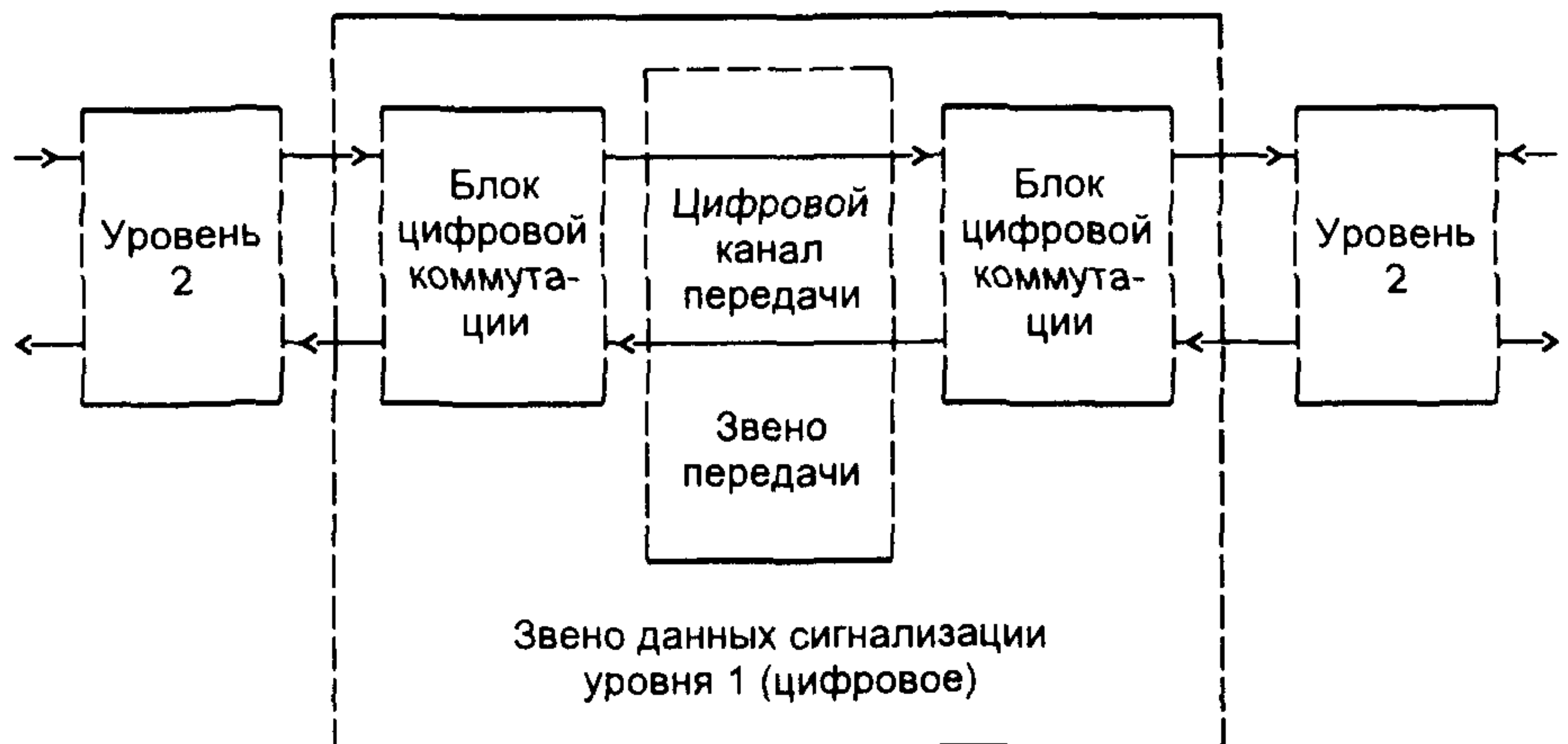
Рисунок 7.1 — Функциональная конфигурация звена данных сигнализации
