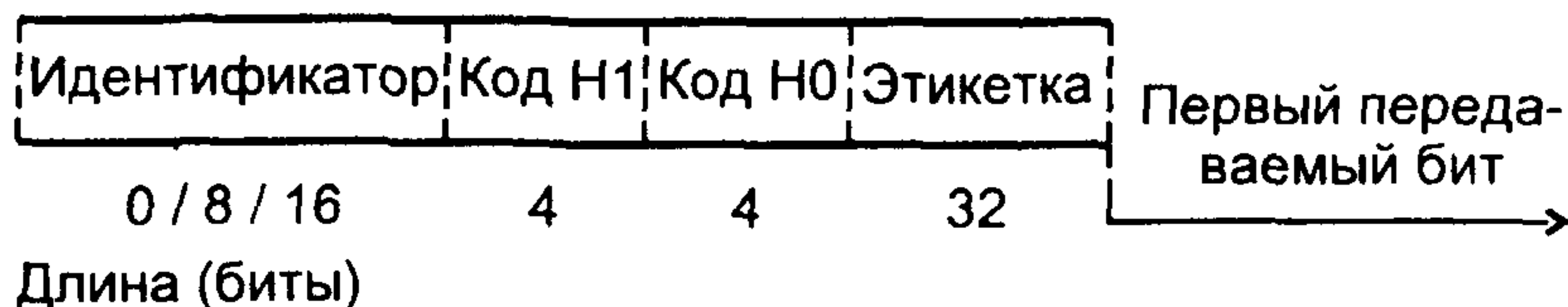
Рисунок 9.4 — Формат сообщений управления сетью сигнализации
