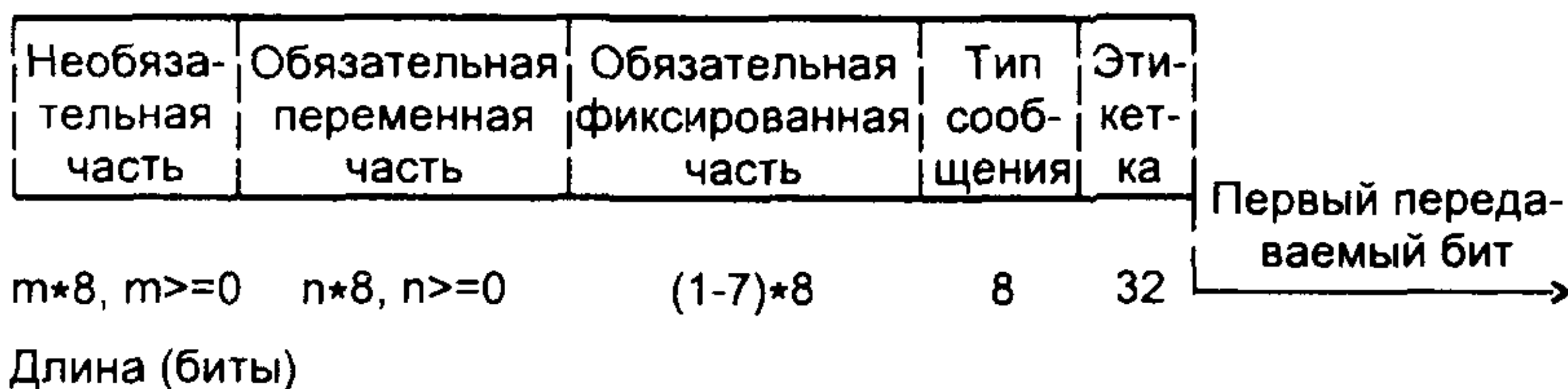
Рисунок 9.3 — Формат сообщений ПУСС
