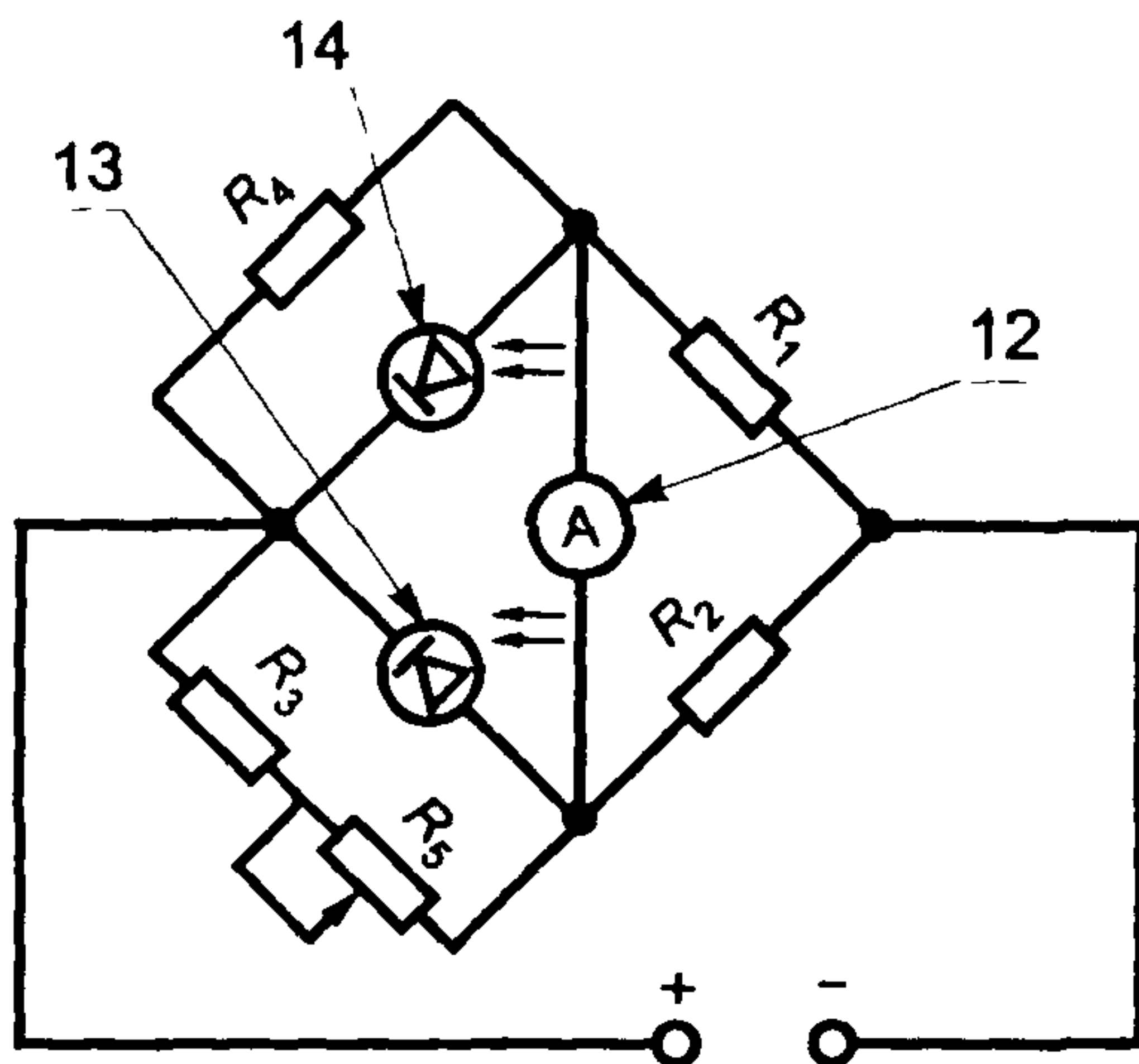
12 — регистрирующее устройство; 13, 14 — приемник
