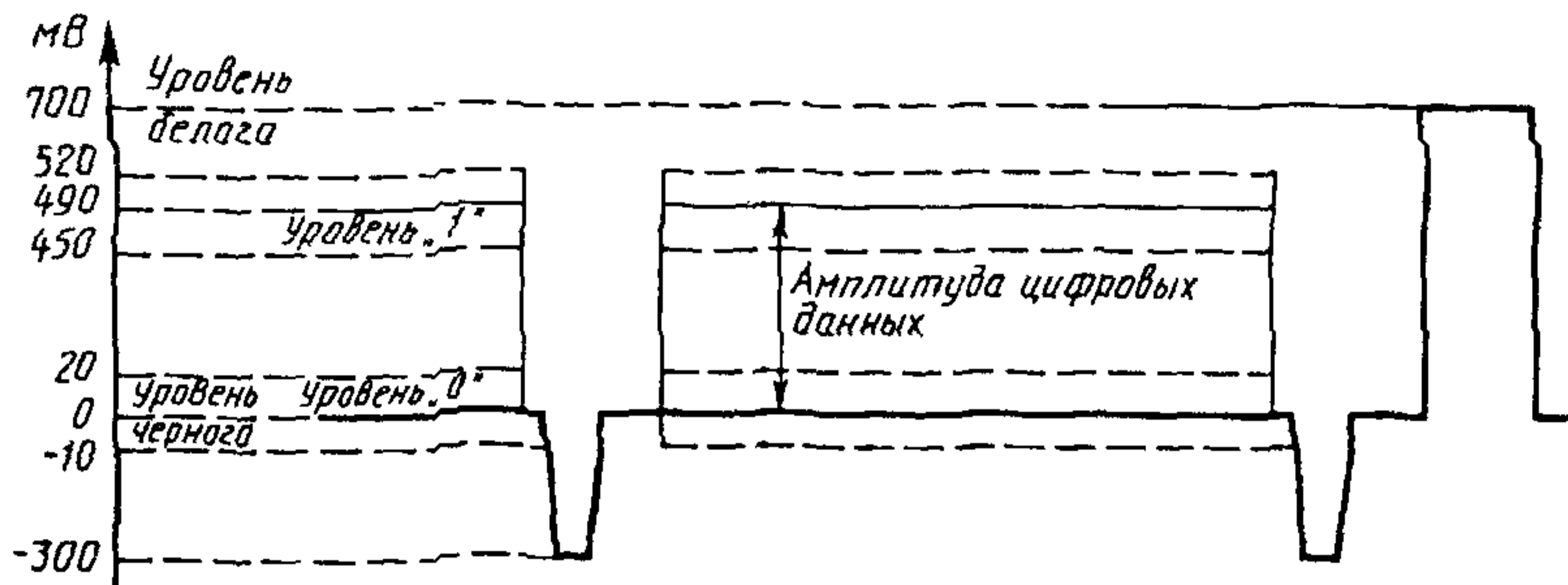
Рисунок 2 — Уровни сигнала цифровых данных сигнала телетекста
