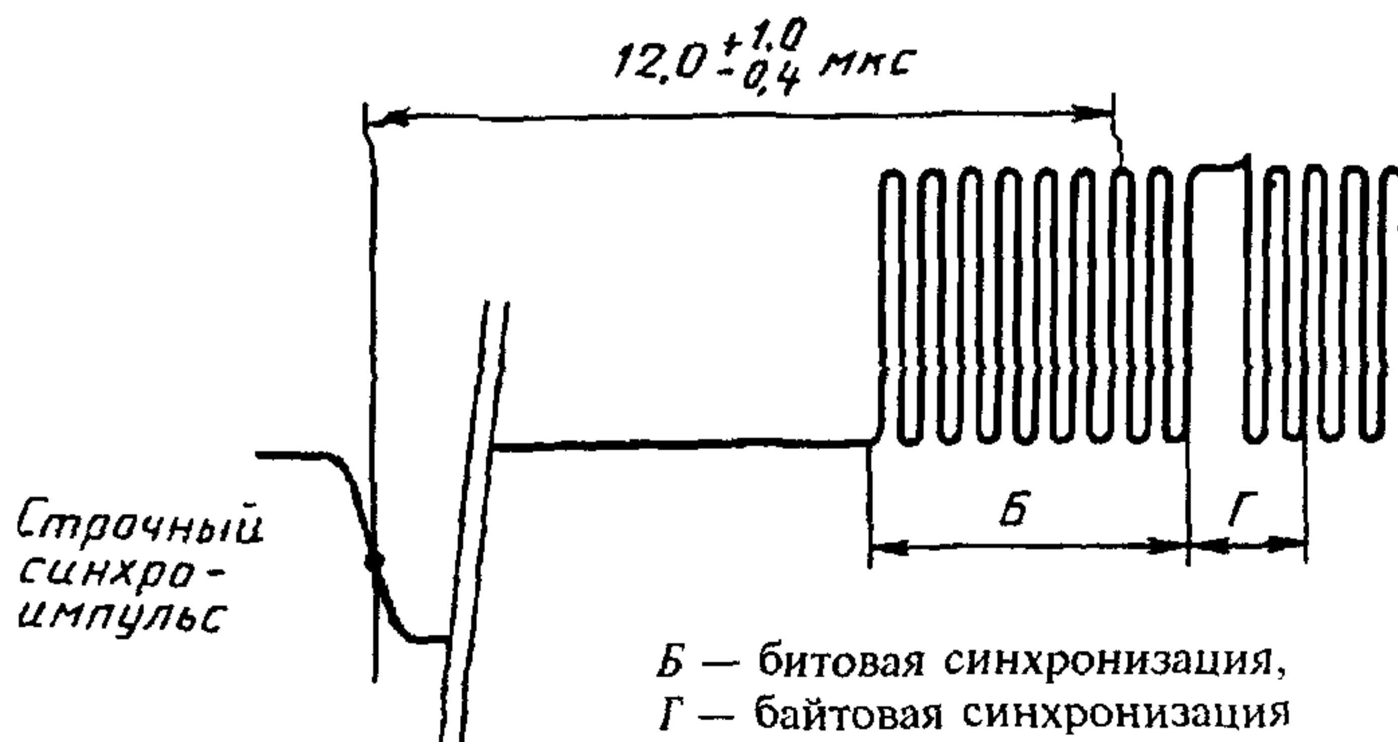
Рисунок 3 — Синхронизация сигнала цифровых данных телетекста
