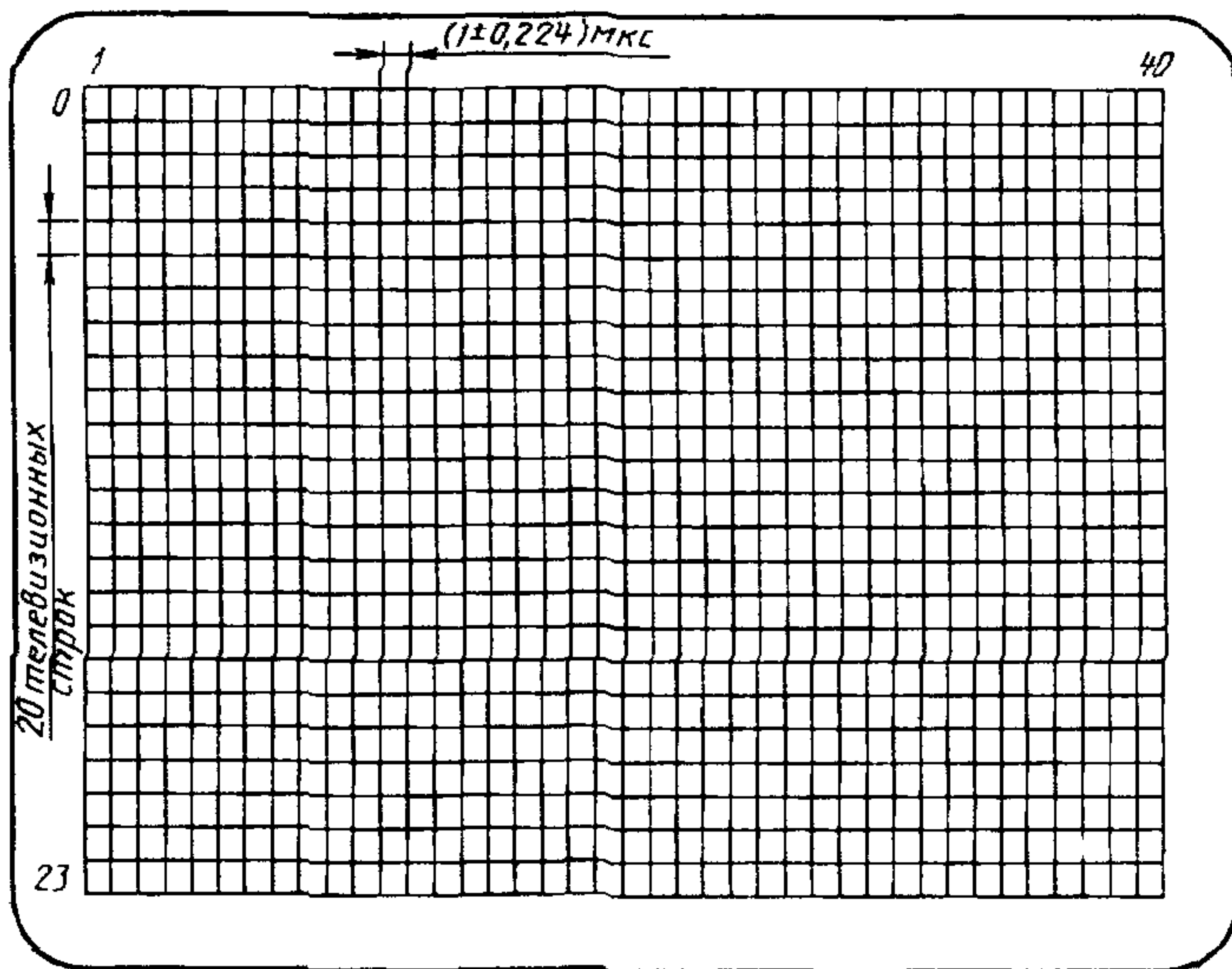
Рисунок 4 — Расположение знакомест на странице телетекста
