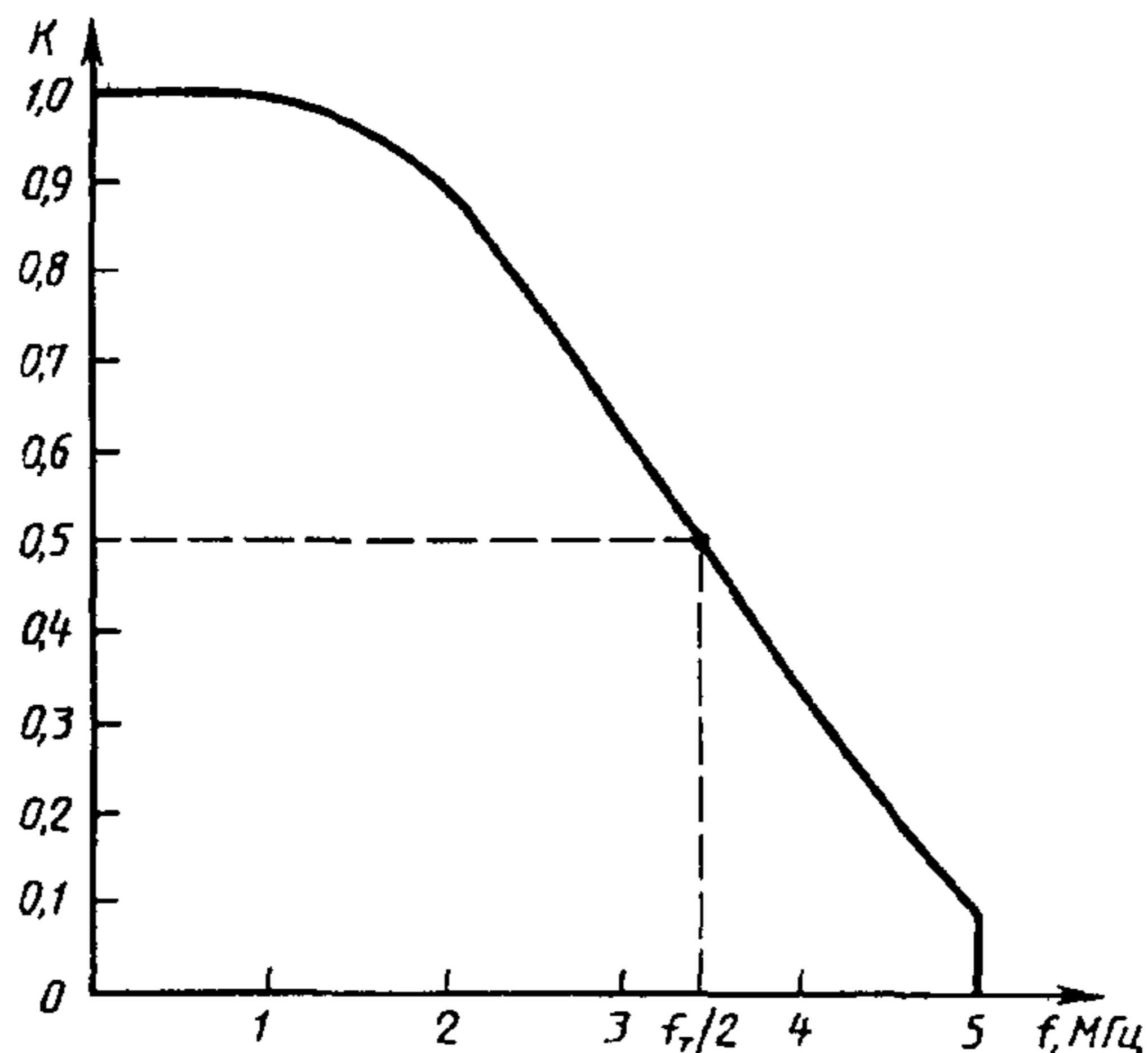
Рисунок 1 — Форма спектра импульсов цифровых данных
