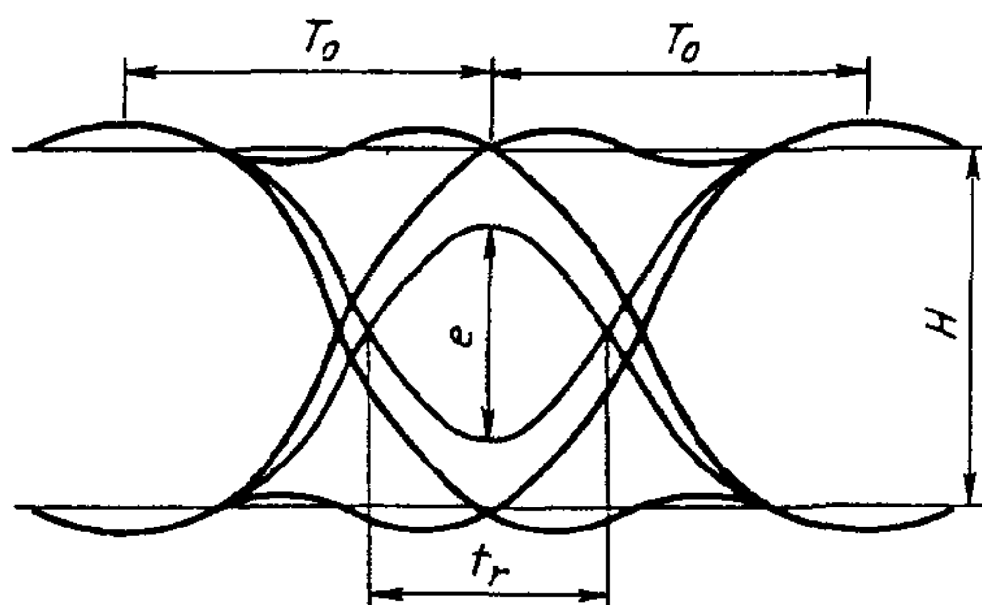
Рисунок 10 — Осциллограмма глазковой диаграммы
