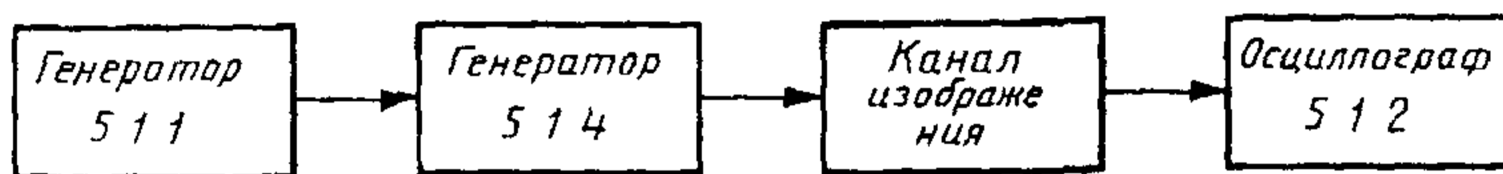
Рисунок 13 — Структурная схема измерений временного положения синхронизации, содержания строки и местоположения пакетов цифровых данных сигнала телетекста
