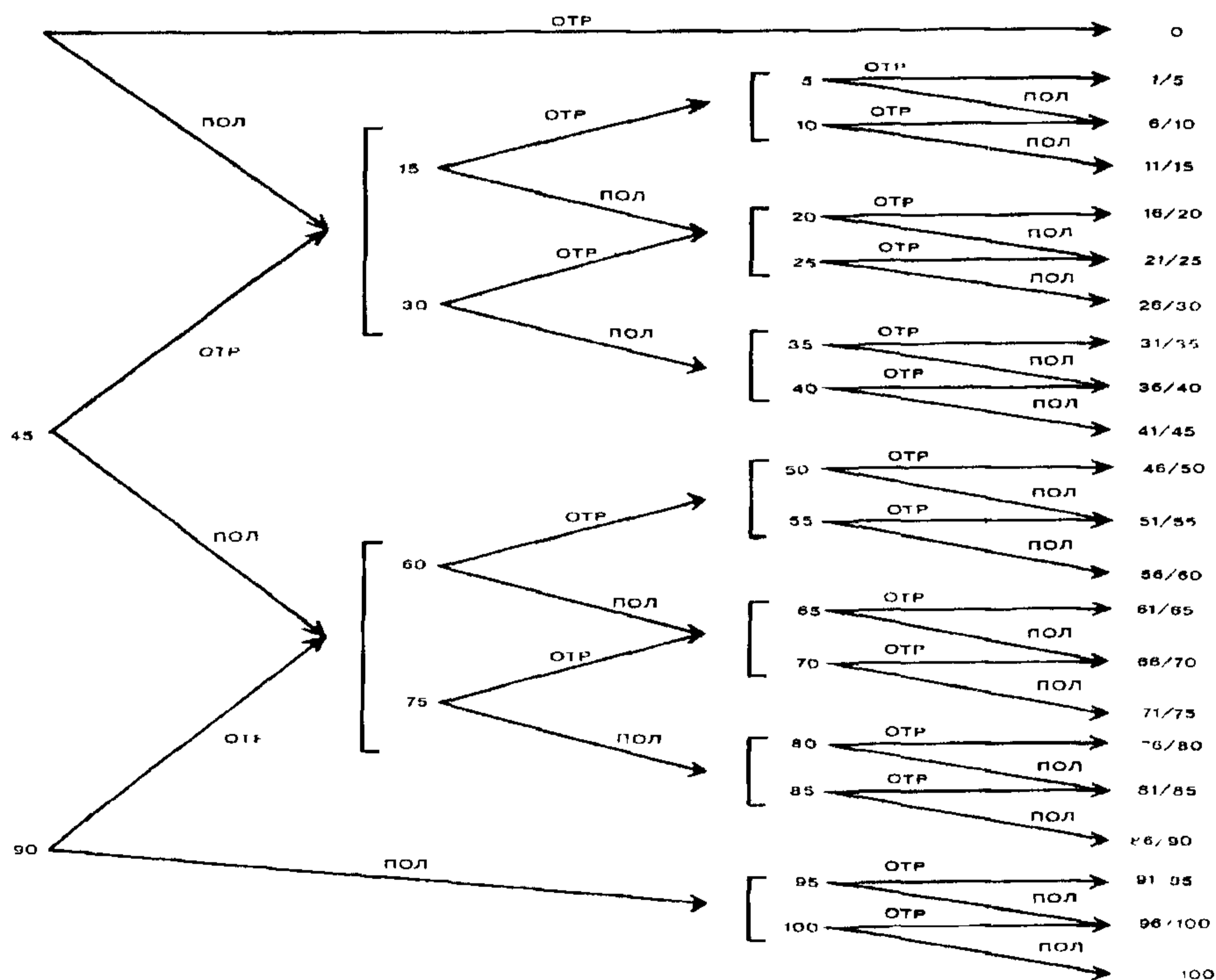
Рисунок 1 — Схема приготовления растворов ксилола в n -гептане
