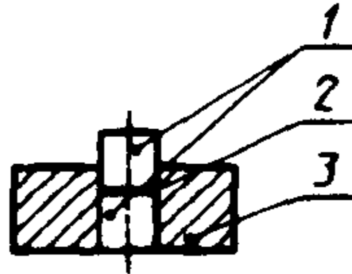
1 — ролик, 2 — навеска БВВ 3 — муфта
